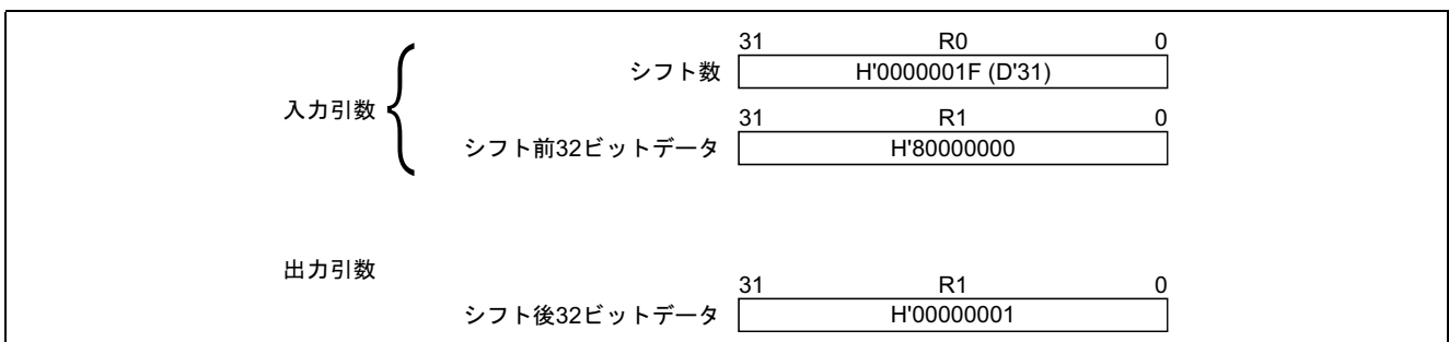
図 1 ソフトウェア SHLRN の実行例
