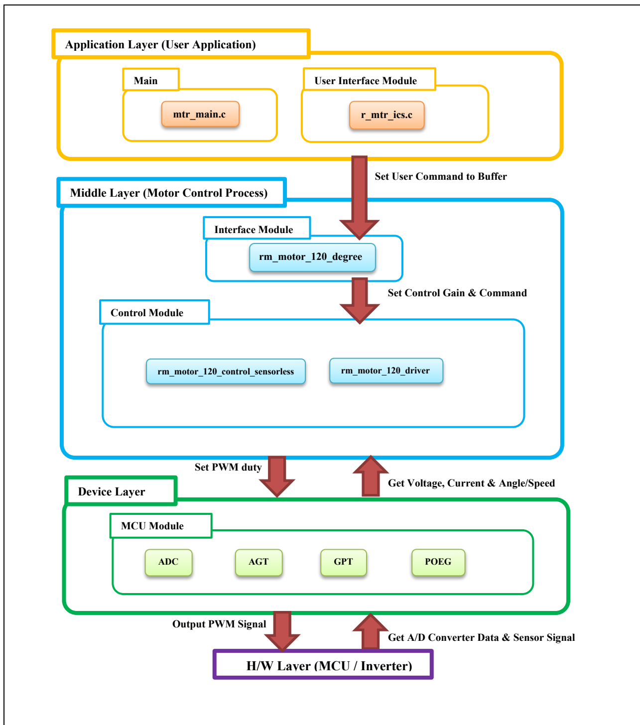
図 2-34 モジュール構成
