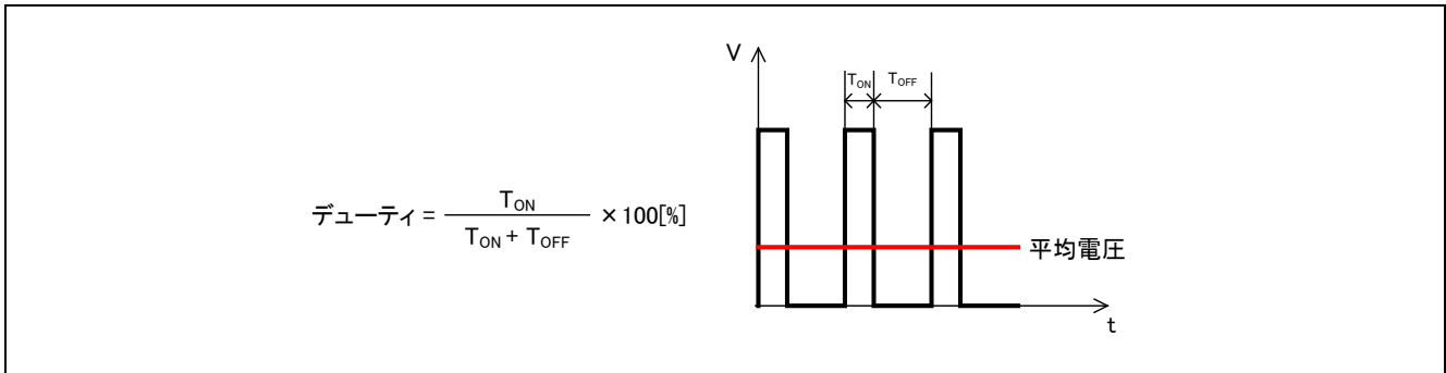
図 3-2 PWM 制御
