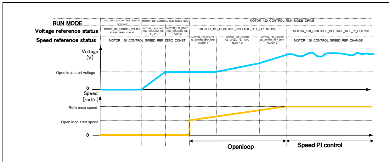
図 3-6 始動方法例
