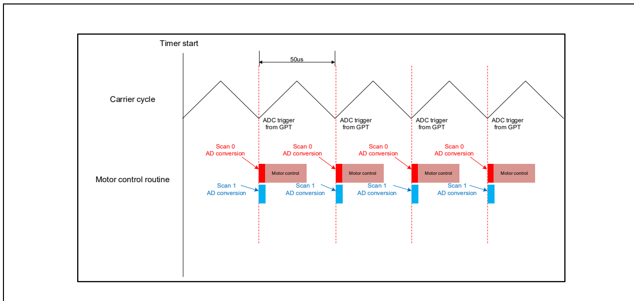
図 3-7 AD トリガタイミング
