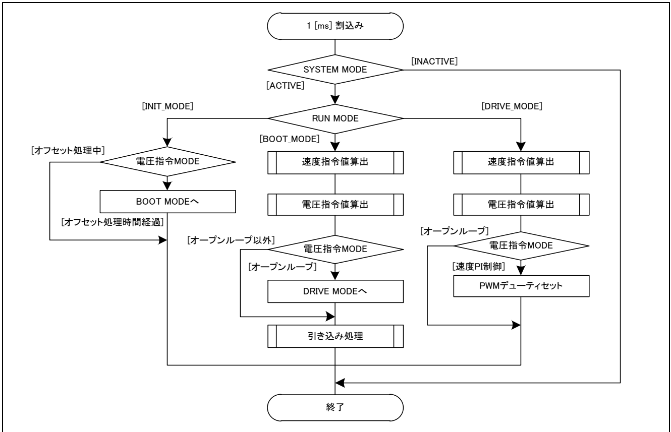
図 3-10 速度制御周期割り込み処理フローチャート
