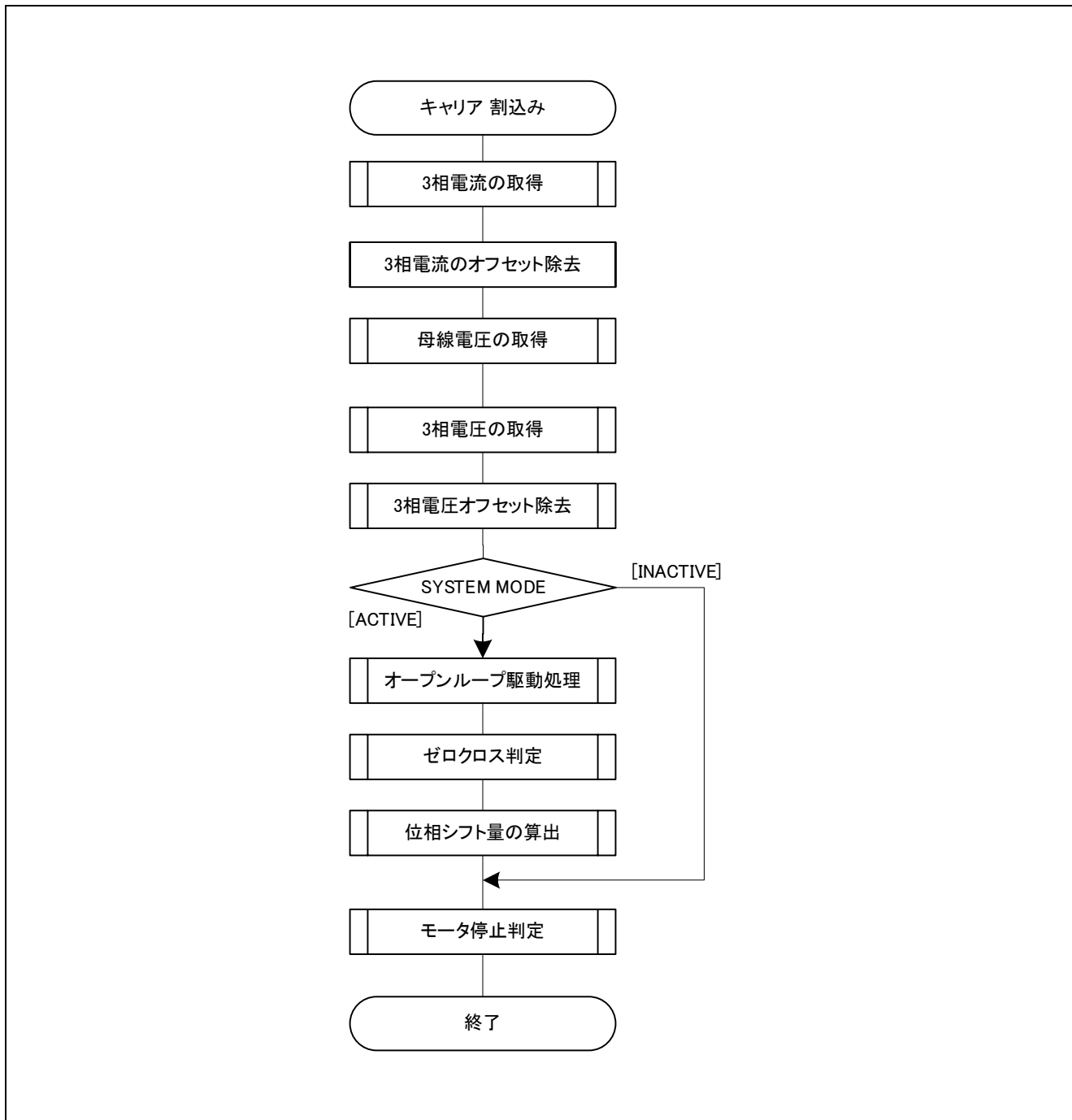
図 3-9 電流制御周期割り込み処理フローチャート
