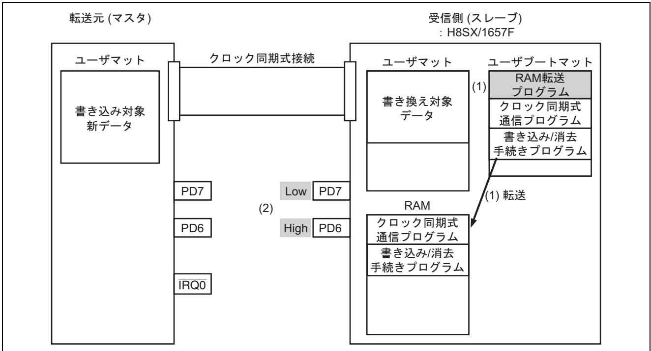
図 6 オンボード書き換え開始
