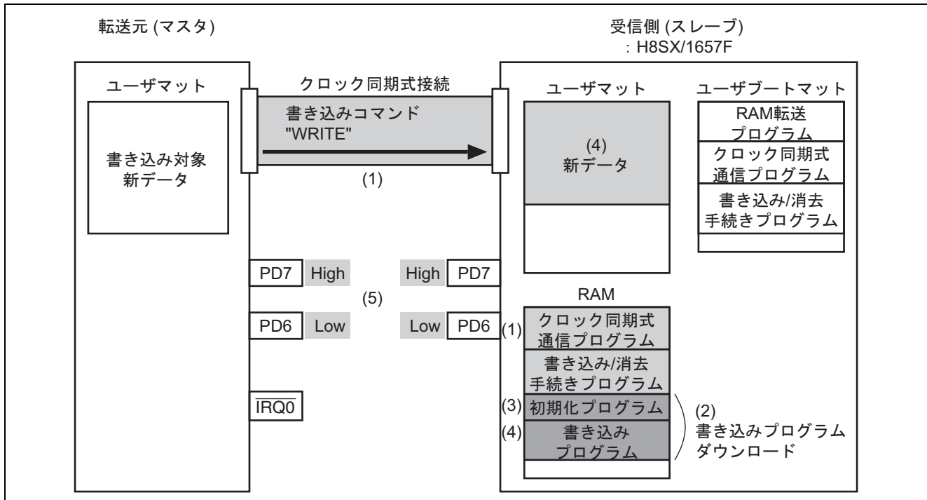
図9 ユーザマット書き込み
