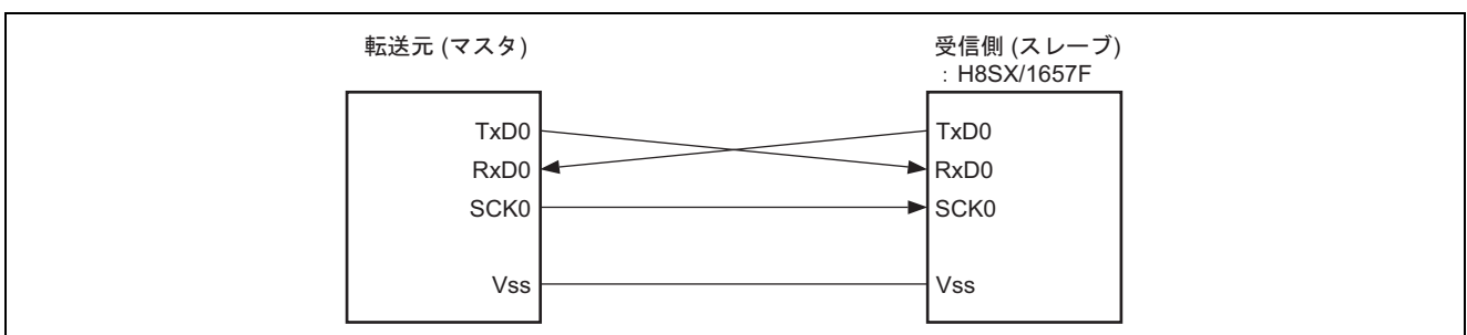
図 2 クロック同期式通信接続図
