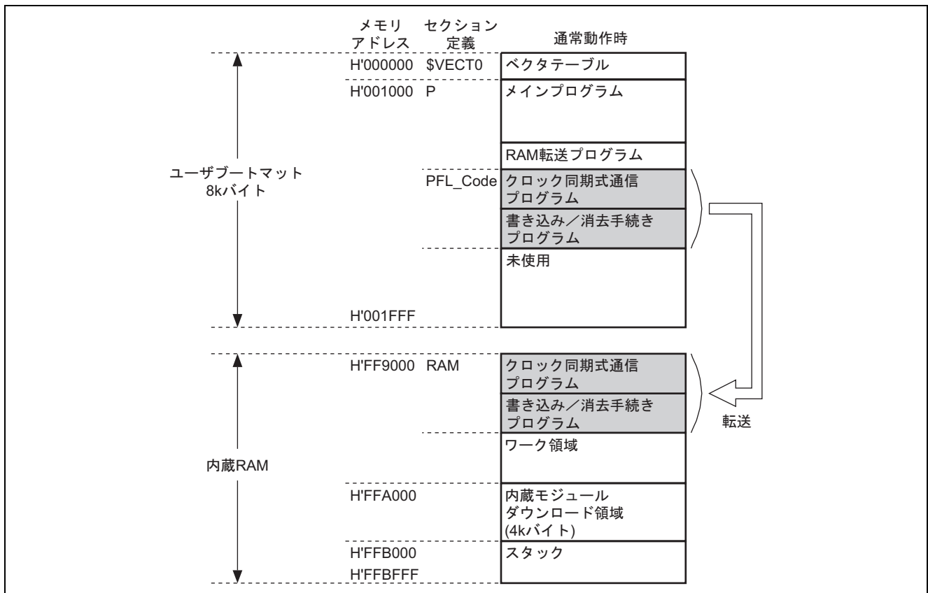
図3 メモリマップ
