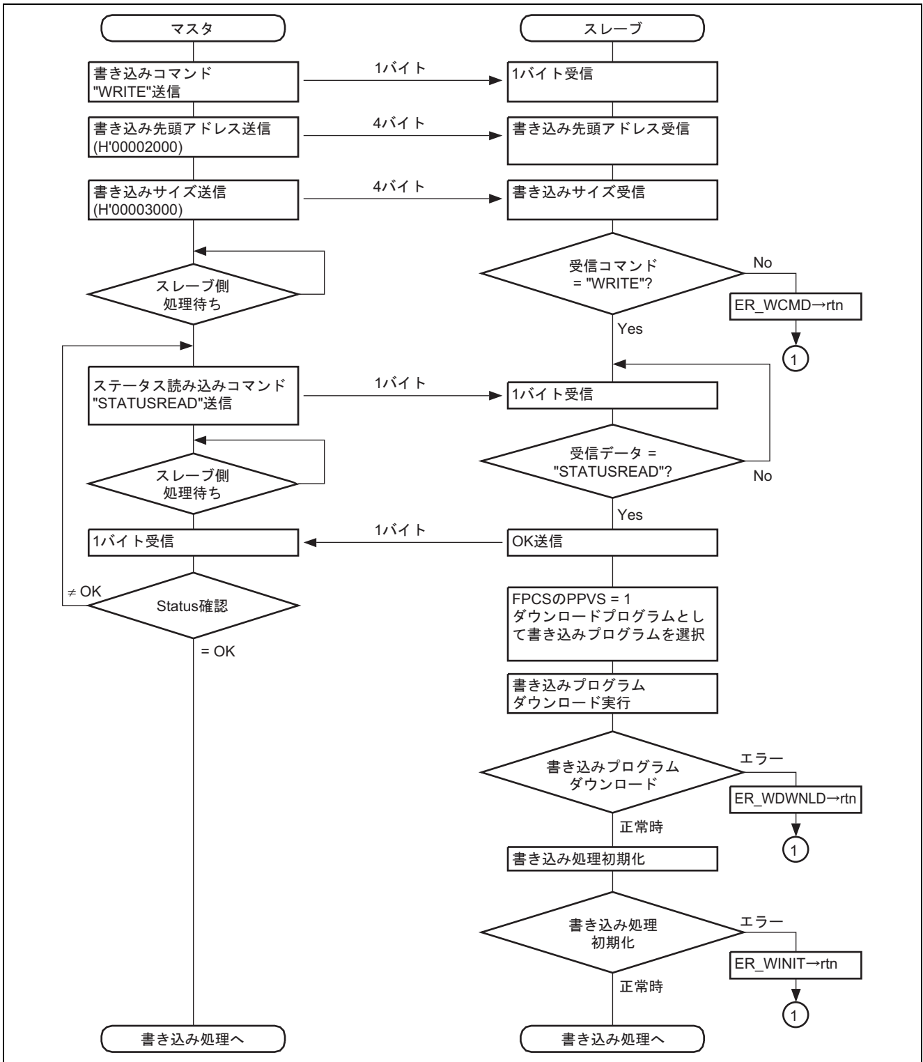
図 11 書き込み位置・サイズ受信処理
