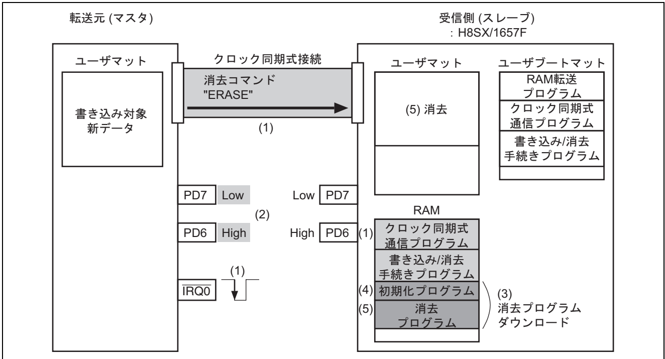
図 8 ユーザマット消去
