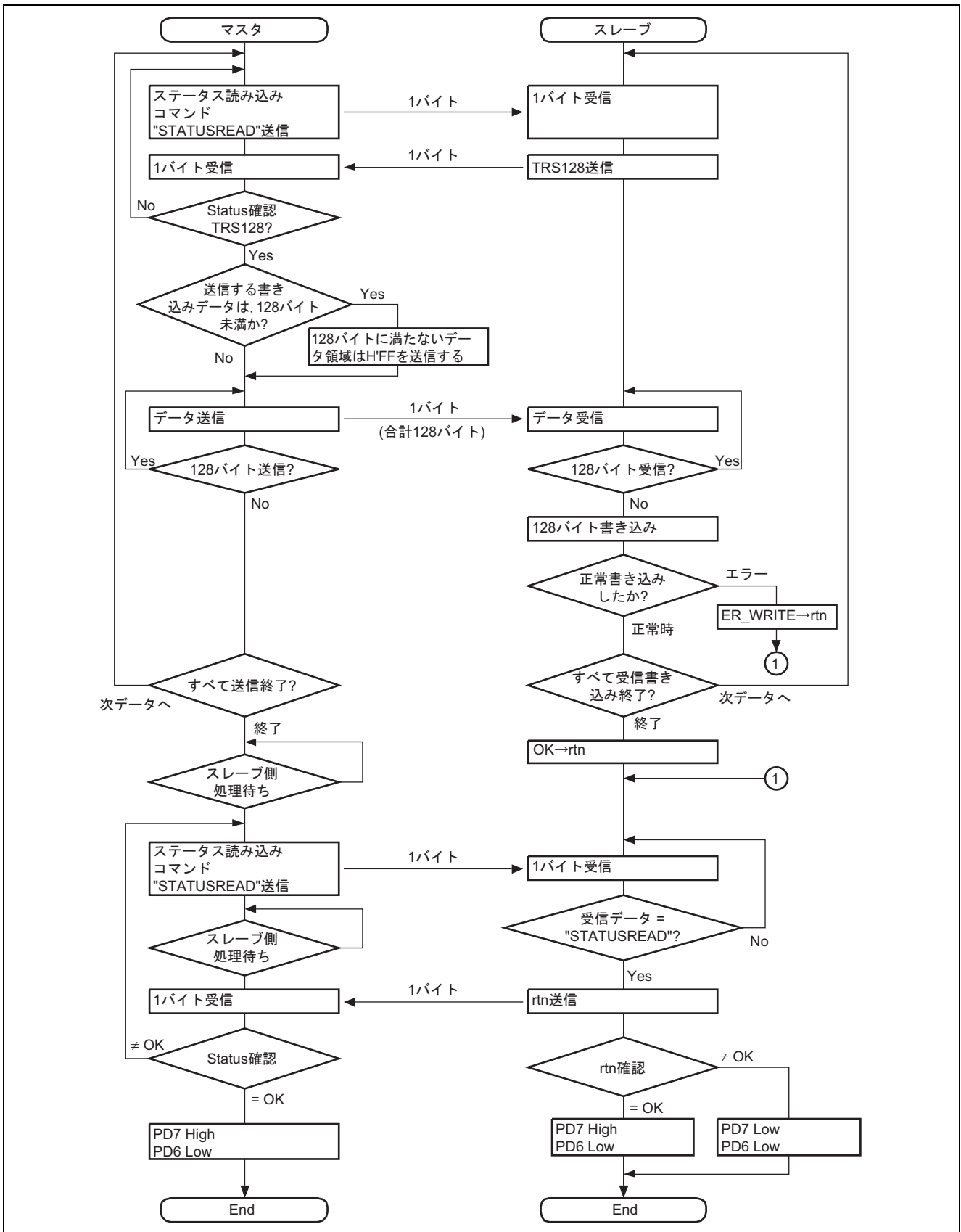
図 12 書き込み処理
