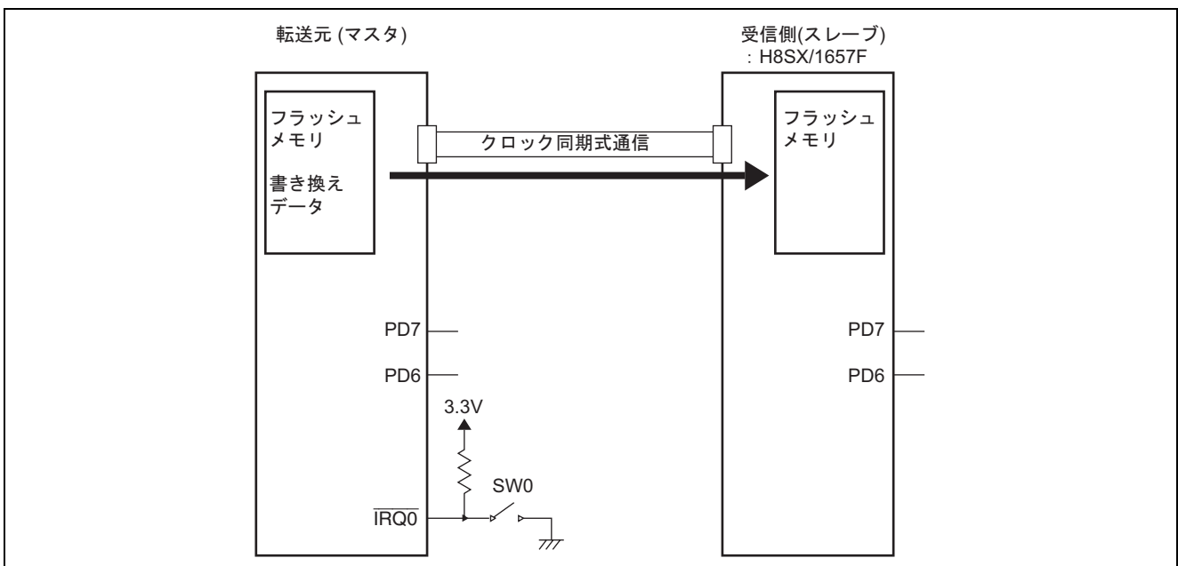
図 1 オンボード書き換え構成例
