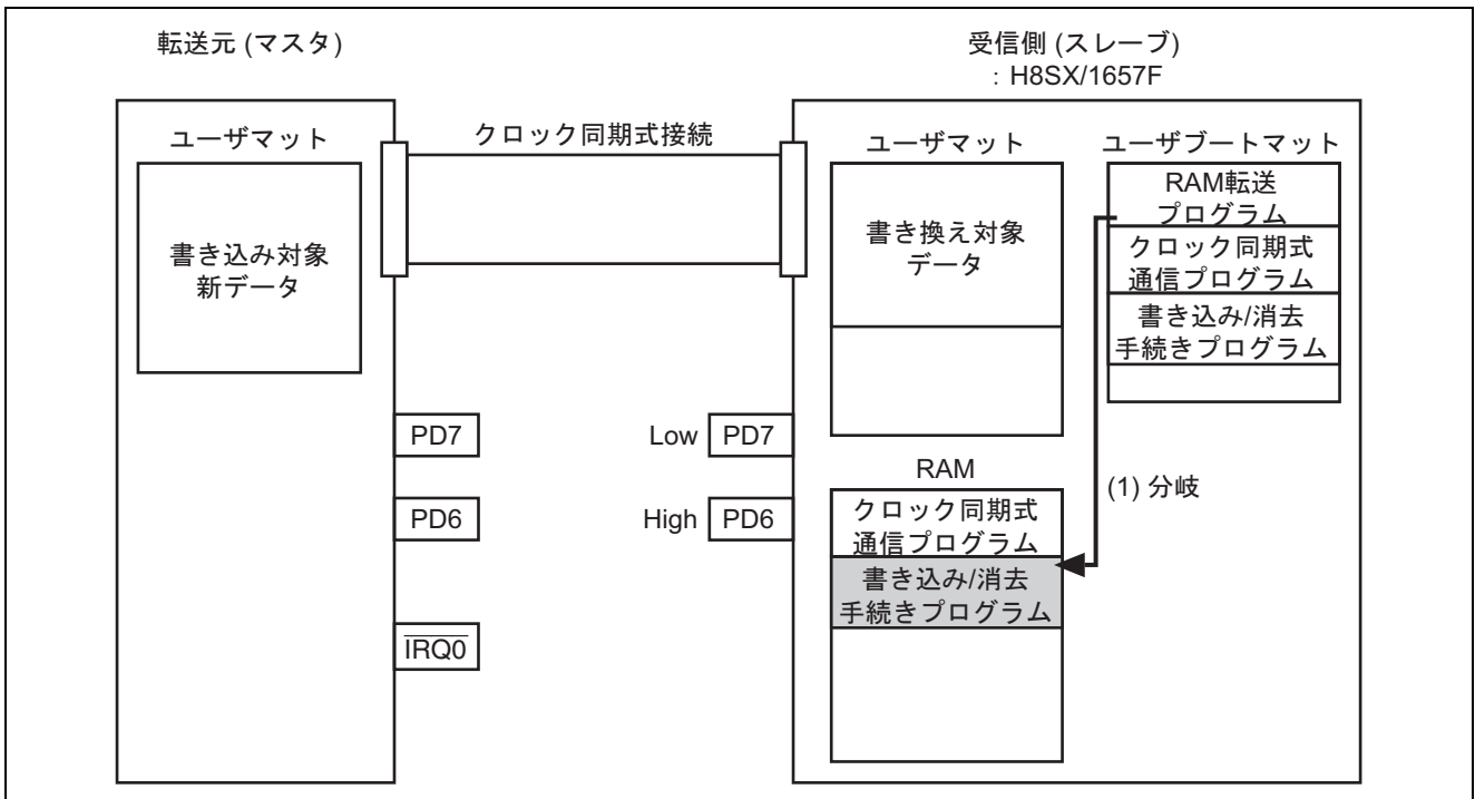
図 7 書き込み / 消去手続きプログラム起動
