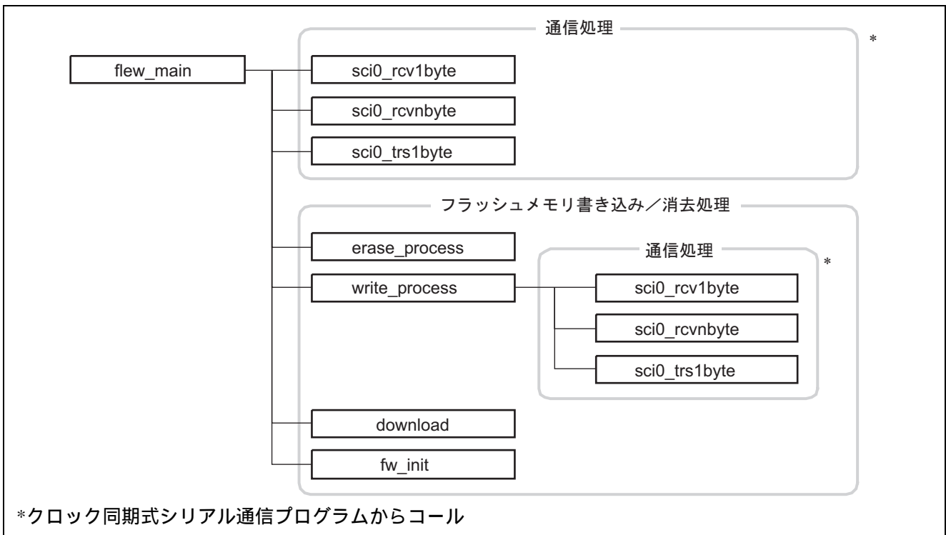
図 14 書き込み / 消去手続きプログラム
