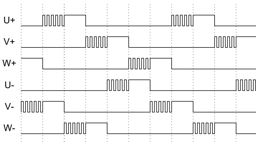
図 3-3 非相補前半 60 度チョッピング
