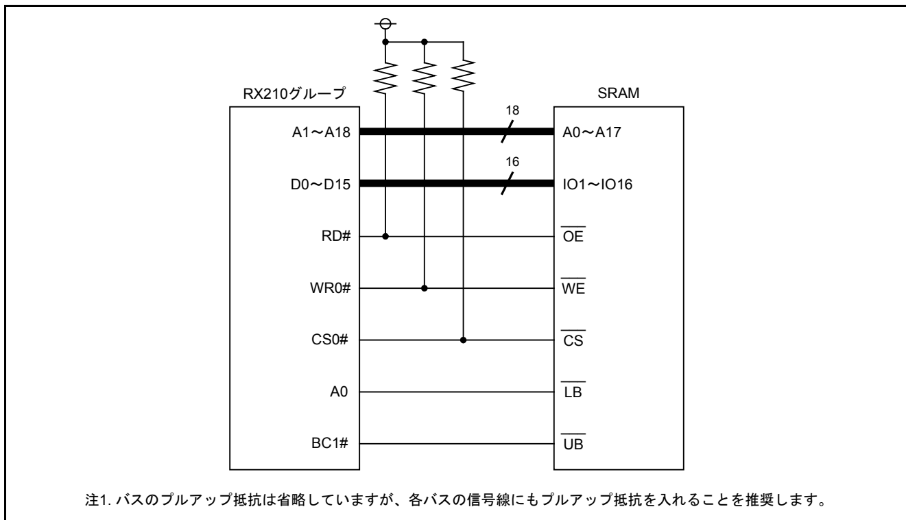
図2.2 セパレートバス 16 ビットでの接続図
