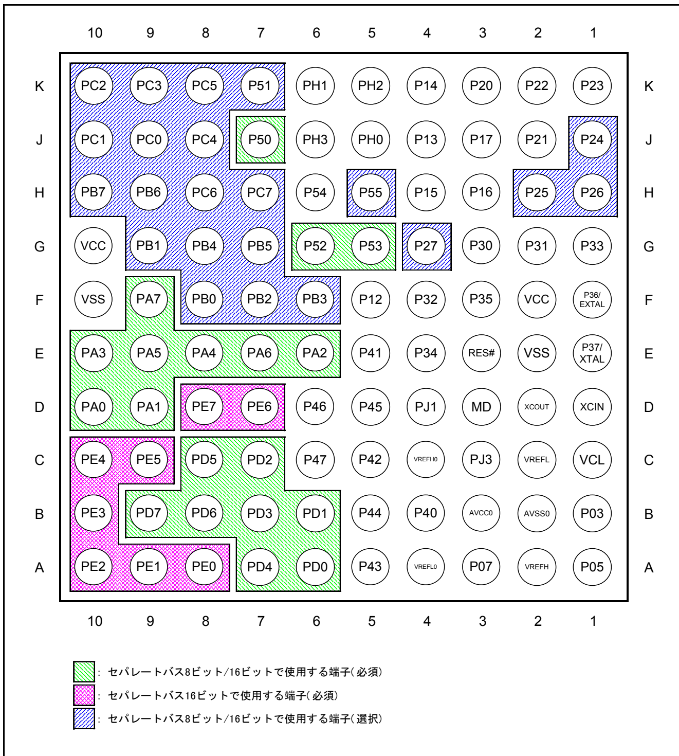
図1.2 セパレートバスの端子配置図(TFLGA パッケージ)
