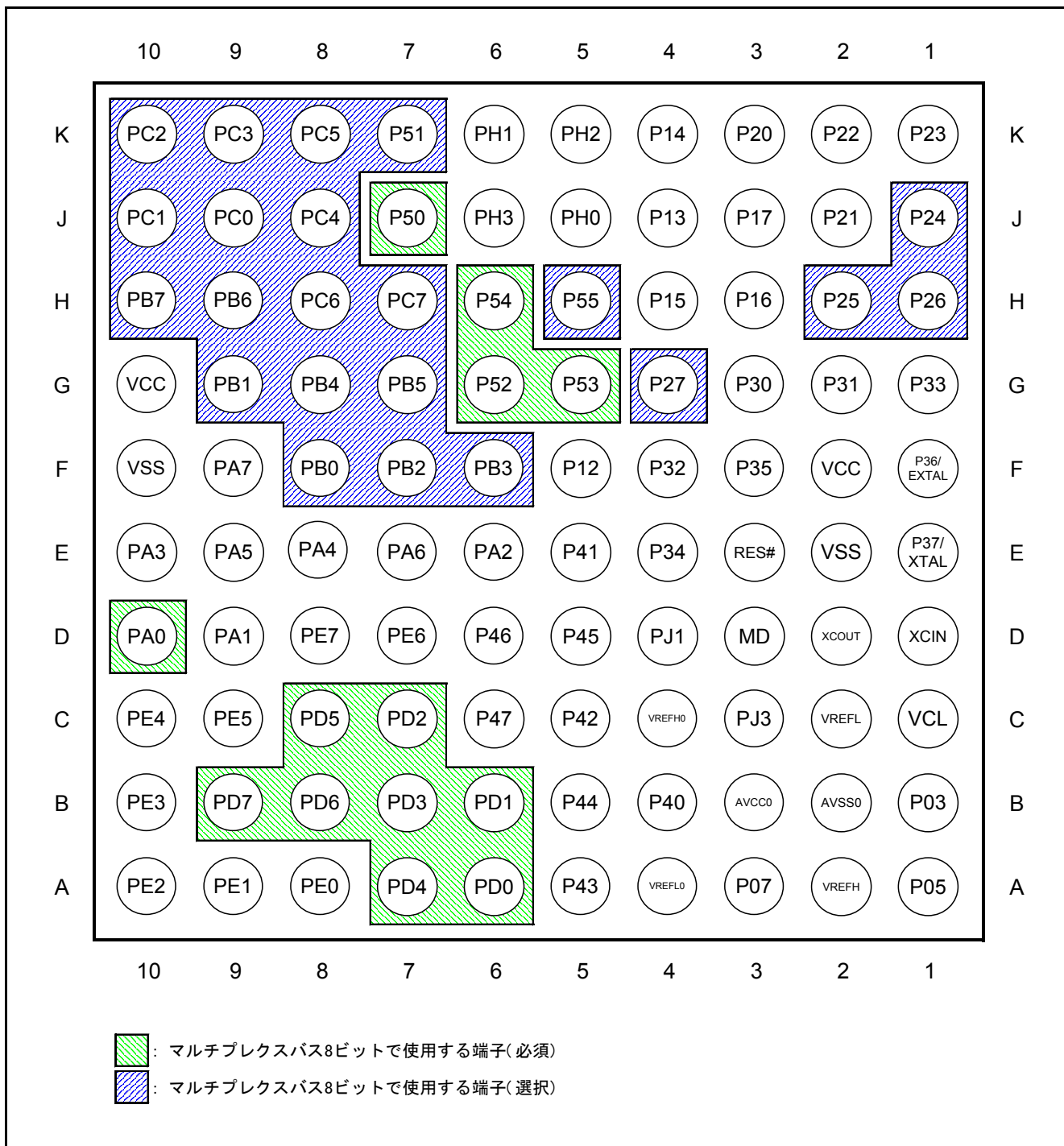
図1.3 マルチプレクスバスの端子配置図(TFLGA パッケージ)
