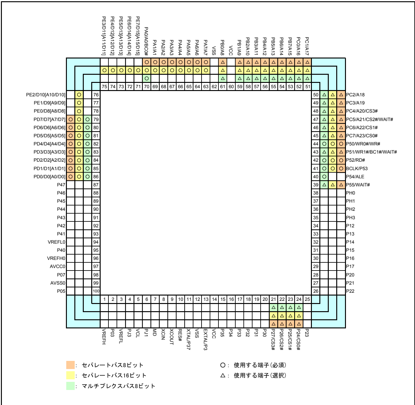
図1.1 端子配置図(LQFP パッケージ)
