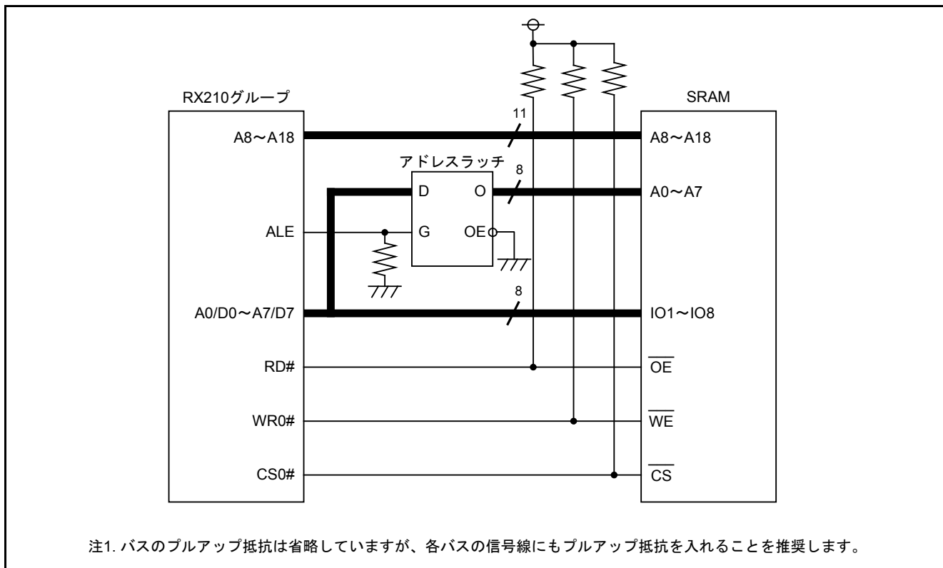
図2.3 マルチプレクスバス 8 ビットでの接続図
