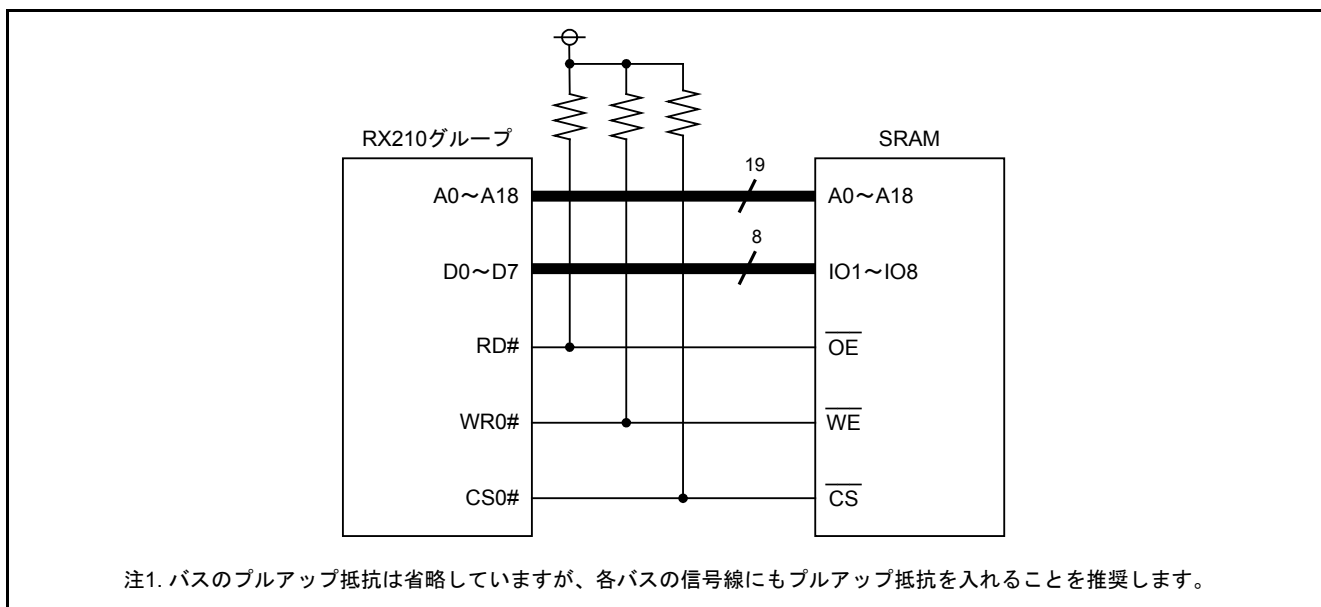
図2.1 セパレートバス 8 ビットでの接続図
