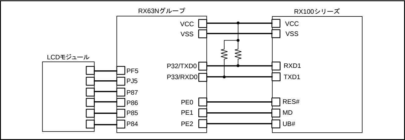
図4.1 接続例
