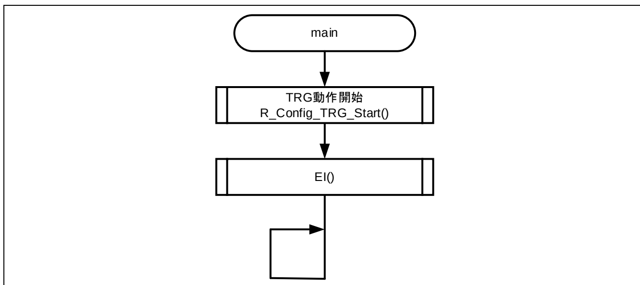
図 4-5 メイン処理
