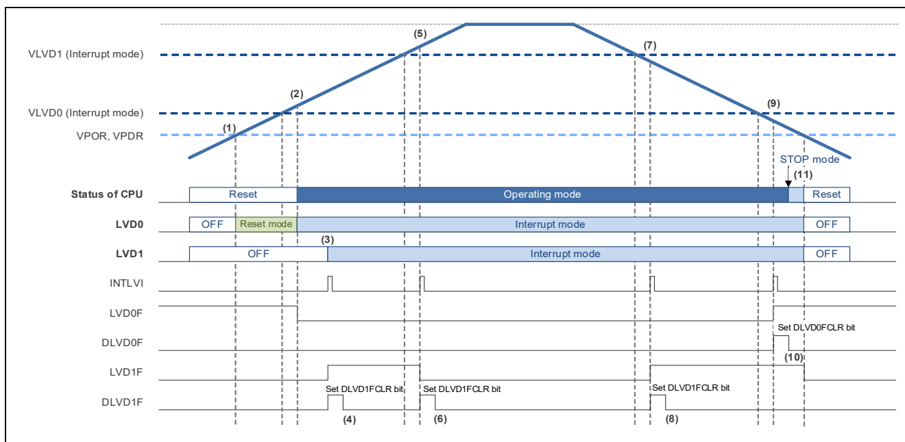
図 3-1 LVD0: 割り込みモード、LVD1: 割り込みモード、 V_{LVD0} < V_{LVD1} 設定時の動作
