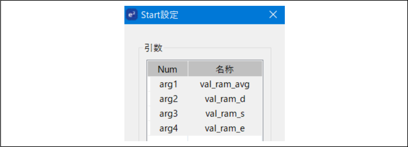
図 6-2 Start 設定
