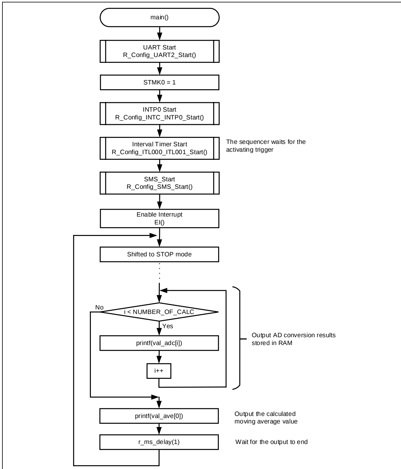
図 5-1 メイン処理
