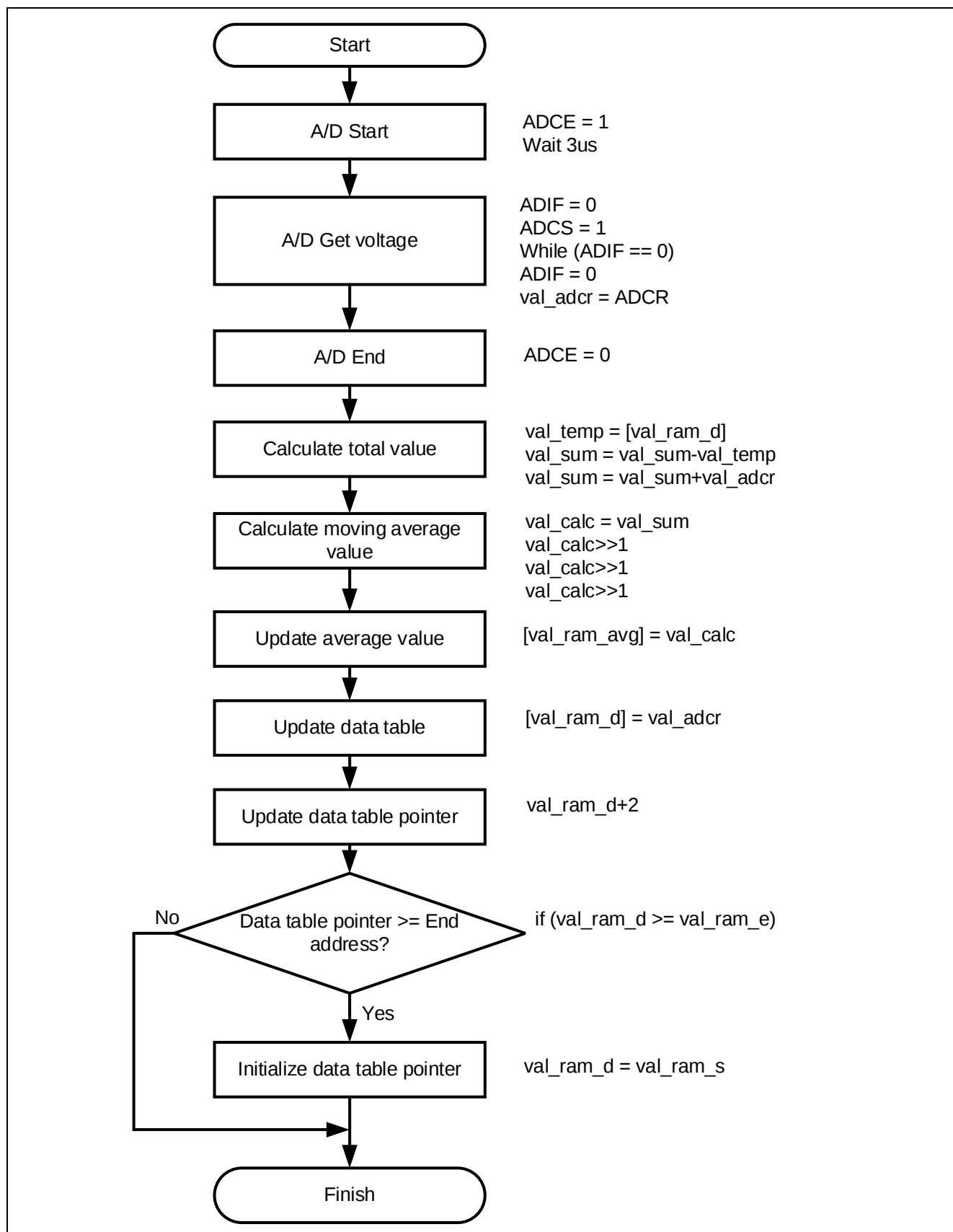
図 5-7 SMS 処理
