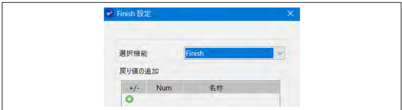
図 6-14 Finish 設定
