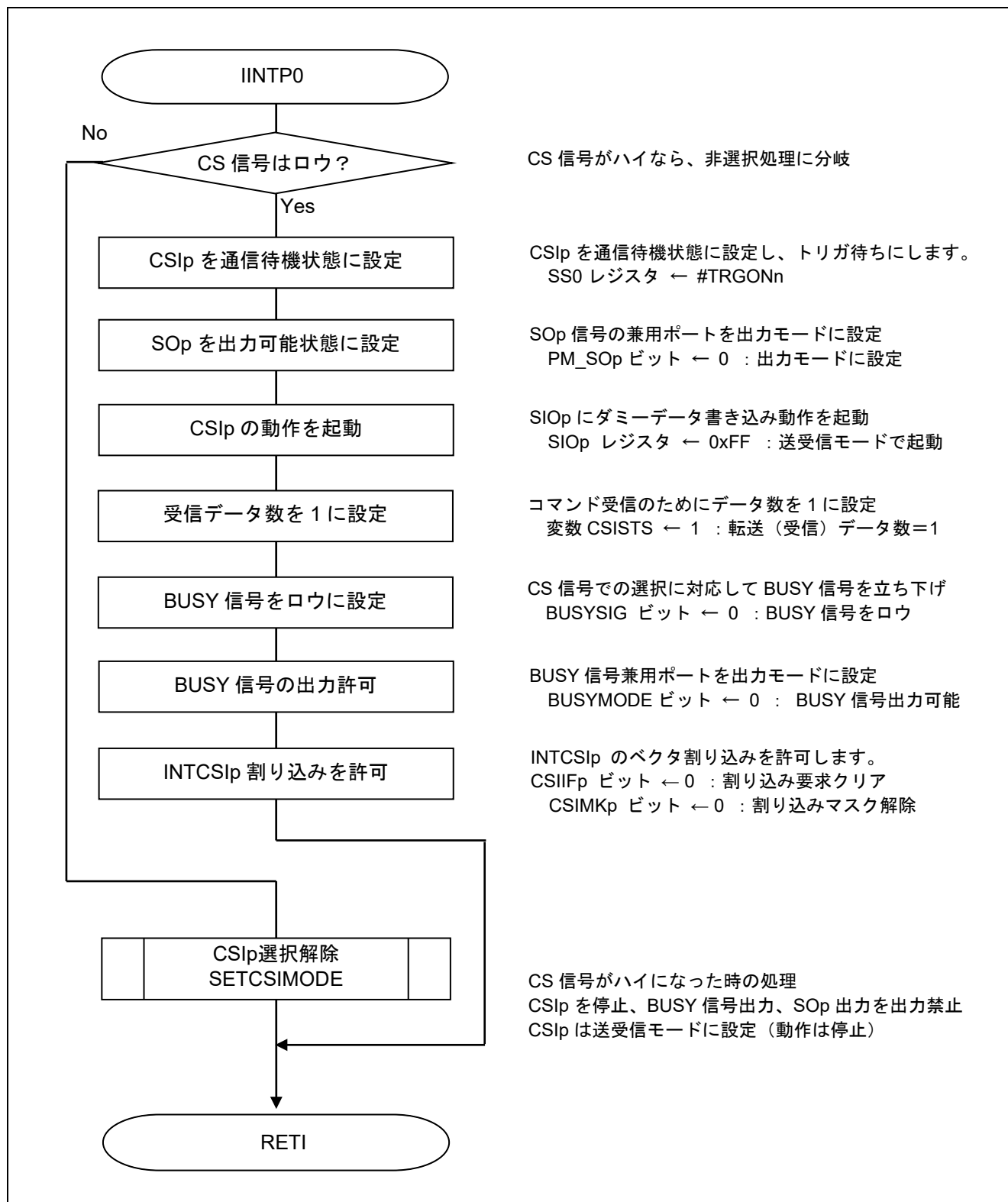
図 5.15 INTPO 割り込み処理関数
