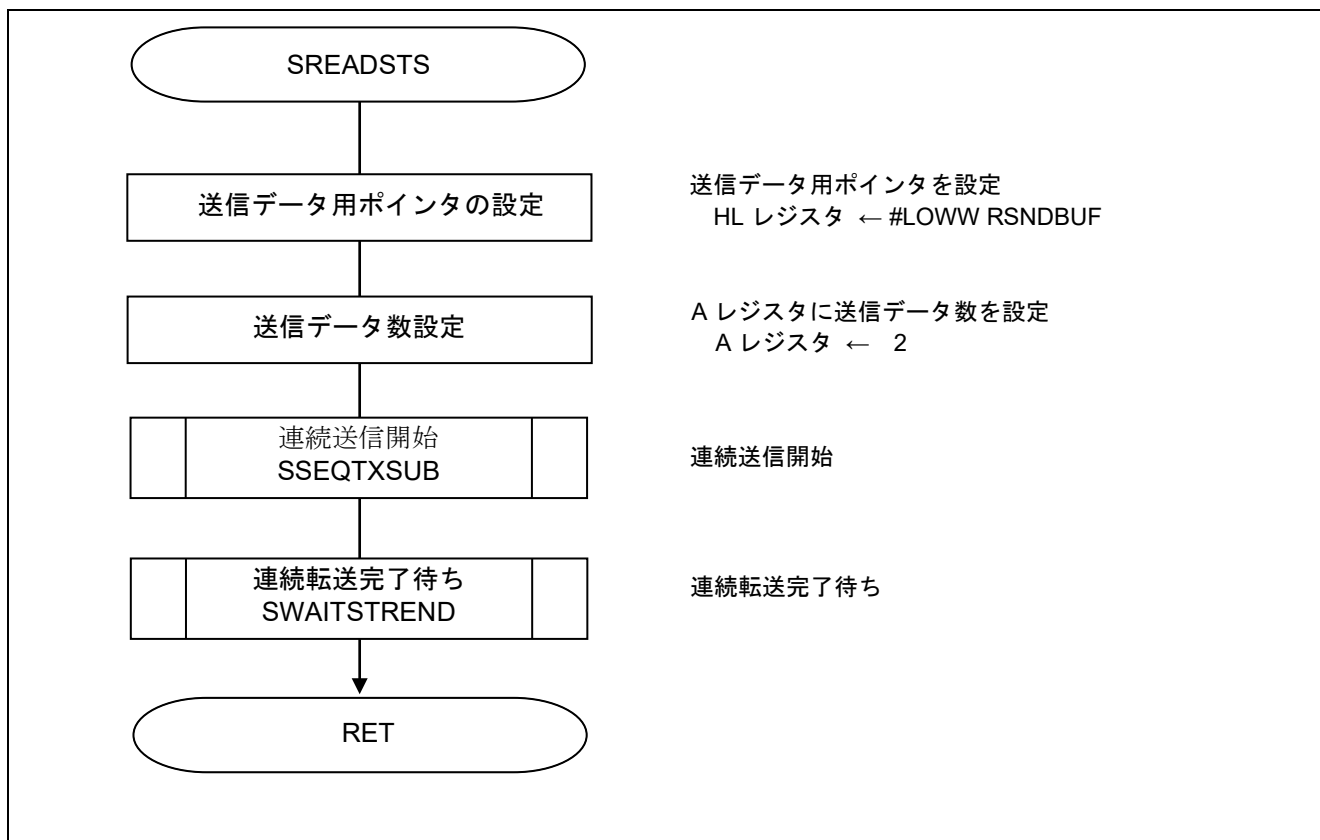
図 5.10 ステータス確認コマンド処理関数
