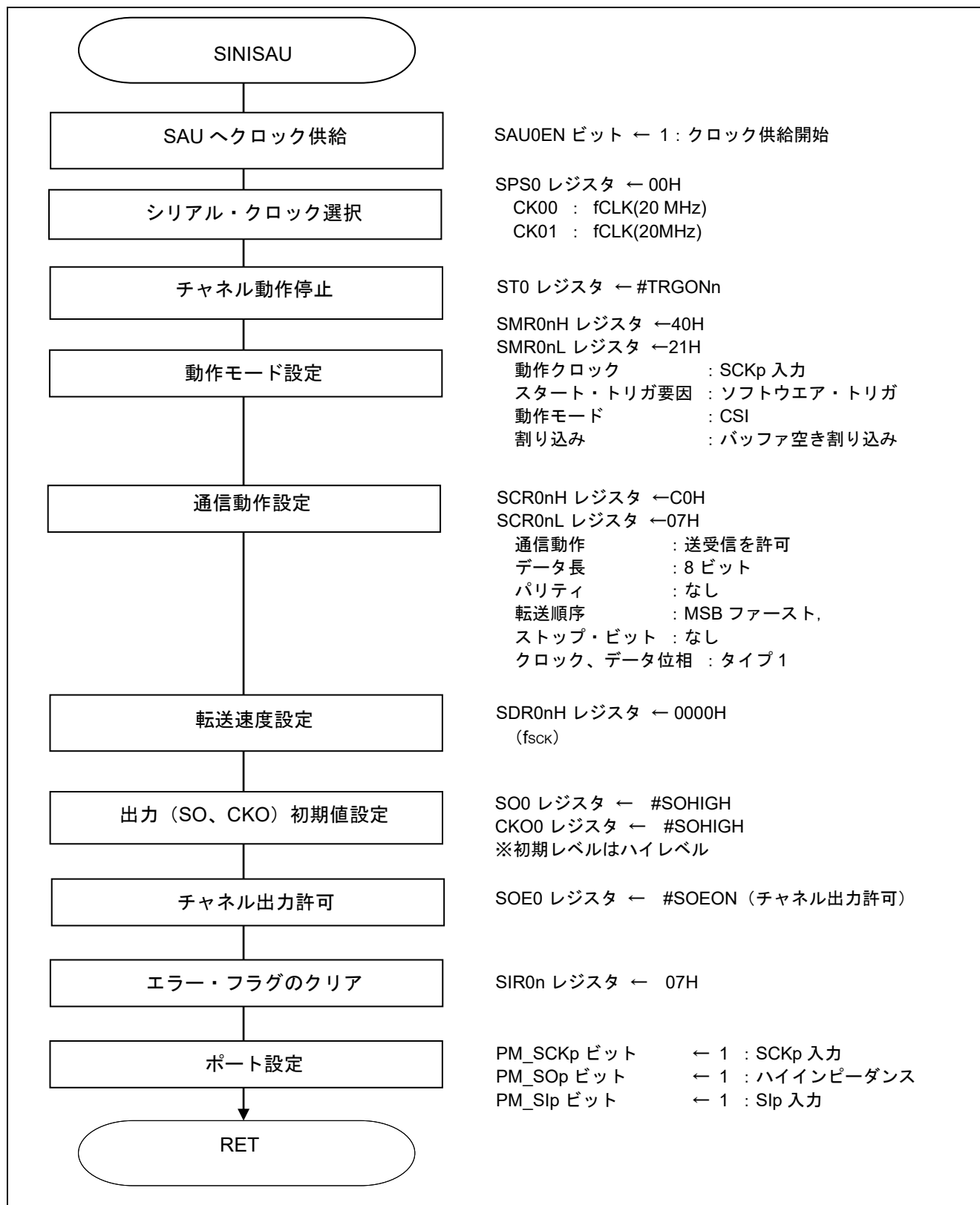
図 5.5 SAU の設定
