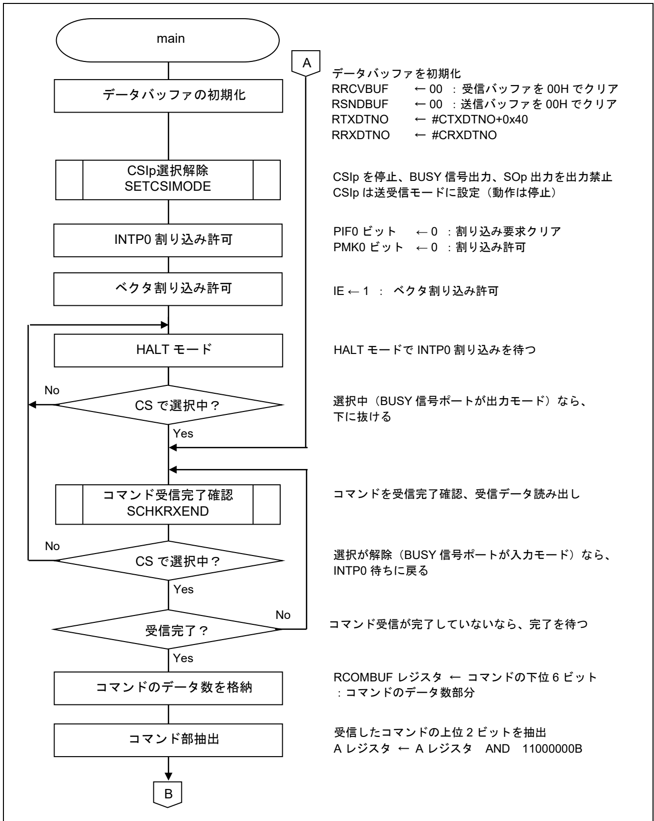
図 5.7 メイン処理(1/2)
