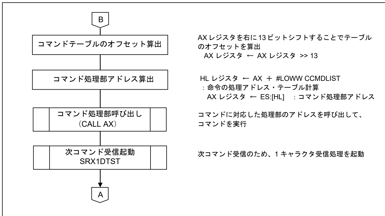
図 5.8 メイン処理(2/2)
