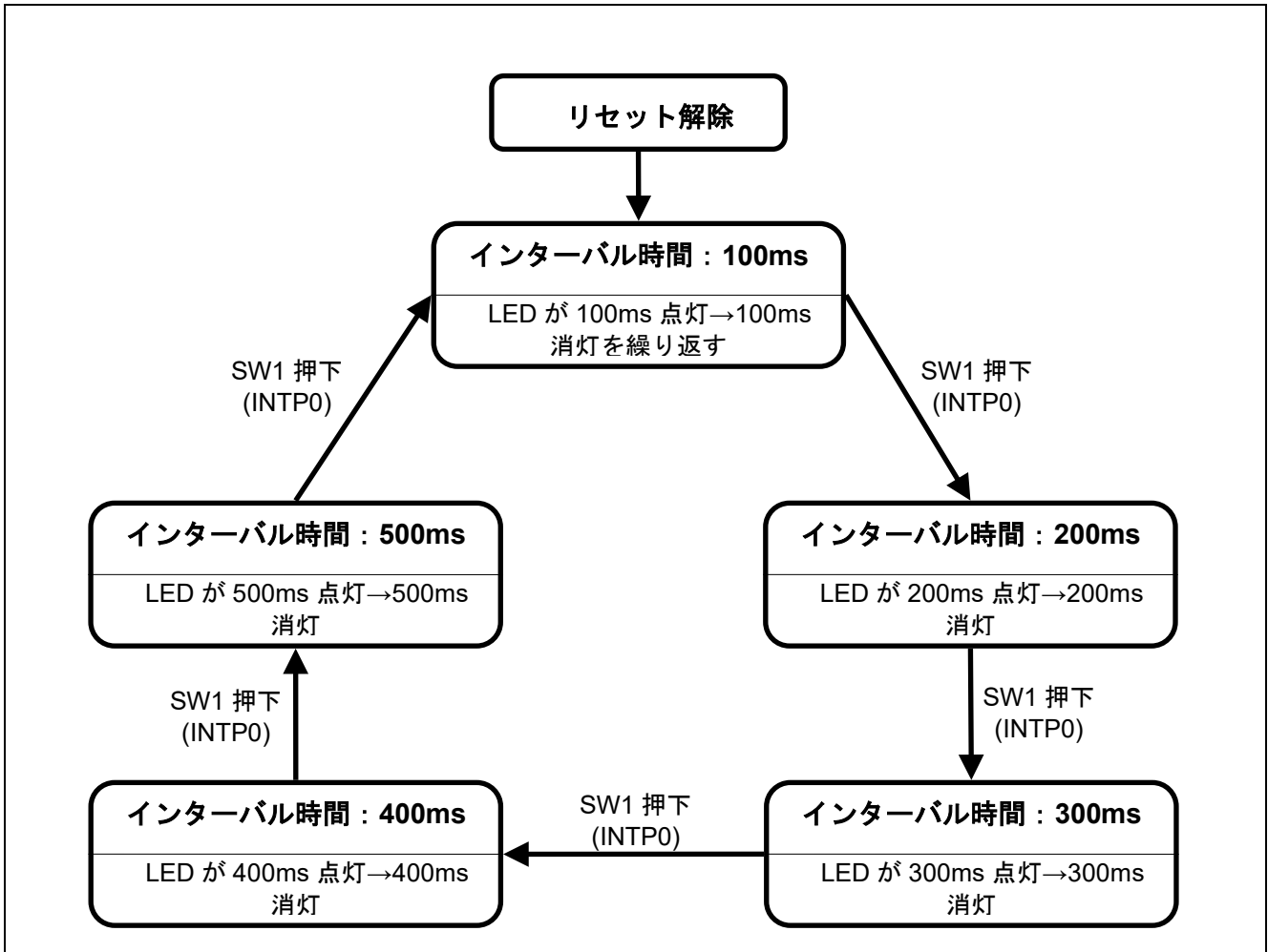
図 1.1 動作概要
