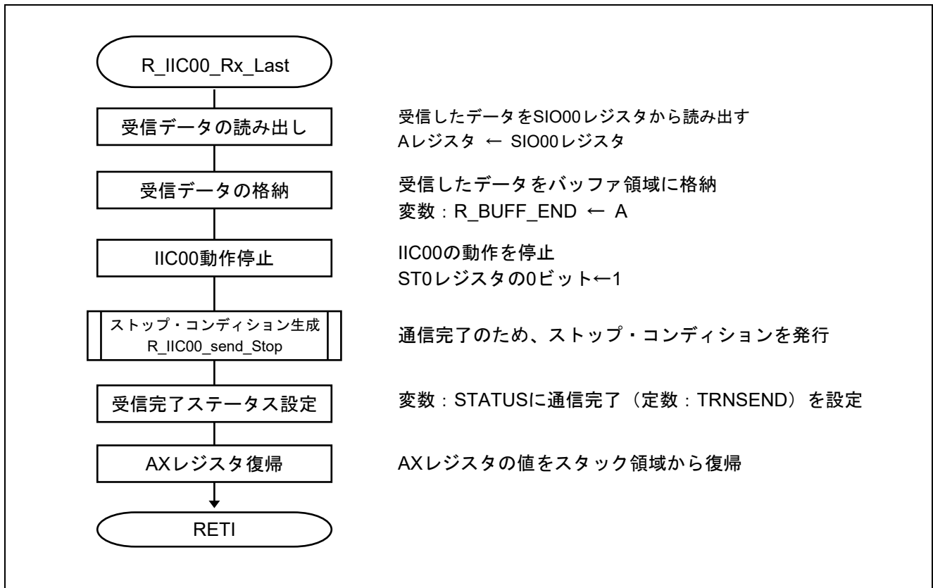
図 5.22 最終データ受信処理
