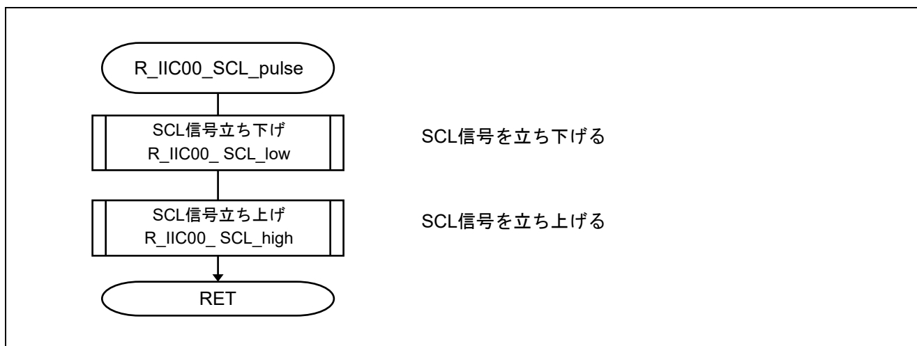
図 5.37 SCL パルス発生
