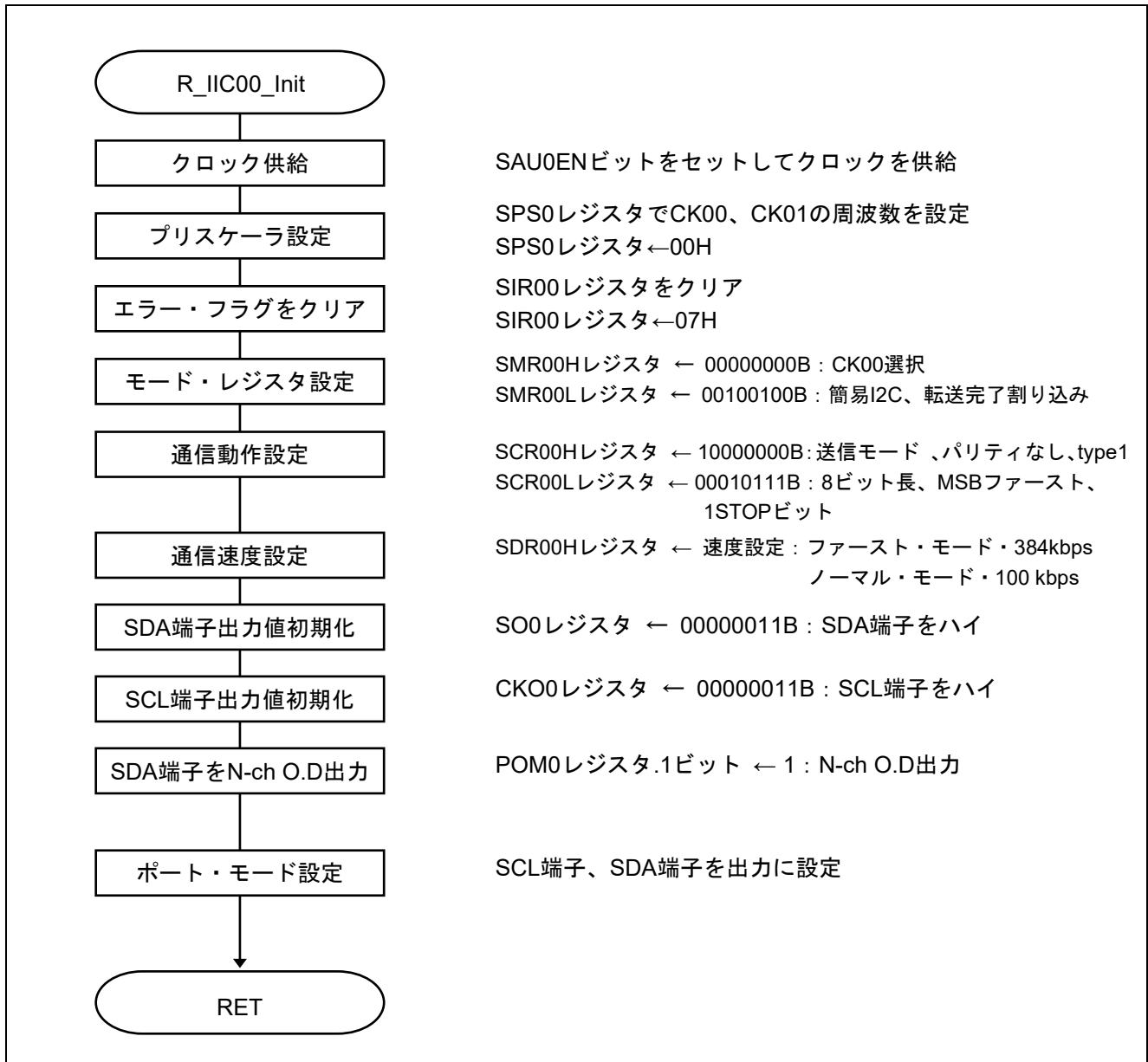
図 5.14 IIC 初期設定
