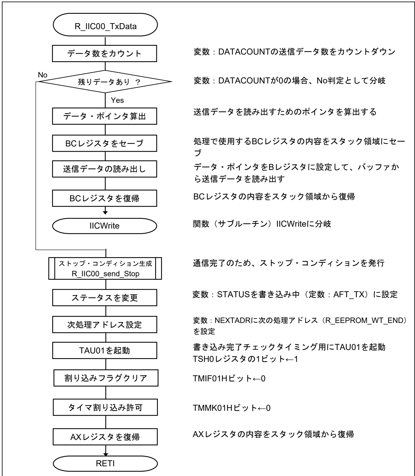
図 5.24 データ送信処理
