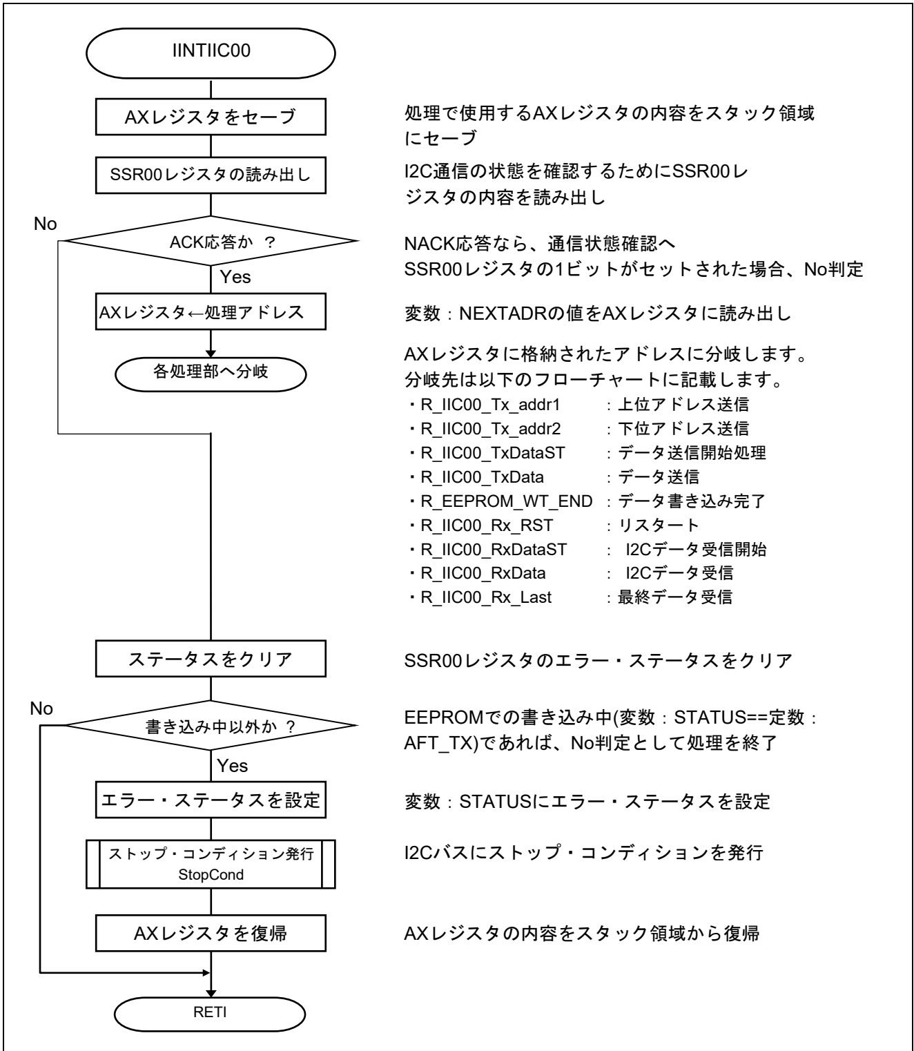
図 5.15 INTIIC00 割り込みエントリ処理
