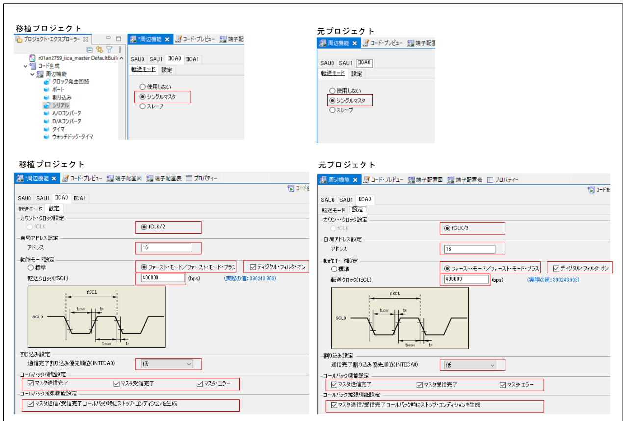
図 3-27 シリアル—IICA0（移植例 2）
