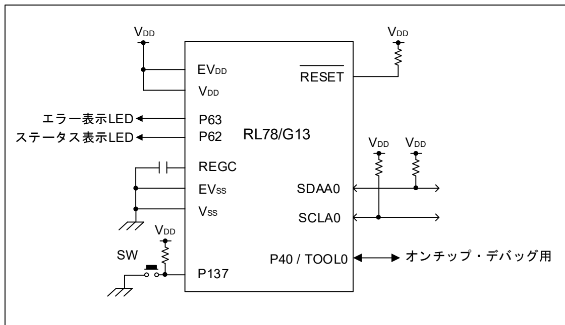
図 3-17 ハードウェア構成例（移植例 2）
