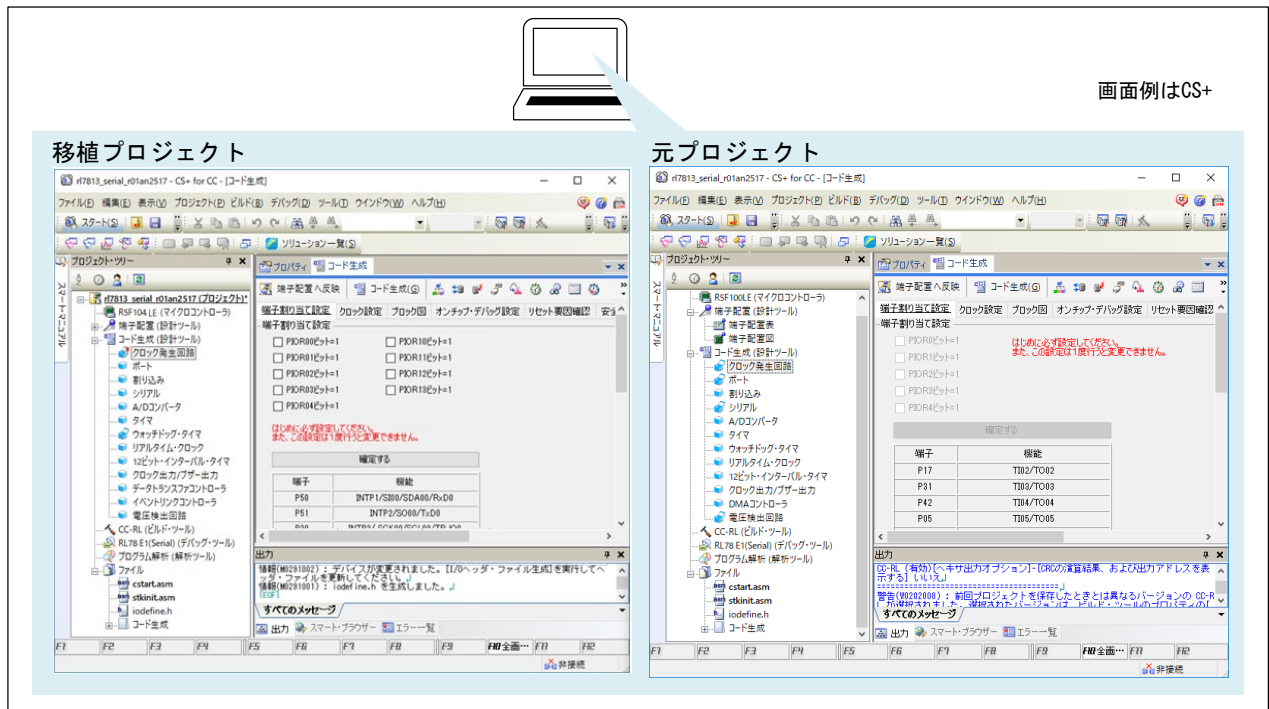
図 2-21 CG 設定作業のイメージ画面
