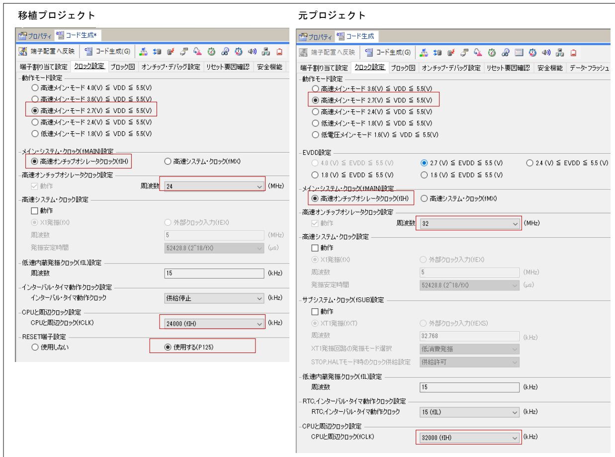
図 3-3 クロック設定（移植例 1）
