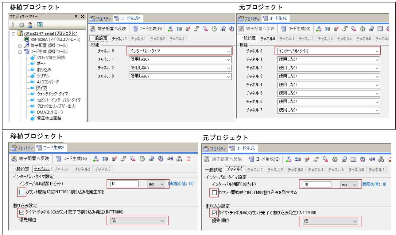
図 3-12 タイマーチャンネル 0 (移植例 1)
