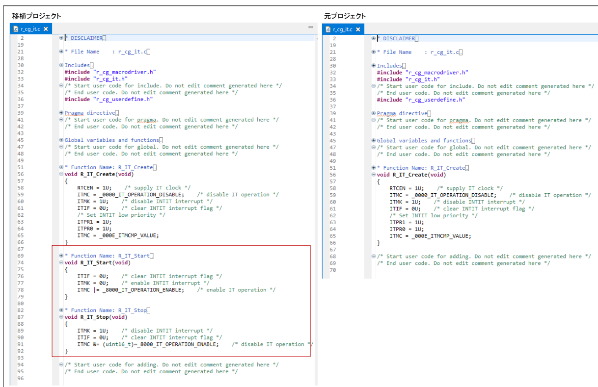
図 3-37 r_cg_it.c (移植例 2)
