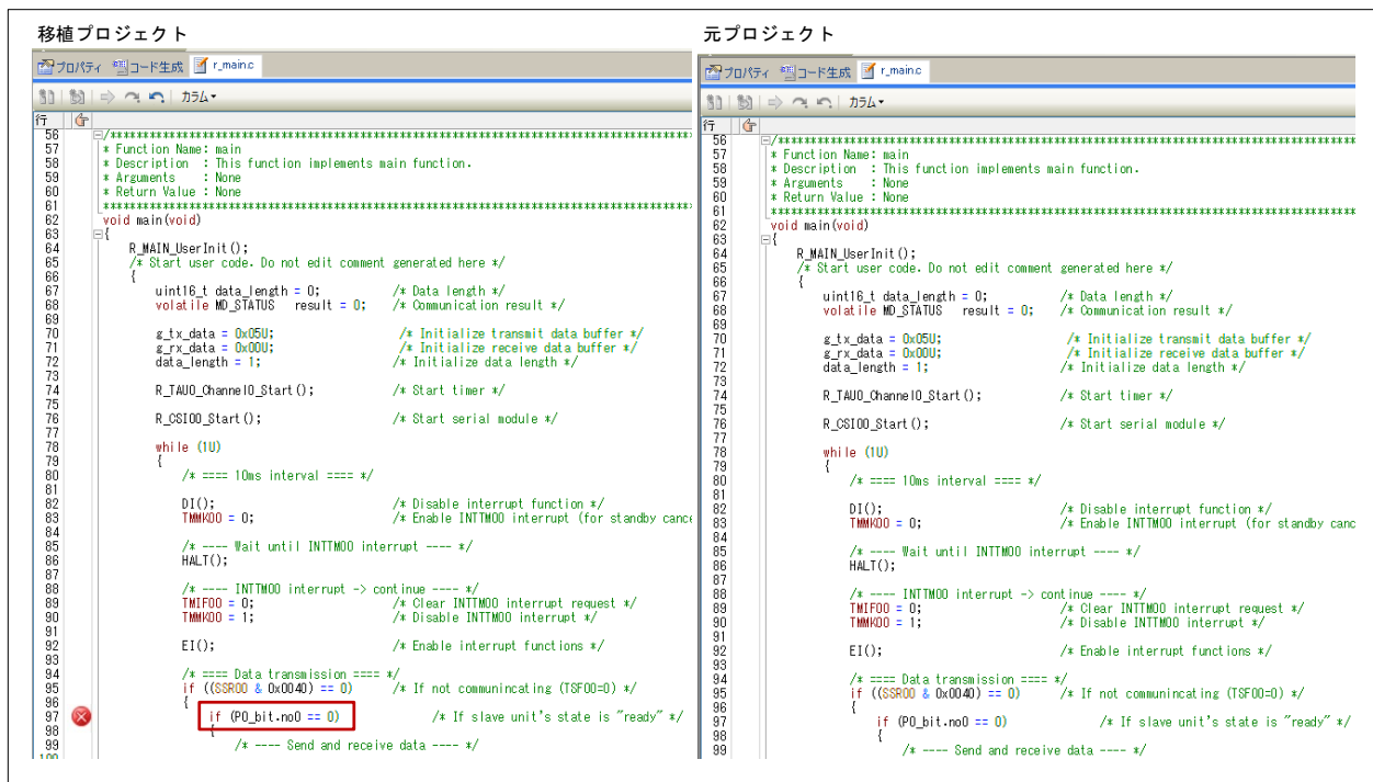
図 3-16 r_main.c (移植例 1)
