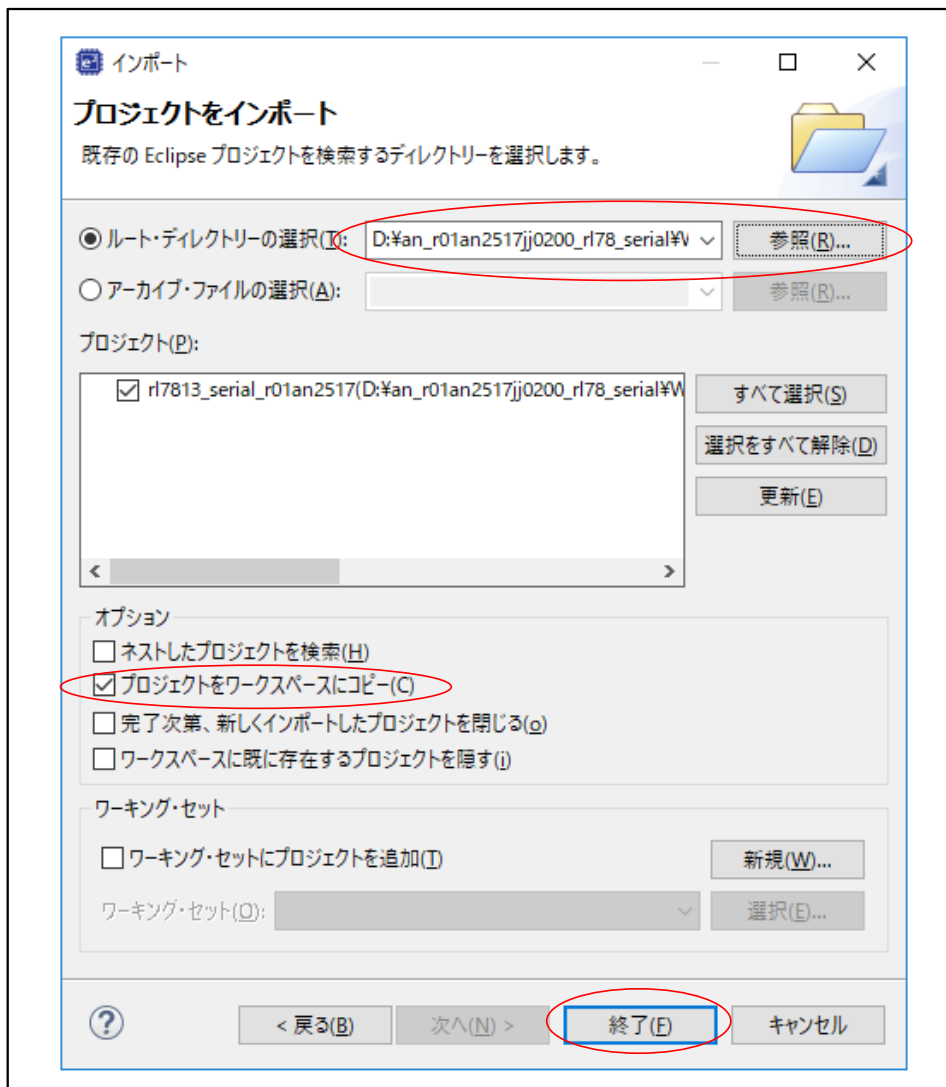
図 2-10 インポート(2/2)
