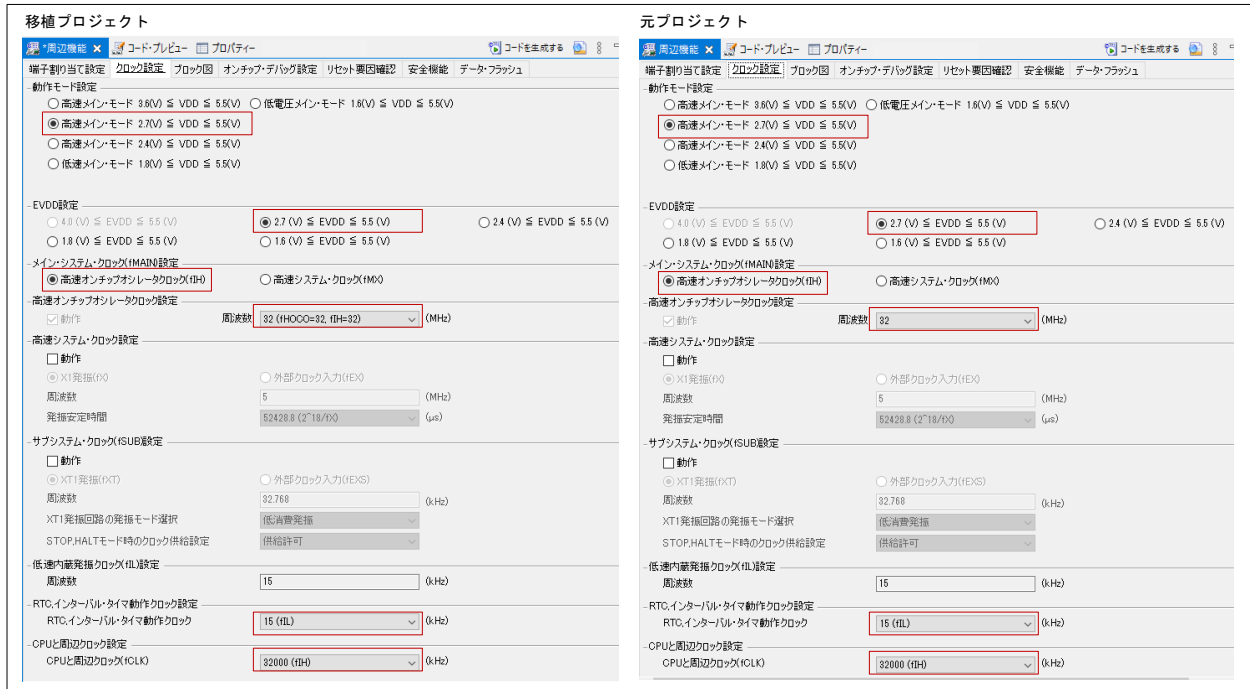
図 3-19 クロック設定 (移植例 2)
