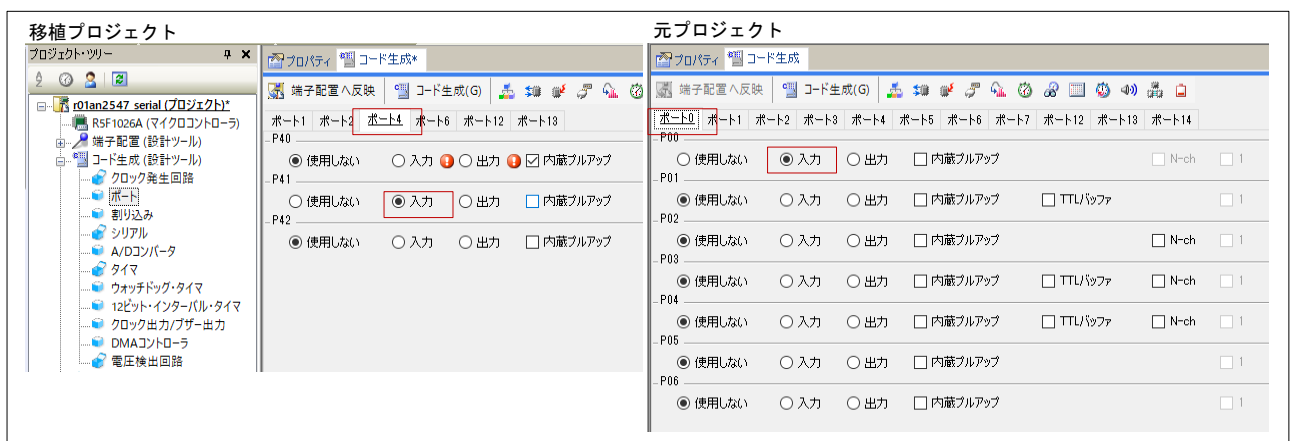
図 3-13 ポート (移植例 1)
