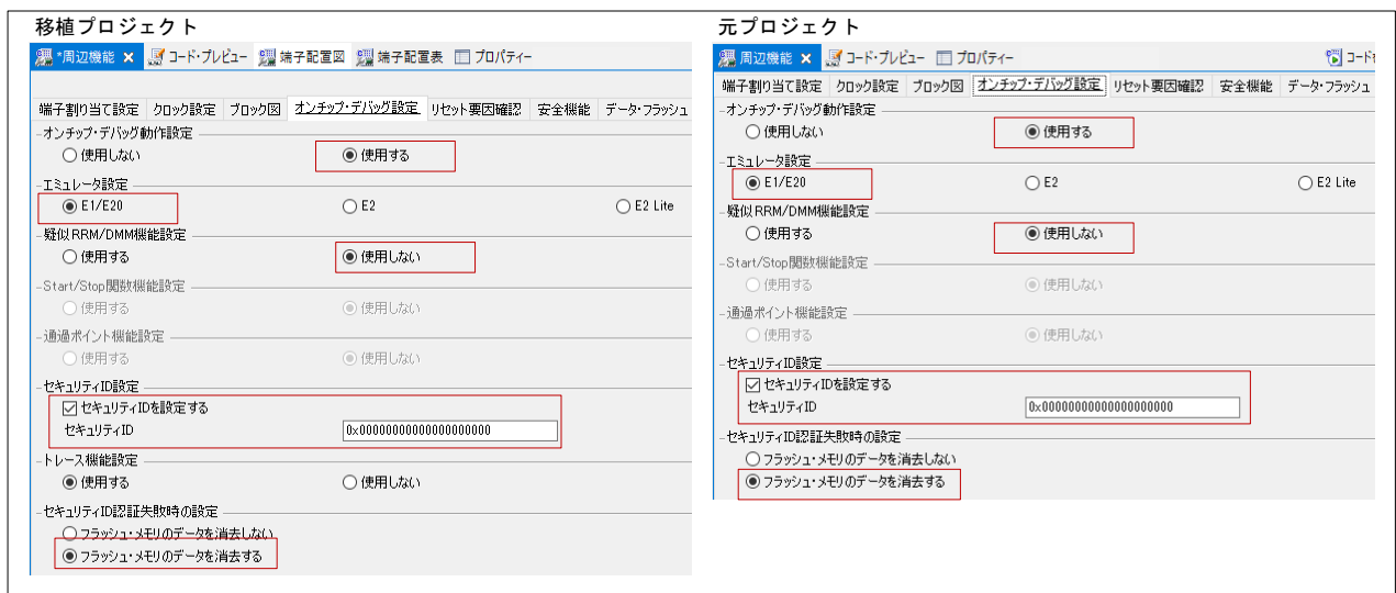
図 3-20 オンチップ・デバッグ設定 (移植例 2)
