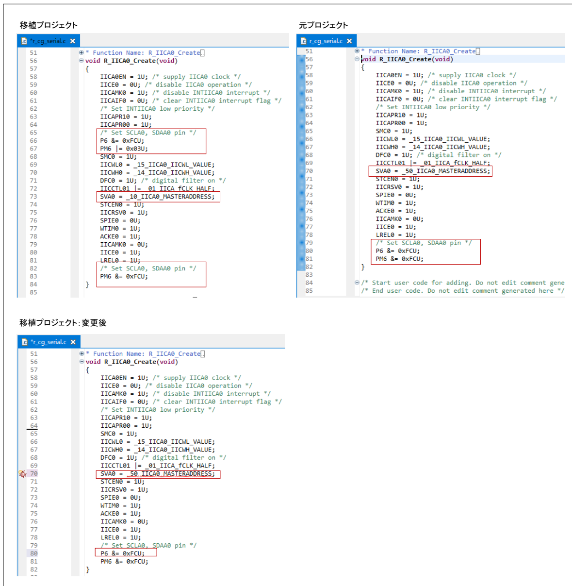
図 3-41 r_cg_serial.c –コード編集 (移植例 2)
