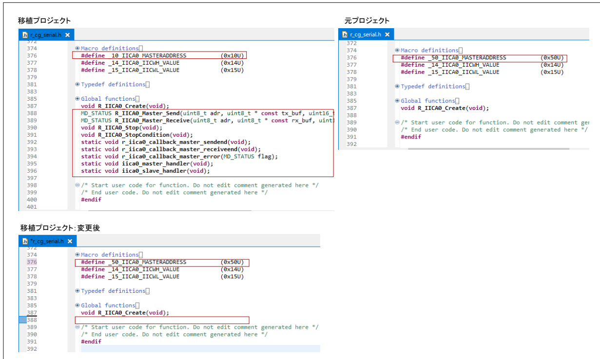
図 3-42 r_cg_serial.h (移植例 2)
