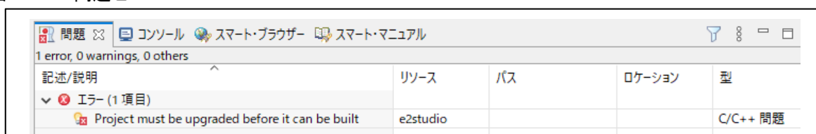
図 2-12 問題ビュー
