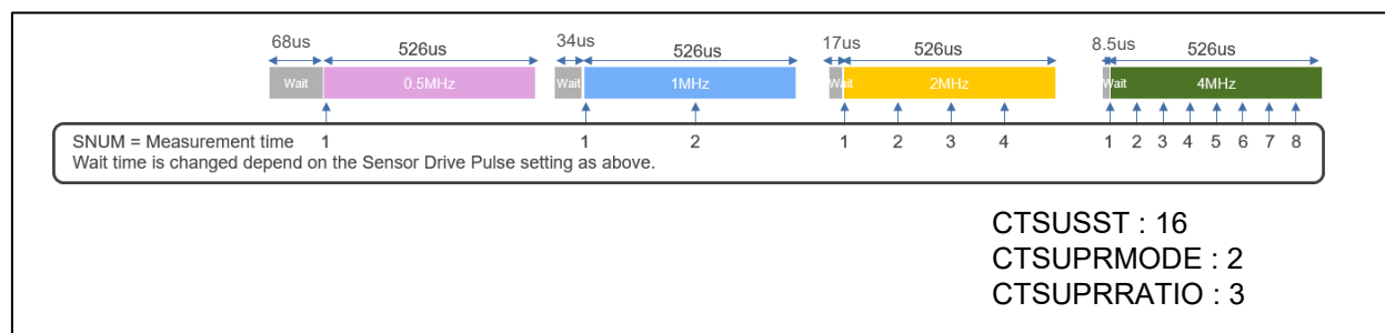
図 12 自己容量計測時間(CTS1)
