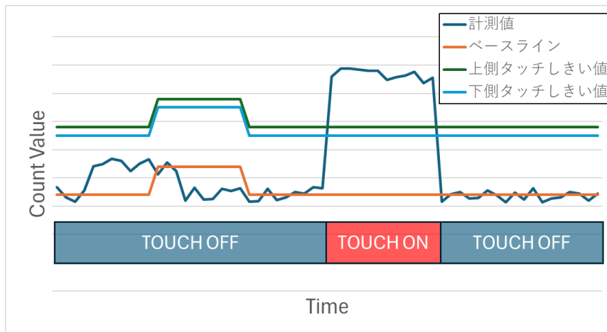
図 11 ボタンの判定
