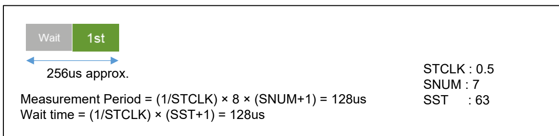
図 15 電流計測時間
