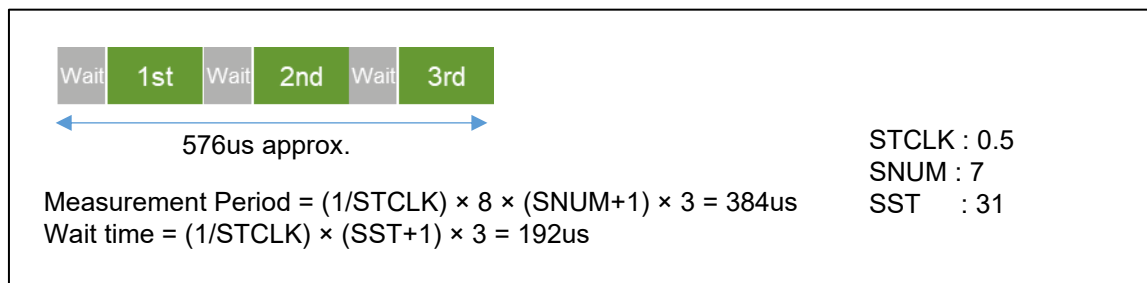
図 13 自己容量計測時間(CTS2L)
