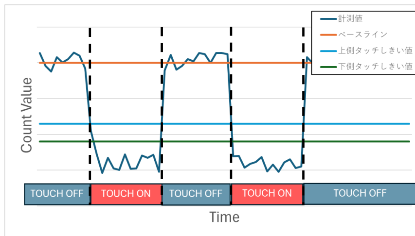
図 10 相互容量の判定
