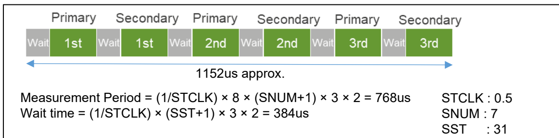
図 14 相互容量計測時間
