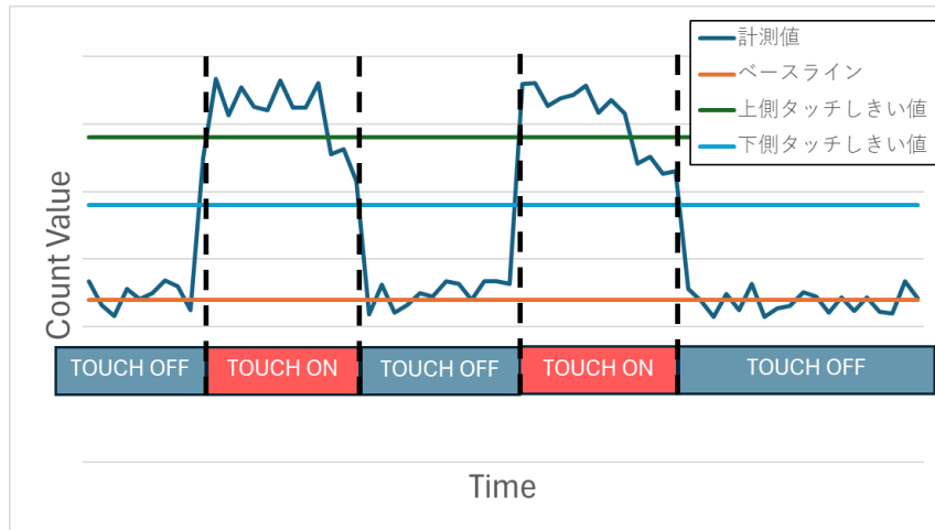
図 9 自己容量の判定
