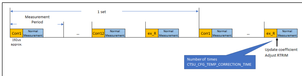
図 16 温度補正計測タイミングチャート
