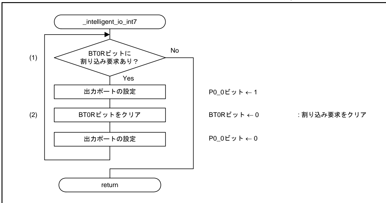
図 5.5 インテリジェントI/O 割り込み処理
