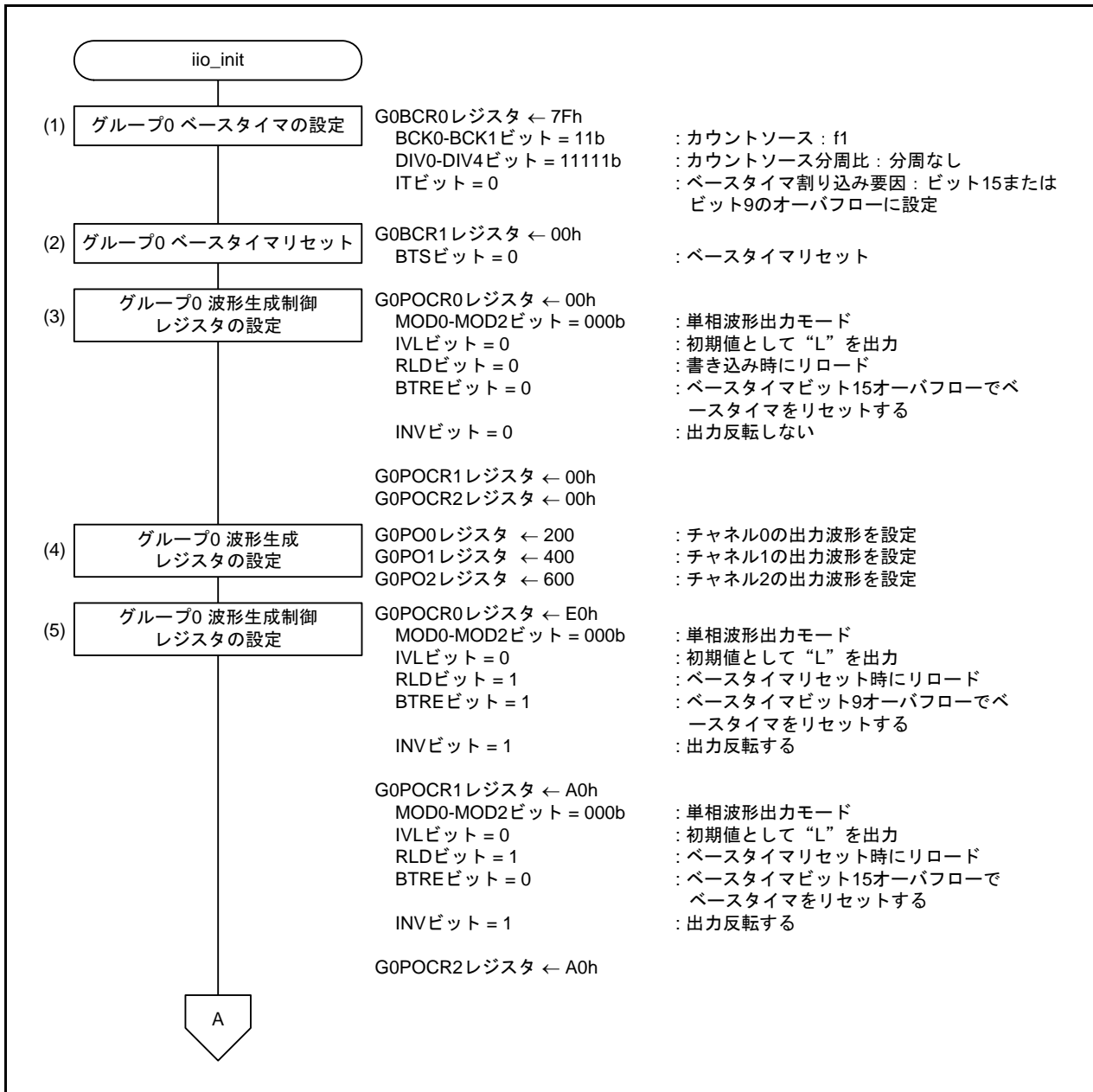
図 5.3 インテリジェント I/O 初期設定 (1/2)
