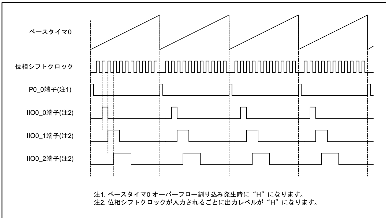
図 5.1 サンプルコードの波形出力タイミング
