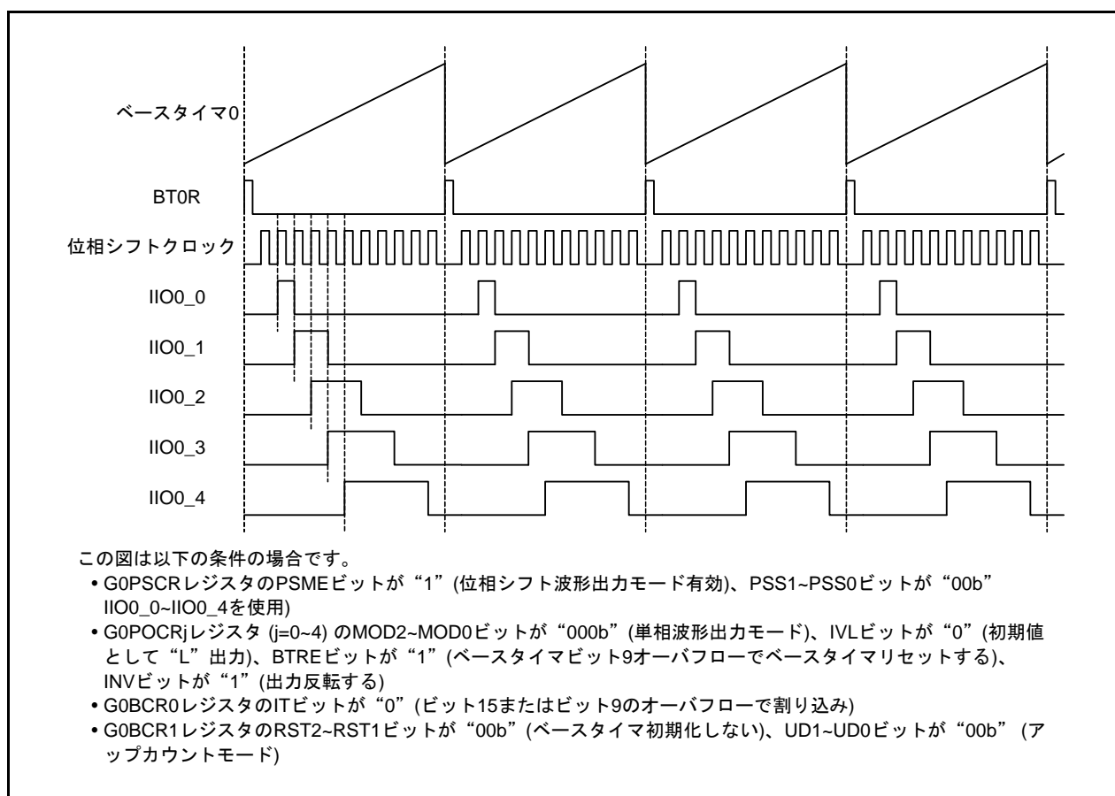
図 1.1 位相シフト波形出力モードの動作例 (i=0, 1)
