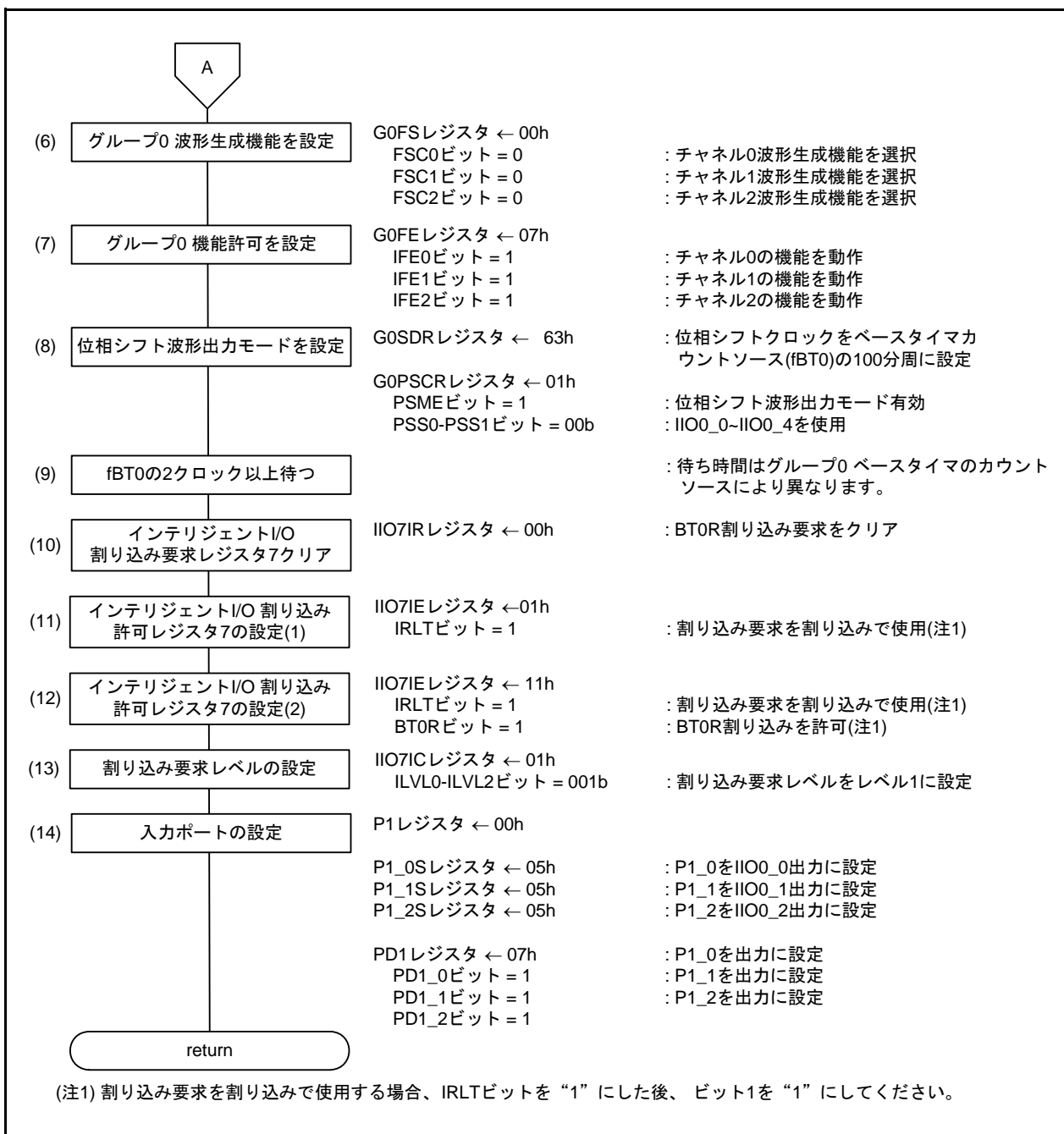
図 5.4 インテリジェント I/O 初期設定(2/2)
