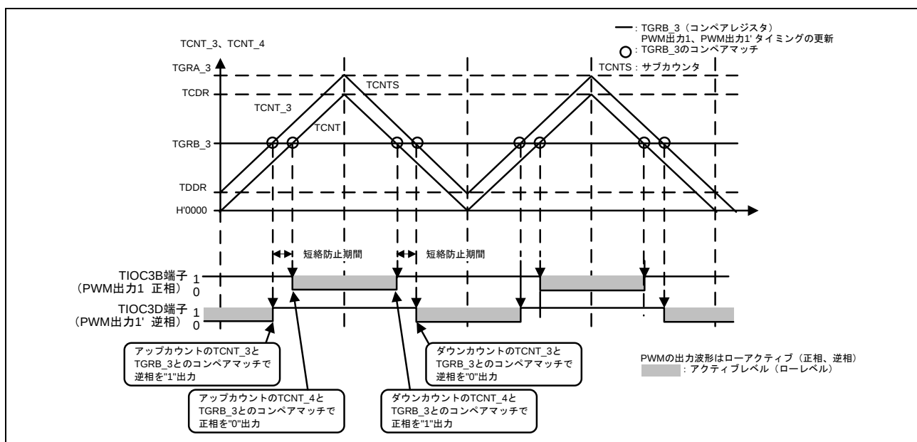
図6 相補PWMの出力波形
