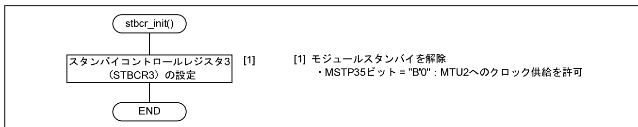
図 11 スタンバイの初期設定
