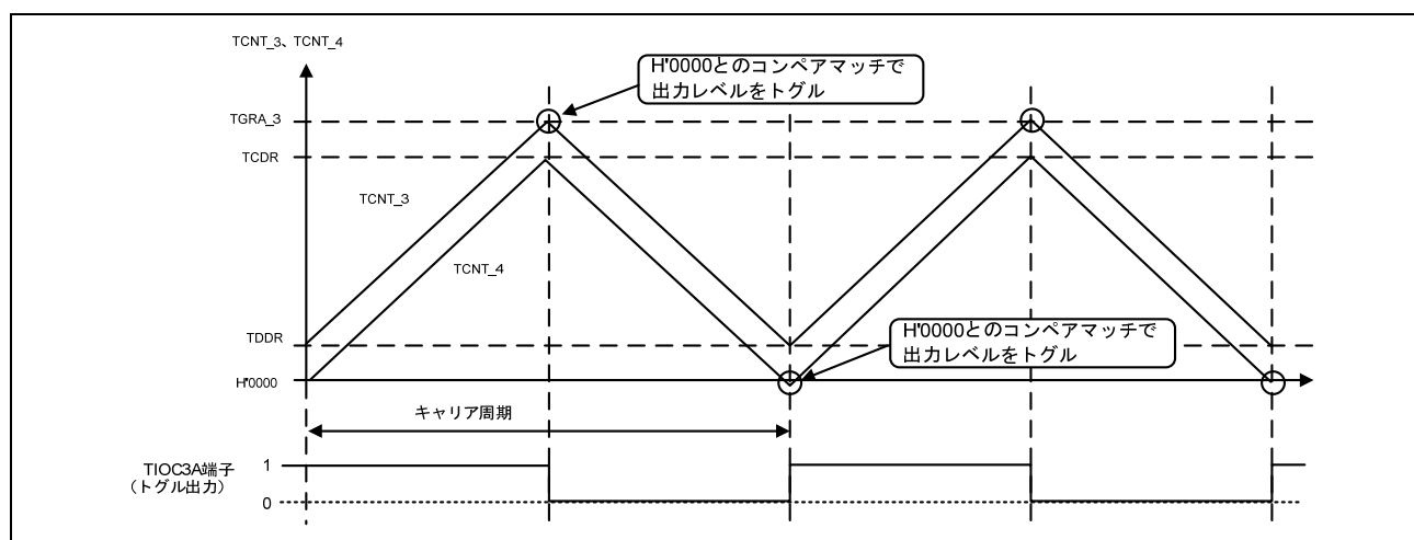
図8 PWM 周期に同期したトグル出力動作
