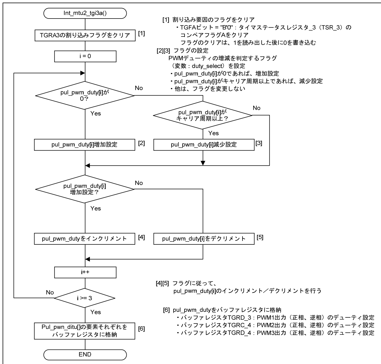
図 14 割り込み処理
