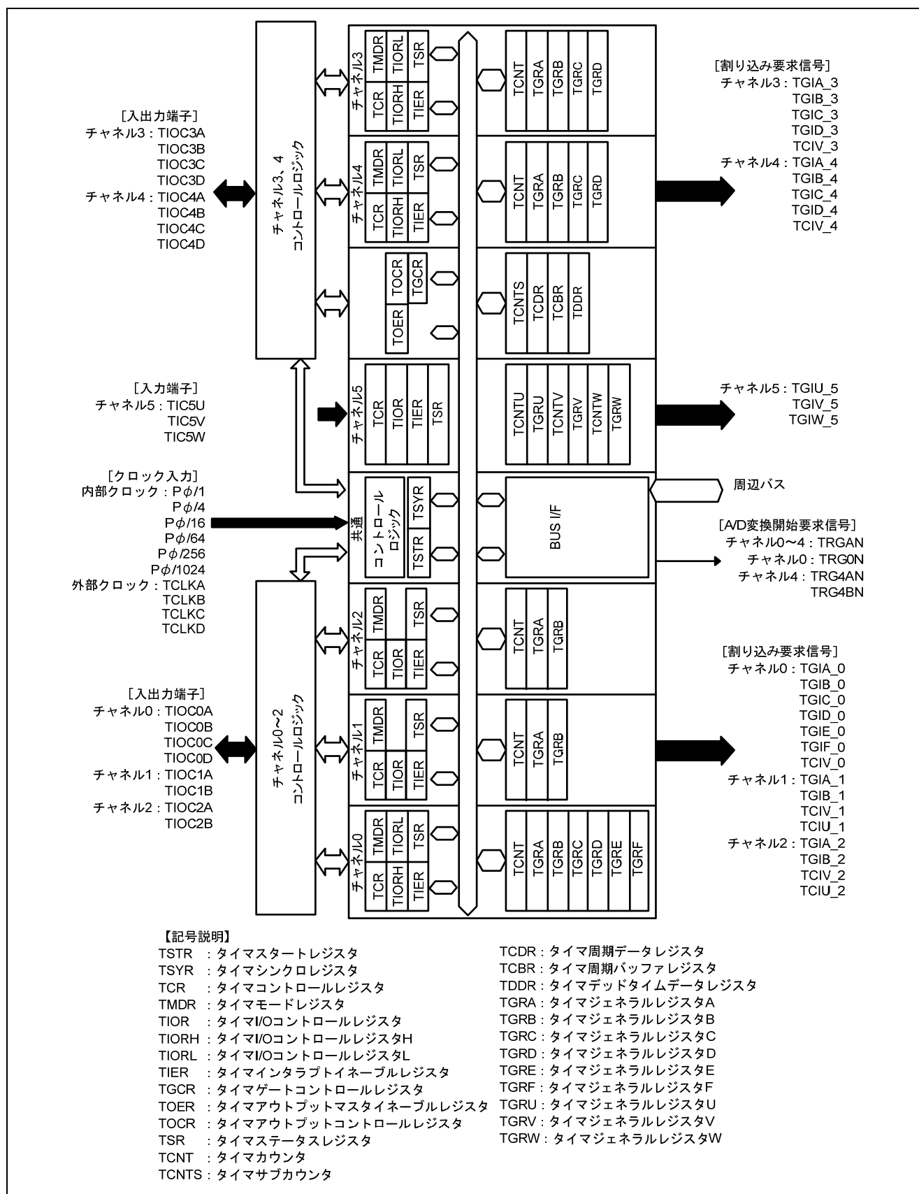
図2 MTU2 のブロック図
