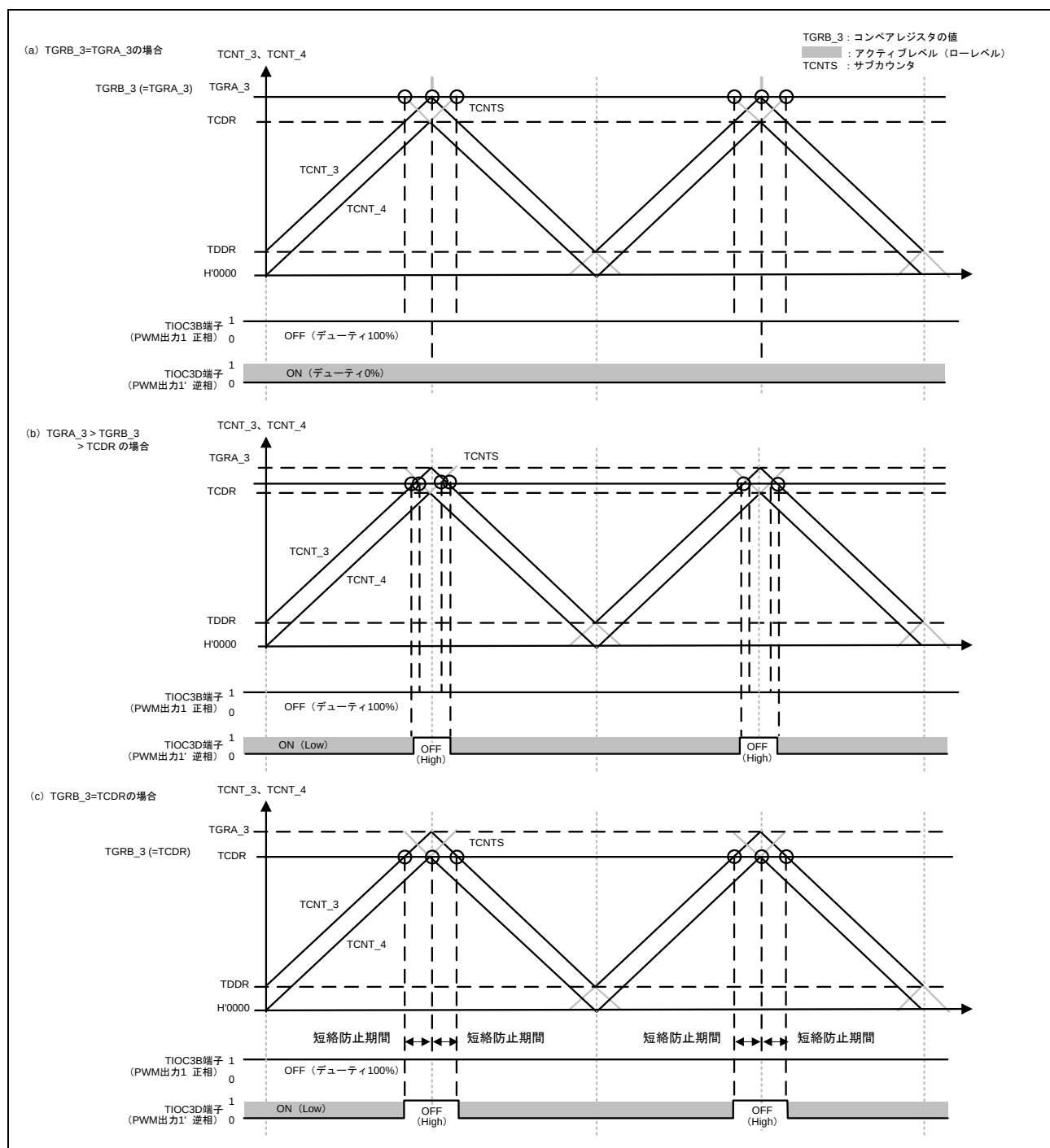
図 9 (a)、(b)、(c) PWM 波形の出力例
