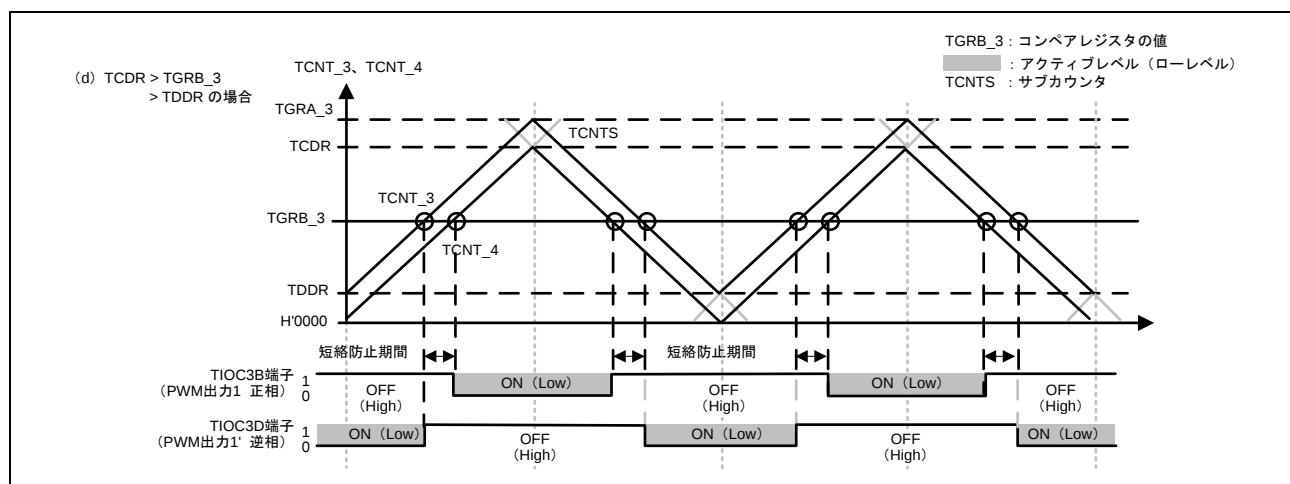
図 9 (d) PWM 波形の出力例
