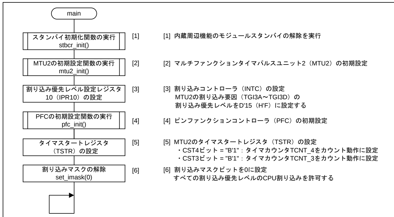
図 10 メイン関数の処理
