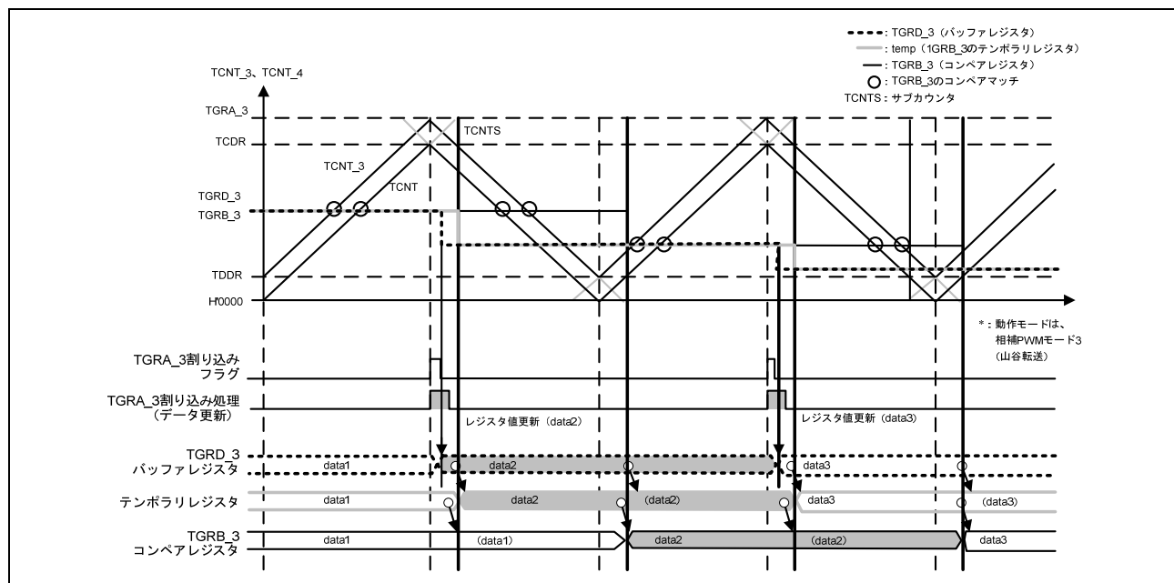
図7 PWM デューティの更新タイミング
