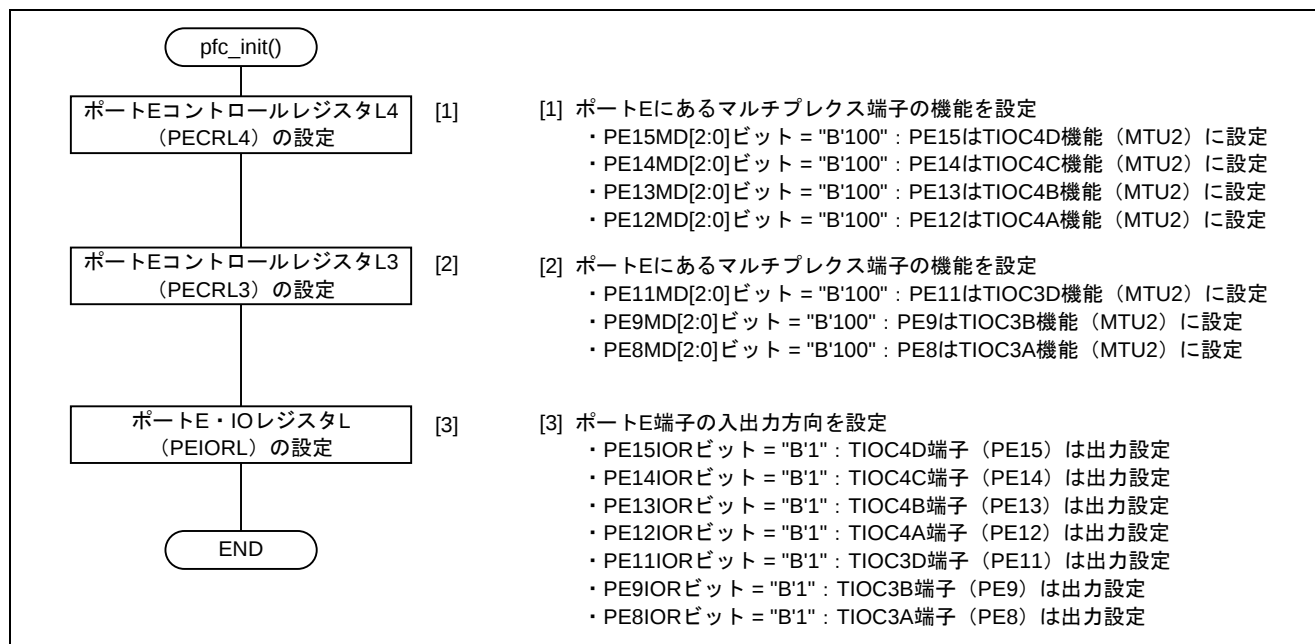
図 13 ピンファンクションコントローラ（PFC）の初期設定
