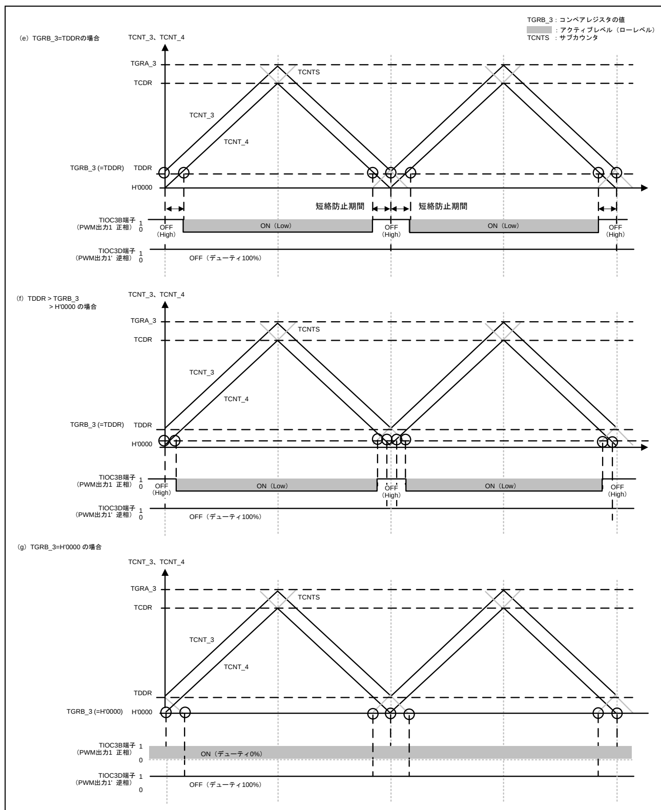
図 9 (e)、(f)、(g) PWM 波形の出力例
