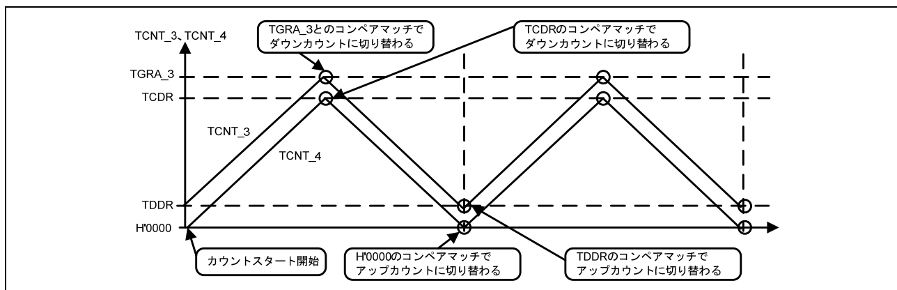
図5 タイマカウンタの動作
