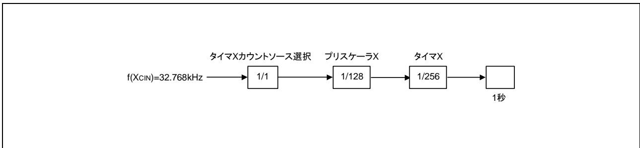
図 3.1 タイマの接続と分周比
