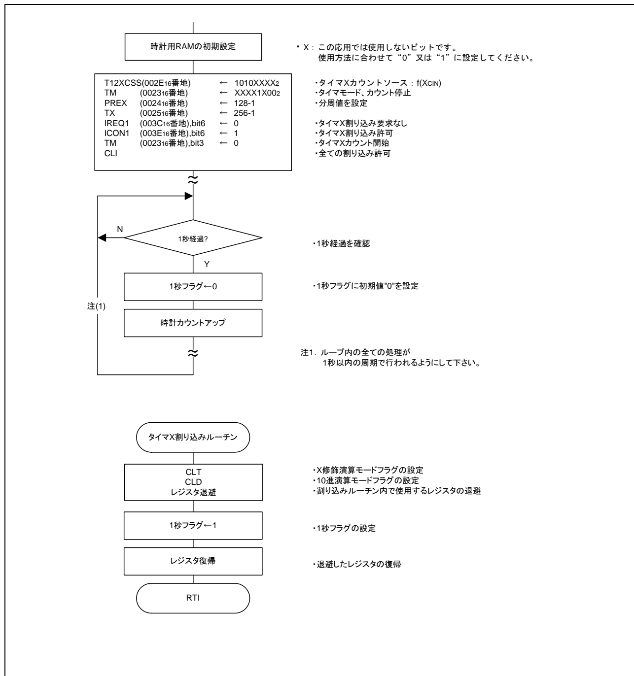
図 3.3 制御手順
