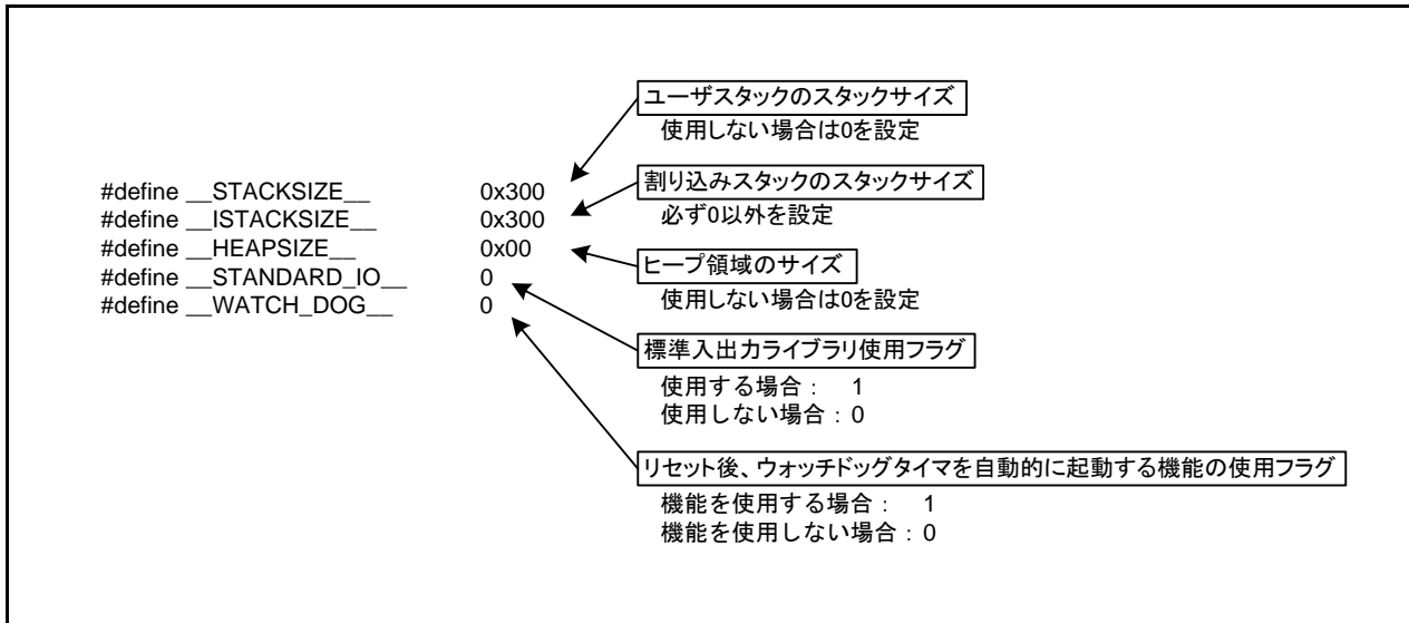
図 4.2 cstartdef.h
