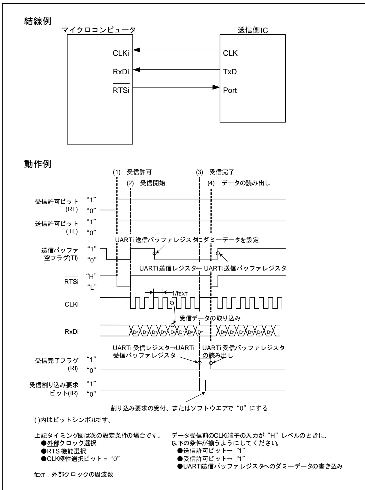
図 4.1 クロック同期形シリアルI/Oモードの受信動作タイミング
