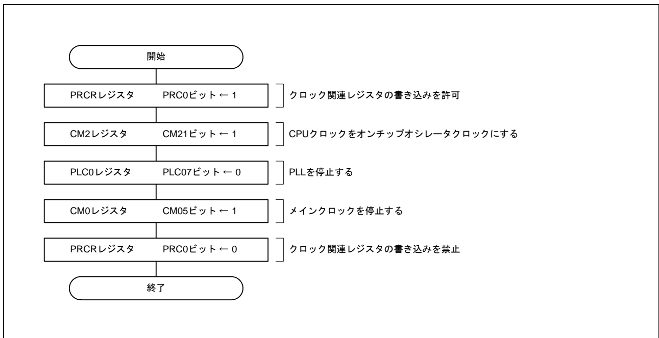
図 3.3 メインクロックモードからオンチップオシレータ低消費電力モードへの遷移手順
