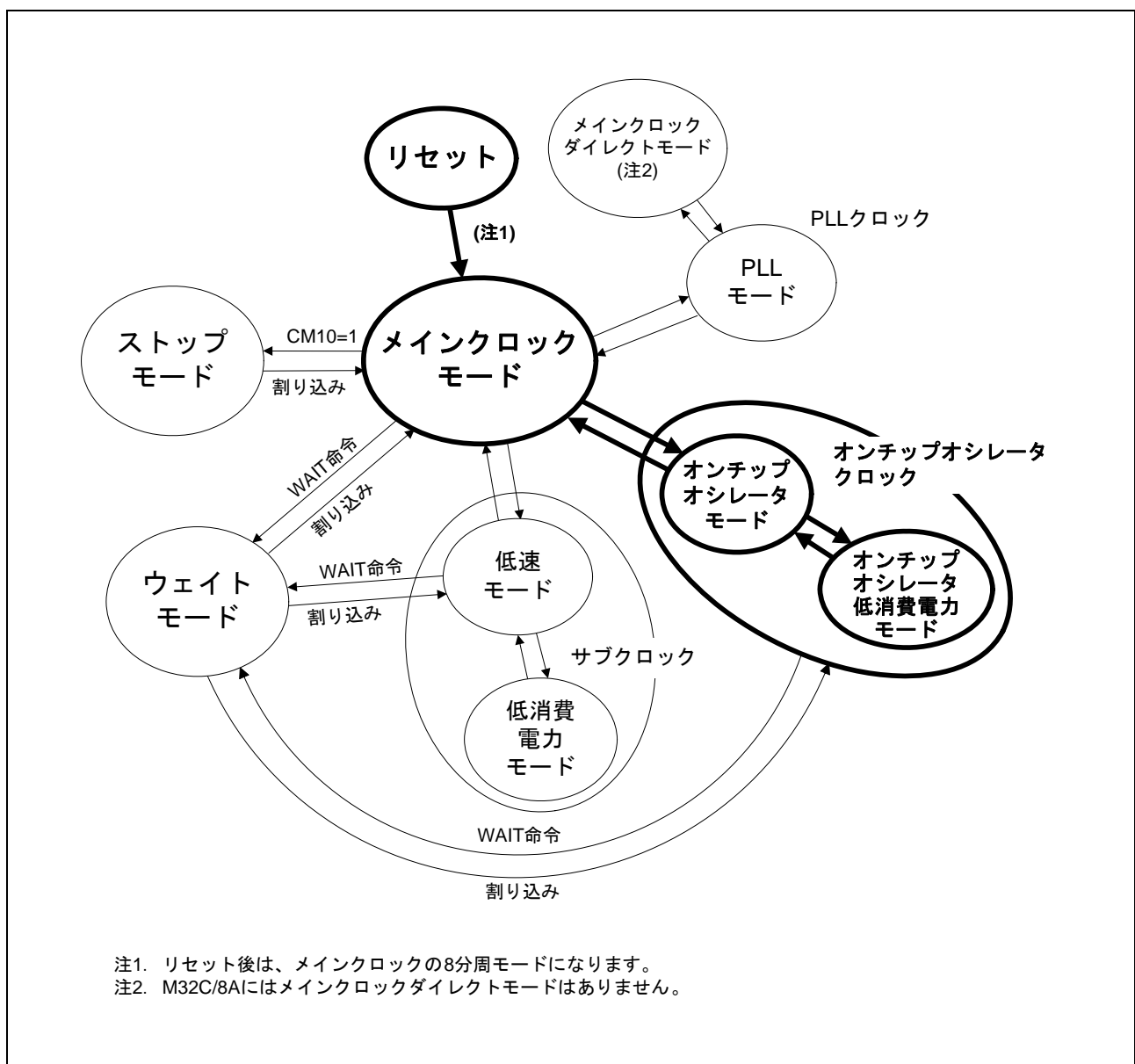
図 3.1 モード遷移図
