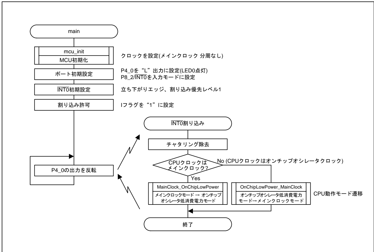
図 3.2 メイン処理のフローチャート
