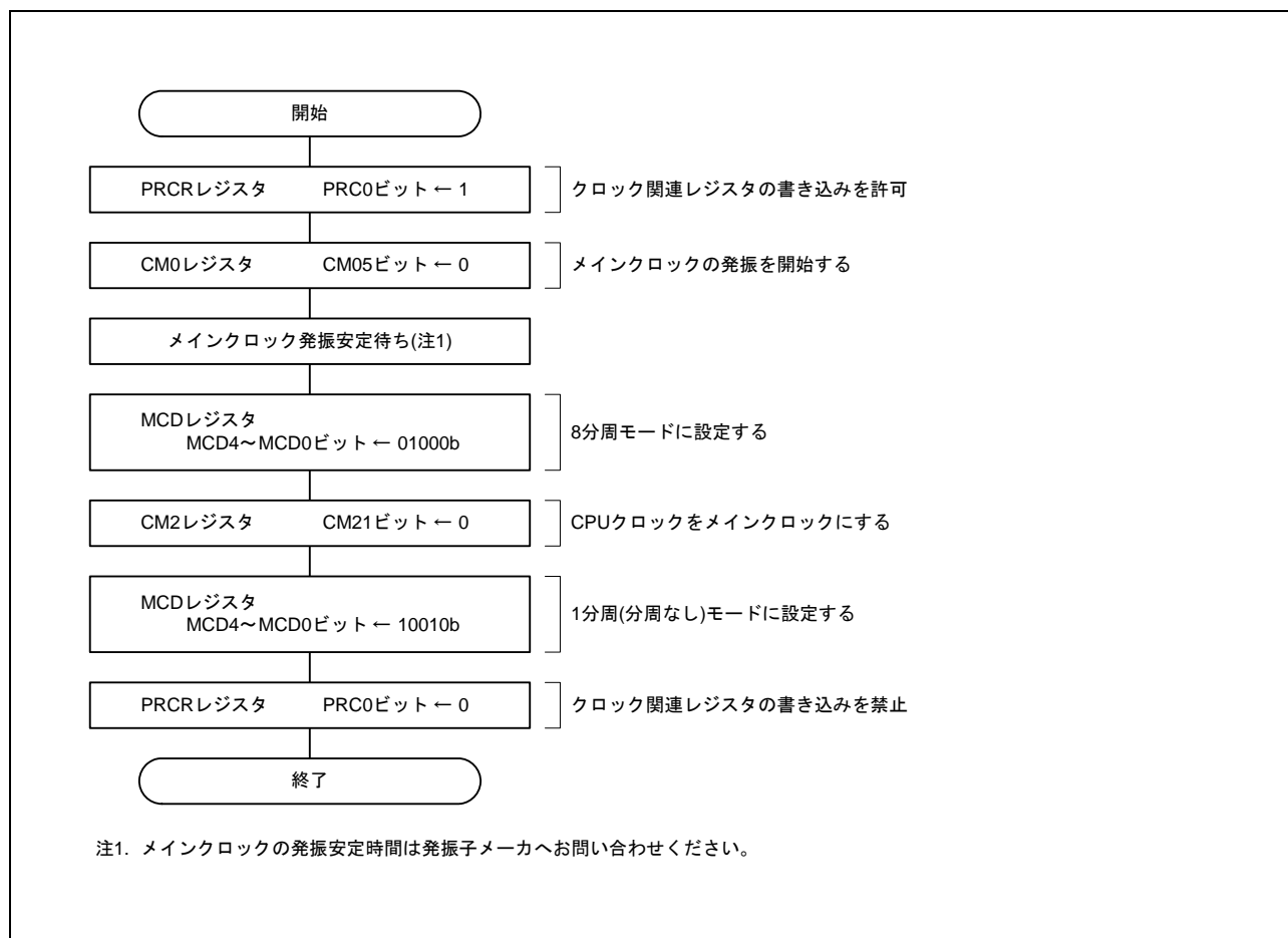
図 3.4 オンチップオシレータ低消費電力モードからメインクロックモードへの遷移手順
