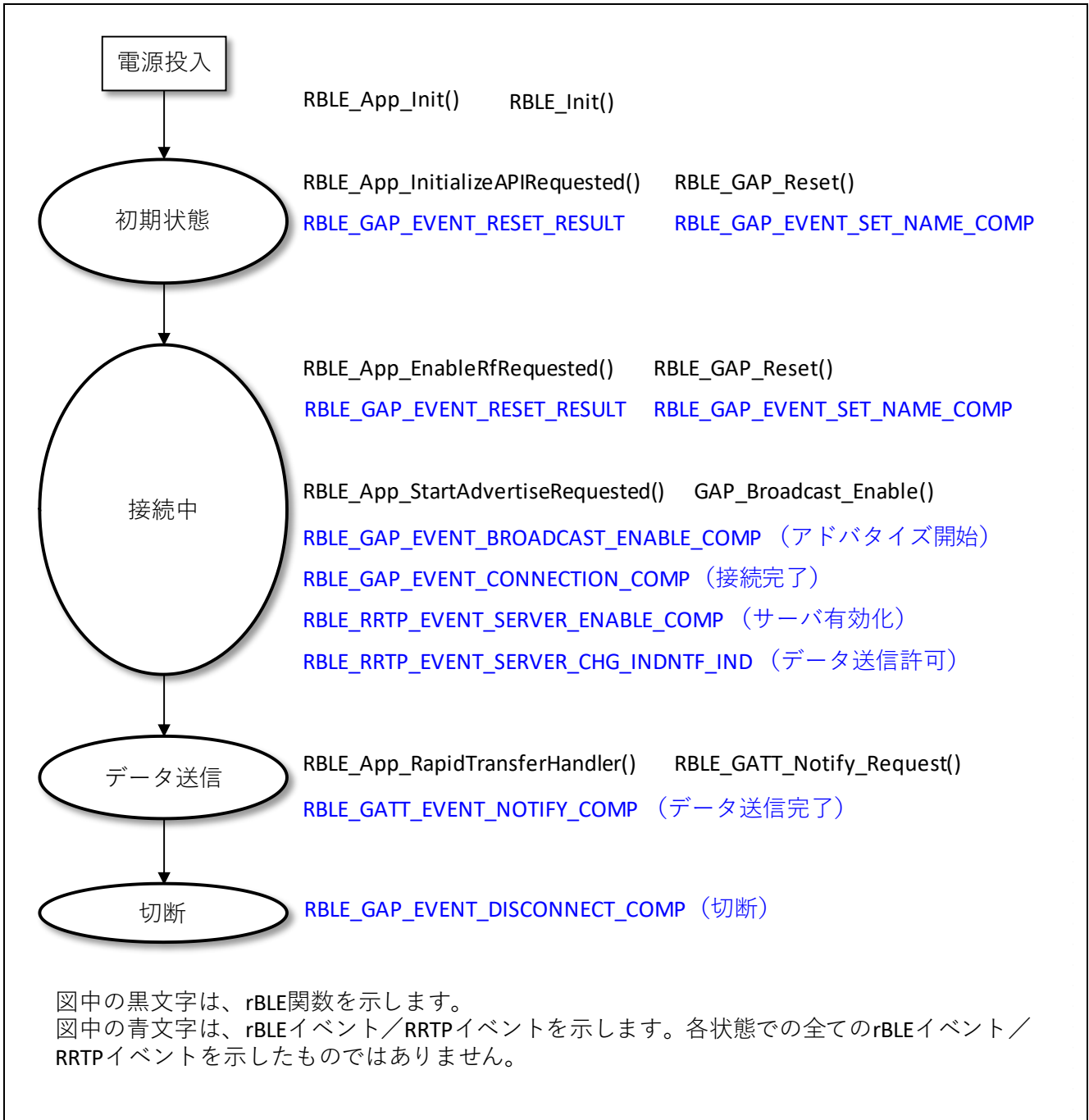
図 2-15 Peripheral 側の状態遷移
