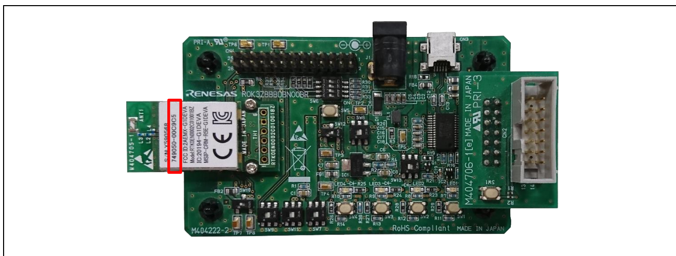
図 2-10 RL78/G1D 搭載モジュール(RTK0EN0002C01001BZ) BD Address
