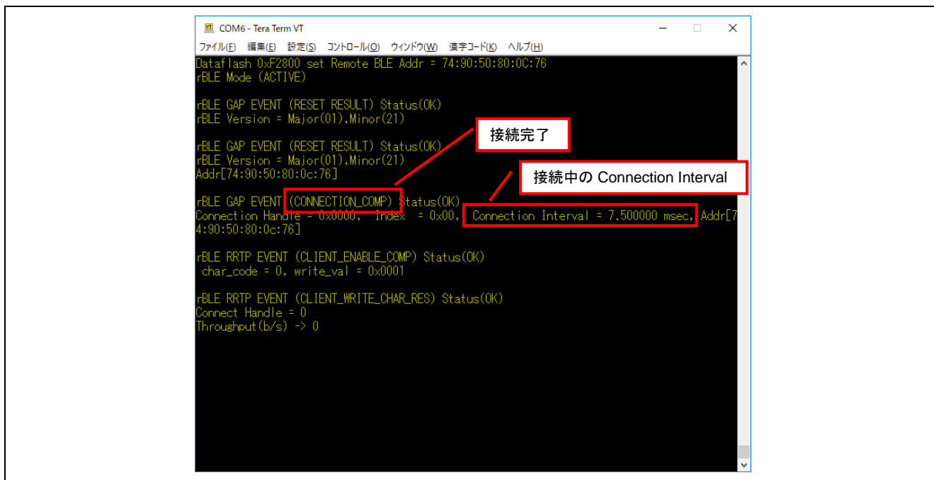
図 3-5 自動接続完了のログ出力
