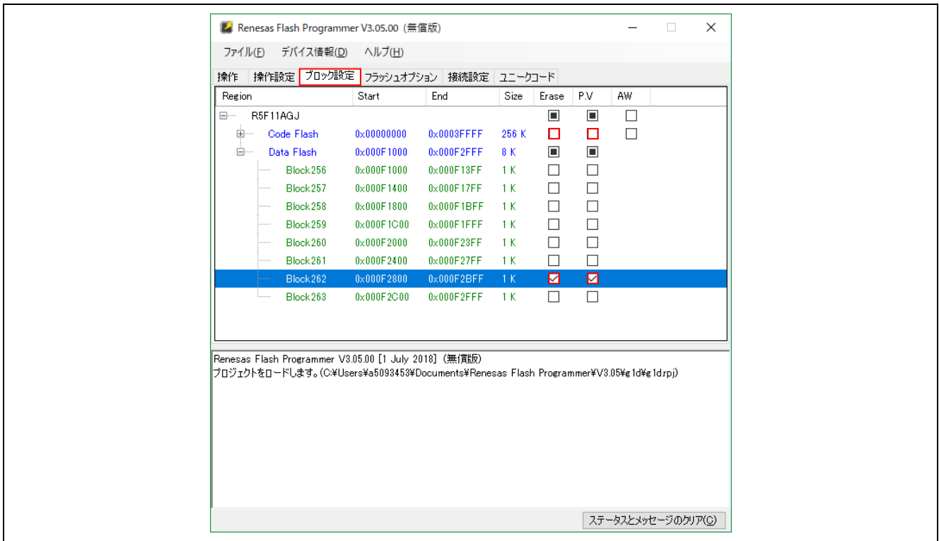
図 2-13 RFP ブロック設定タブ
