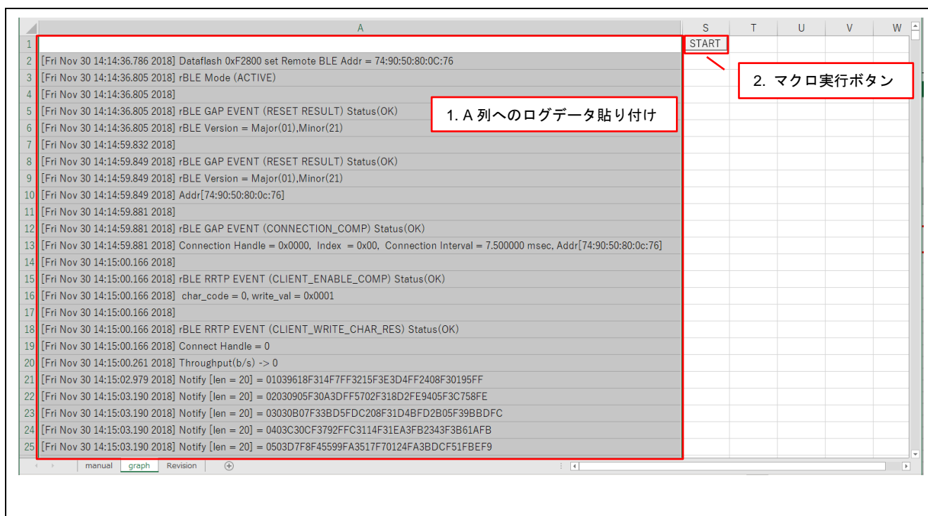
図 3-7 ログデータのグラフ化操作
