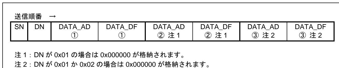
図 3-2 送信データ（パケット）フォーマット
