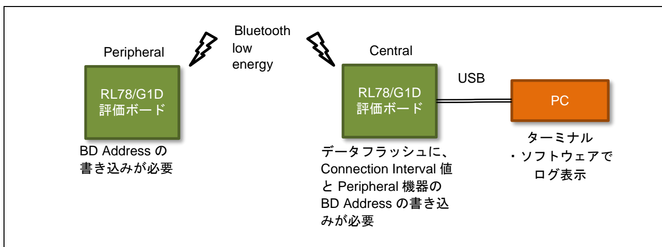
図 2-8 動作確認用簡易デモシステム構成
