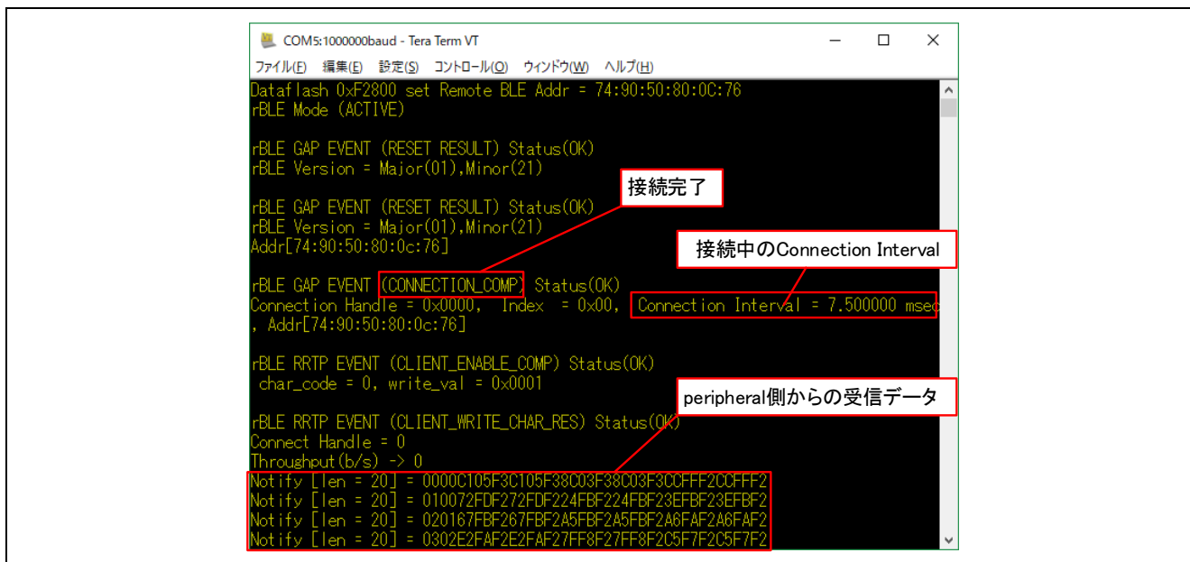
図 2-18 自動接続完了とデータ受信のログ出力
