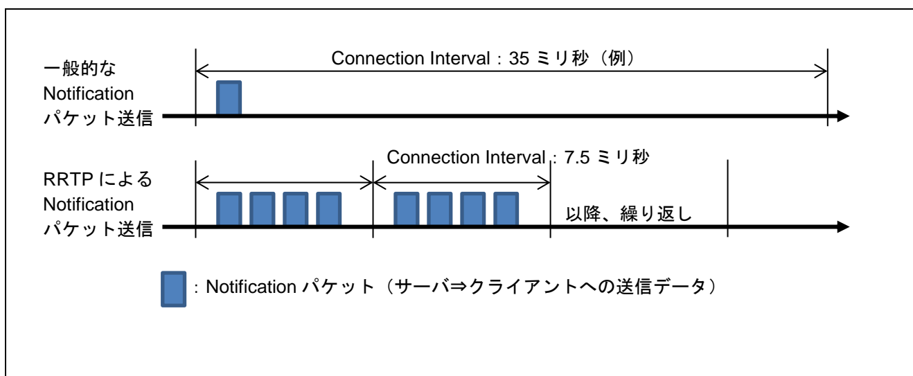
図 2-1 RRTP の Notification パケットによる通知 (サーバからのデータ送信)
