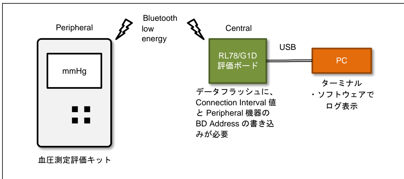
図 3-1 高速データ転送動作デモシステム構成
