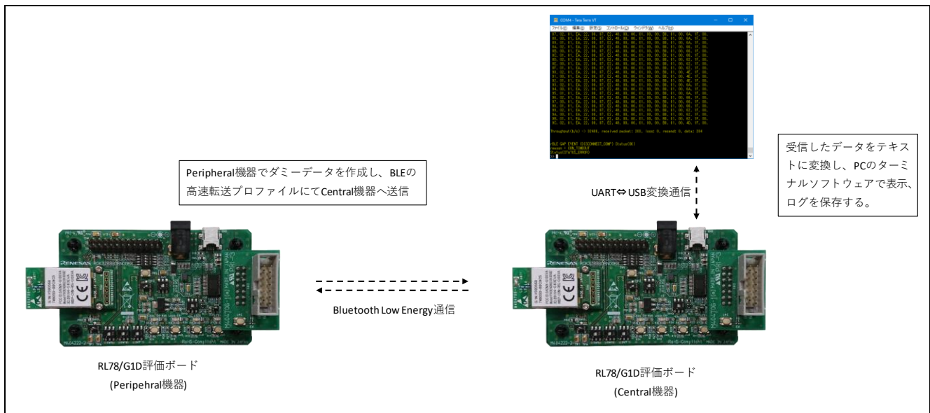
図 1-1 サンプルプログラムの動作環境概要
