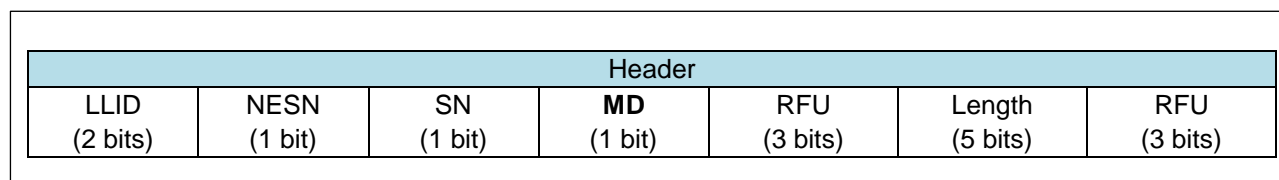
図 2-3 PDU header の構造 (Bluetooth Ver.4.1 の場合)
