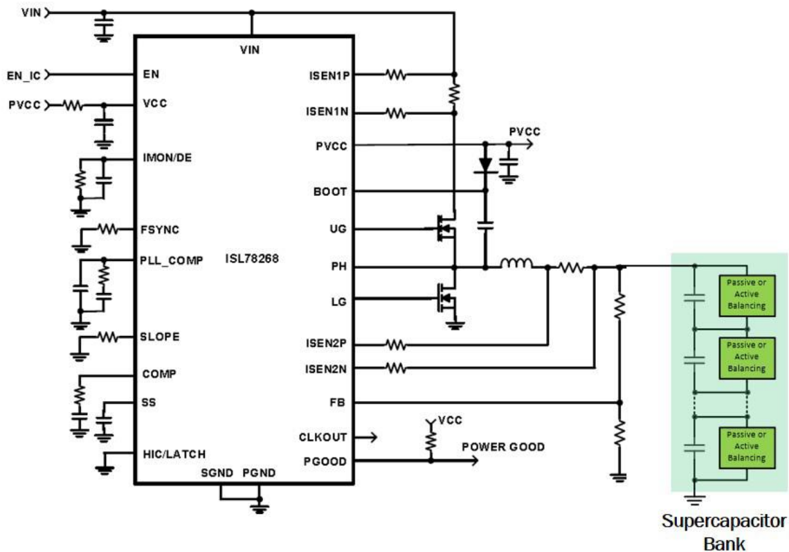
图3：无源或有源平衡 无源或有源平衡 无源或有源平衡 超级电容器组
