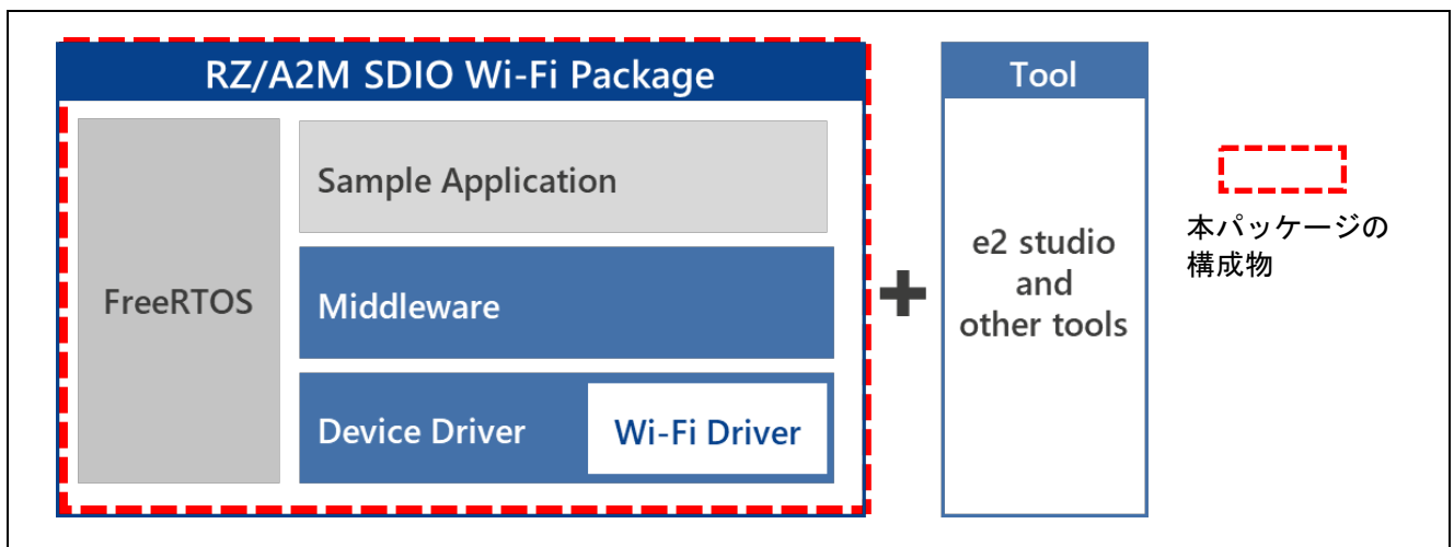
図 2 RZ/A2M SDIO Wi-Fi Package のソフトウェア構造
