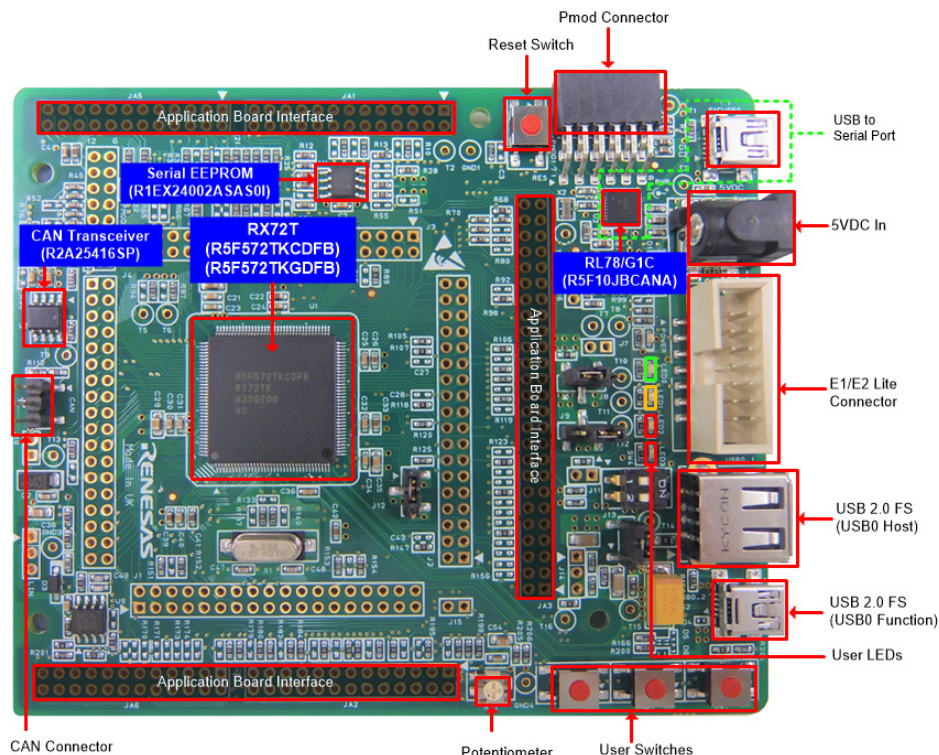
図 2 CPU ボード図 (部品面)
