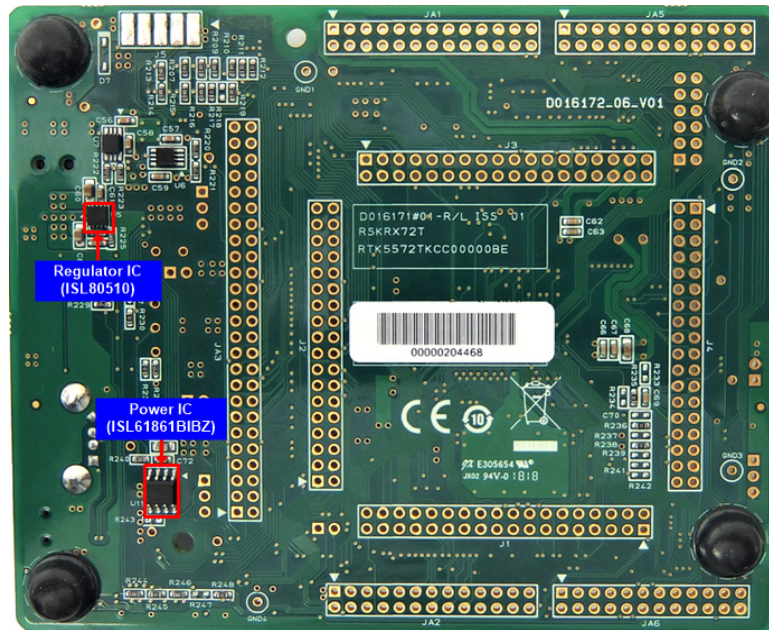
図3 CPUボード図（ハンダ面）
