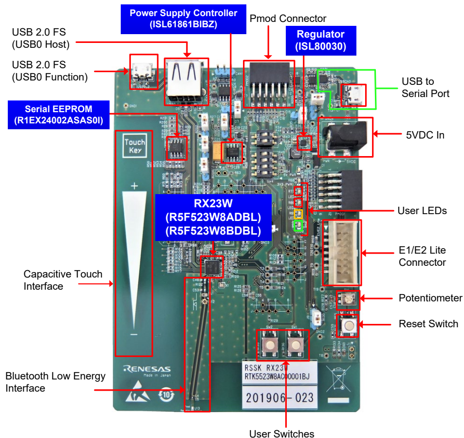
図 2 CPU ボード図 (部品面)
