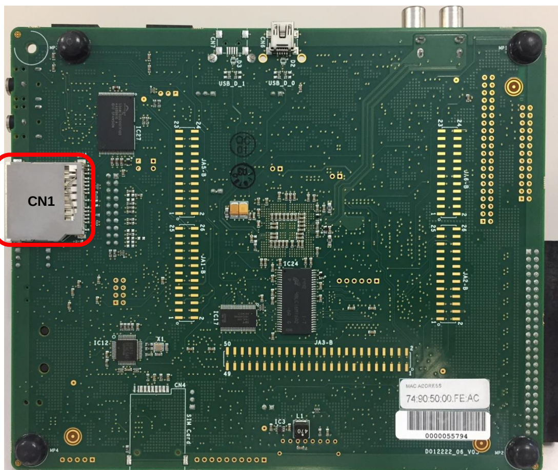
図 1 SD/MMC スロット位置（ボード S 面）
