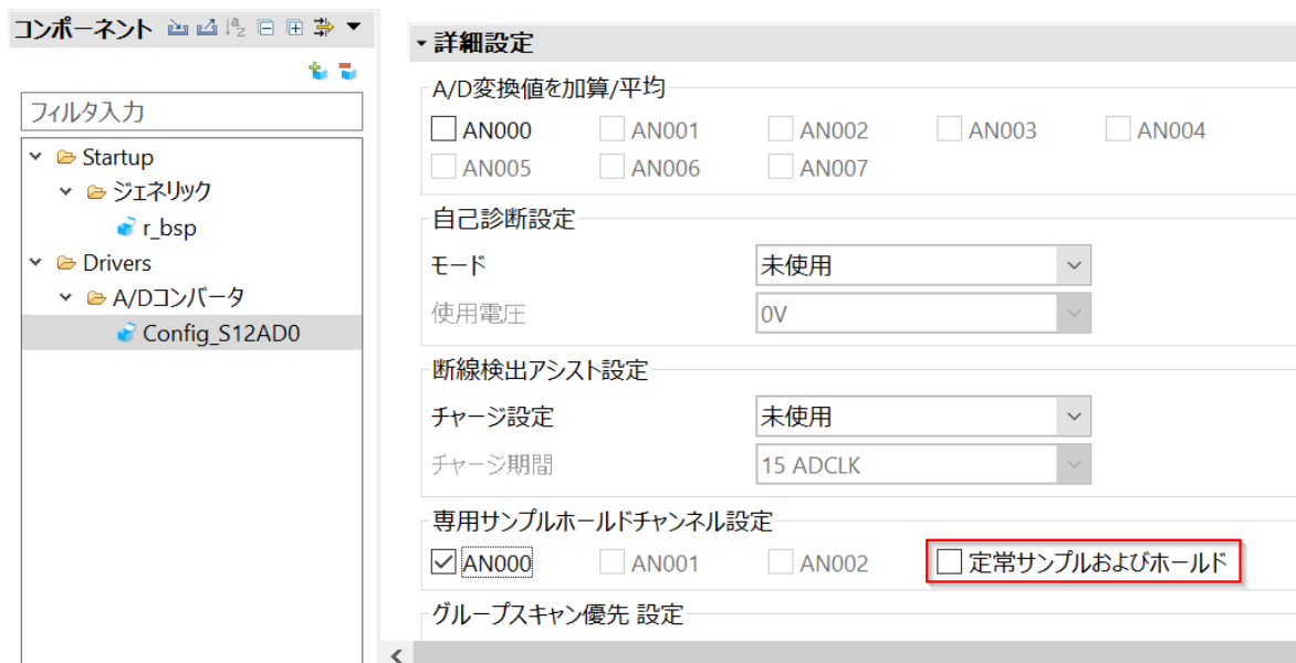
図 2-5 常時サンプリングを有効にするチェックボックス
