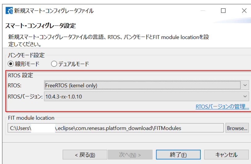
図 2-1 プロジェクト作成時の FreeRTOS カーネル選択
