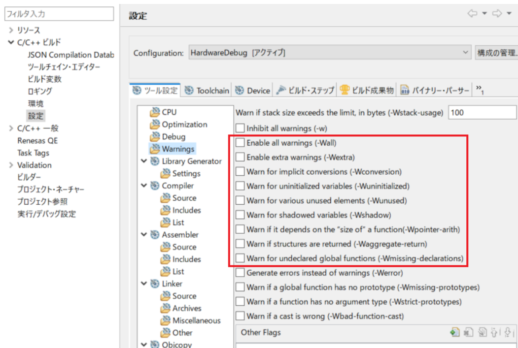
図 3-2 GCC 警告設定
