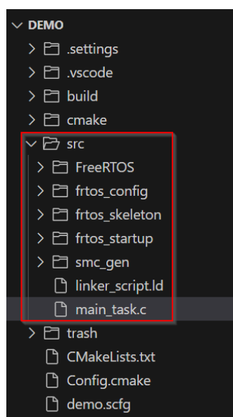
図 2-2 FreeRTOS カーネルを選択して作成されたプロジェクト
