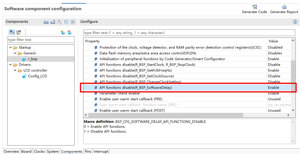
Figure 3-2 Enable R_BSP_SoftwareDelay function
