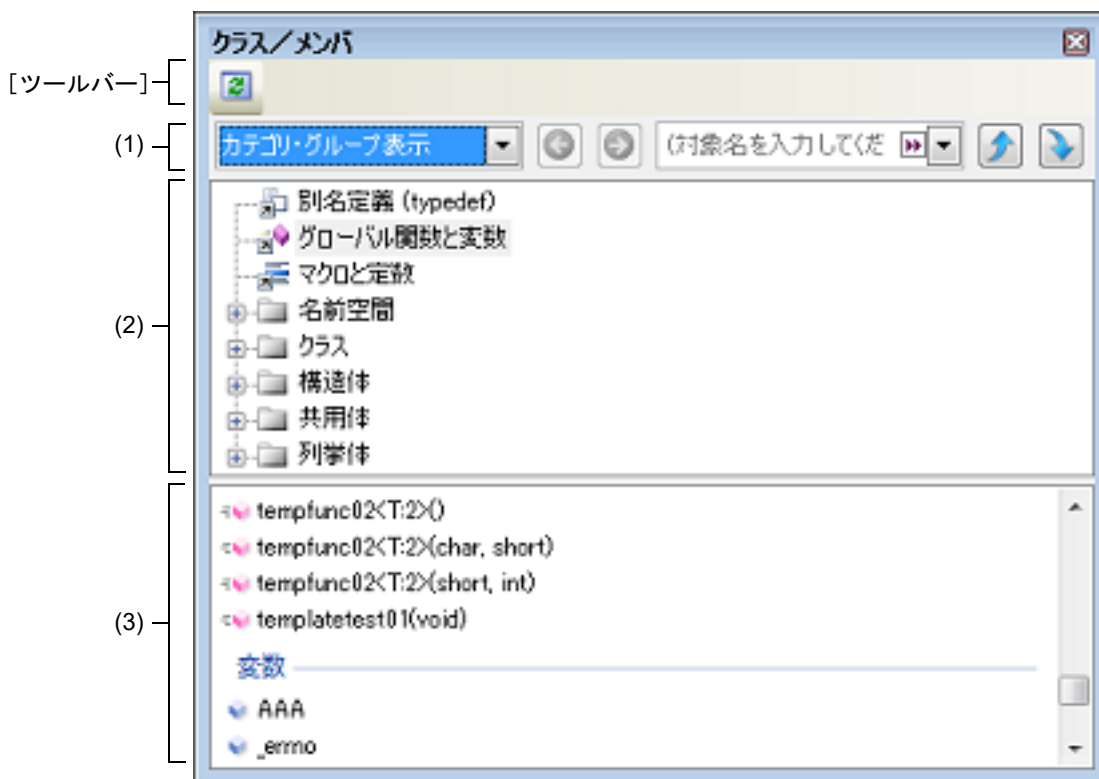
図 A.22 クラス／メンバパネル
