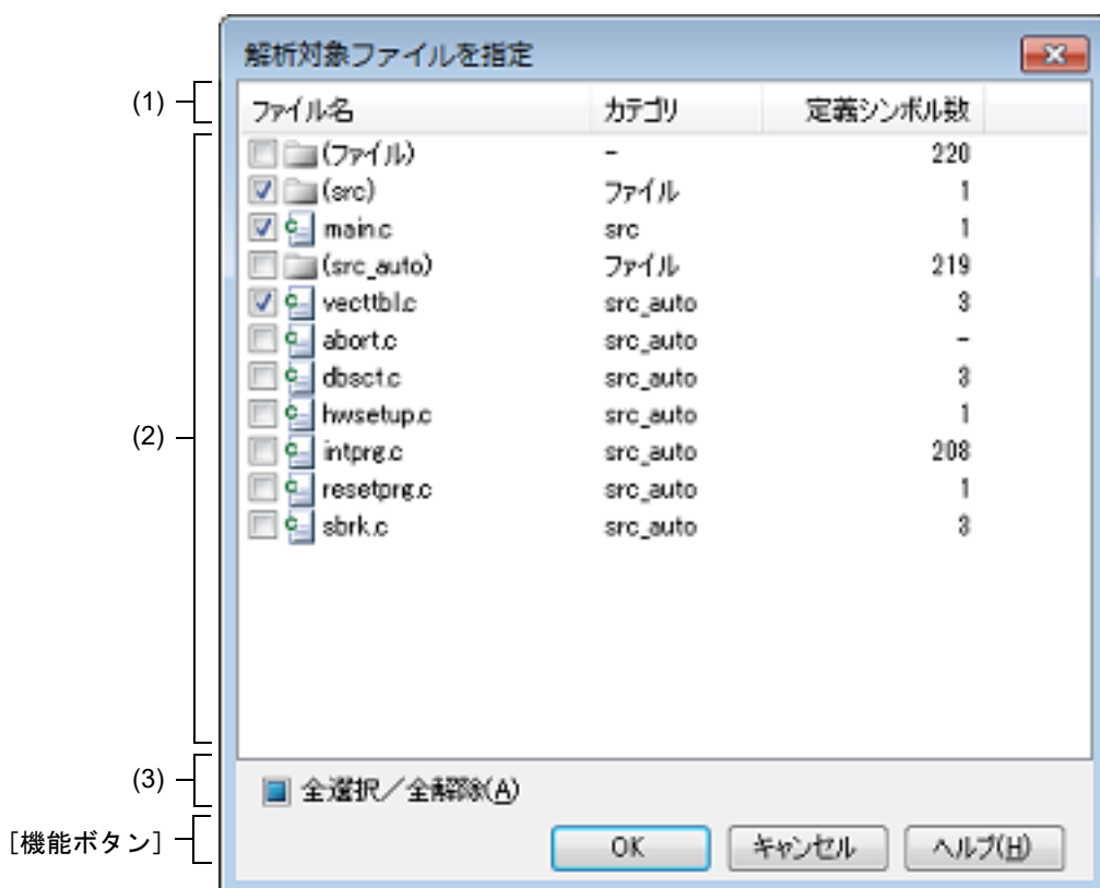
図 A.40 解析対象ファイルを指定 ダイアログ
