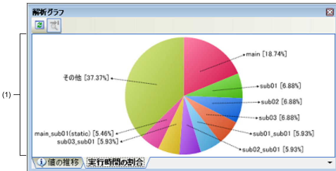
図 A.15 解析グラフ パネル：〔実行時間の割合〕タブ
