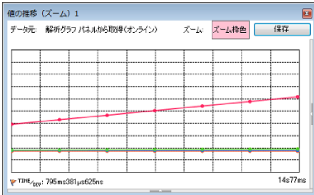
図 2.35 ズーム表示（値の推移（ズーム）パネル）
