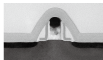
40nmトランジスタ断面図
