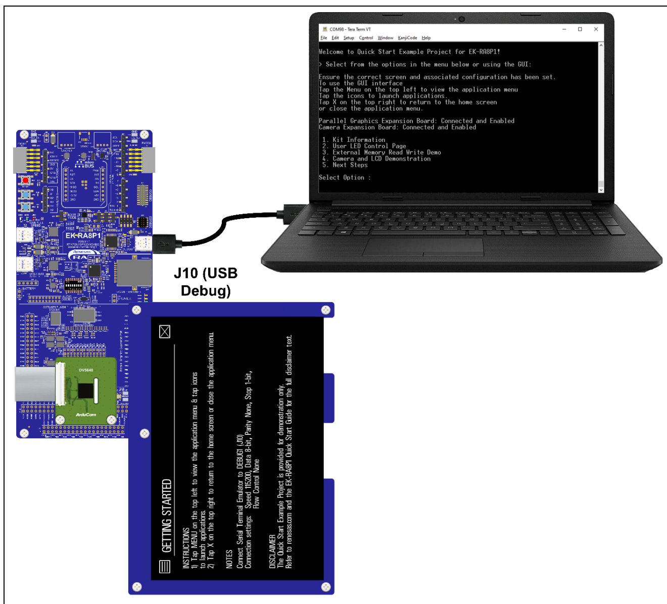
図 4. EK-RA8P1 ボードを USB デバッグ経由でホスト PC に接続
