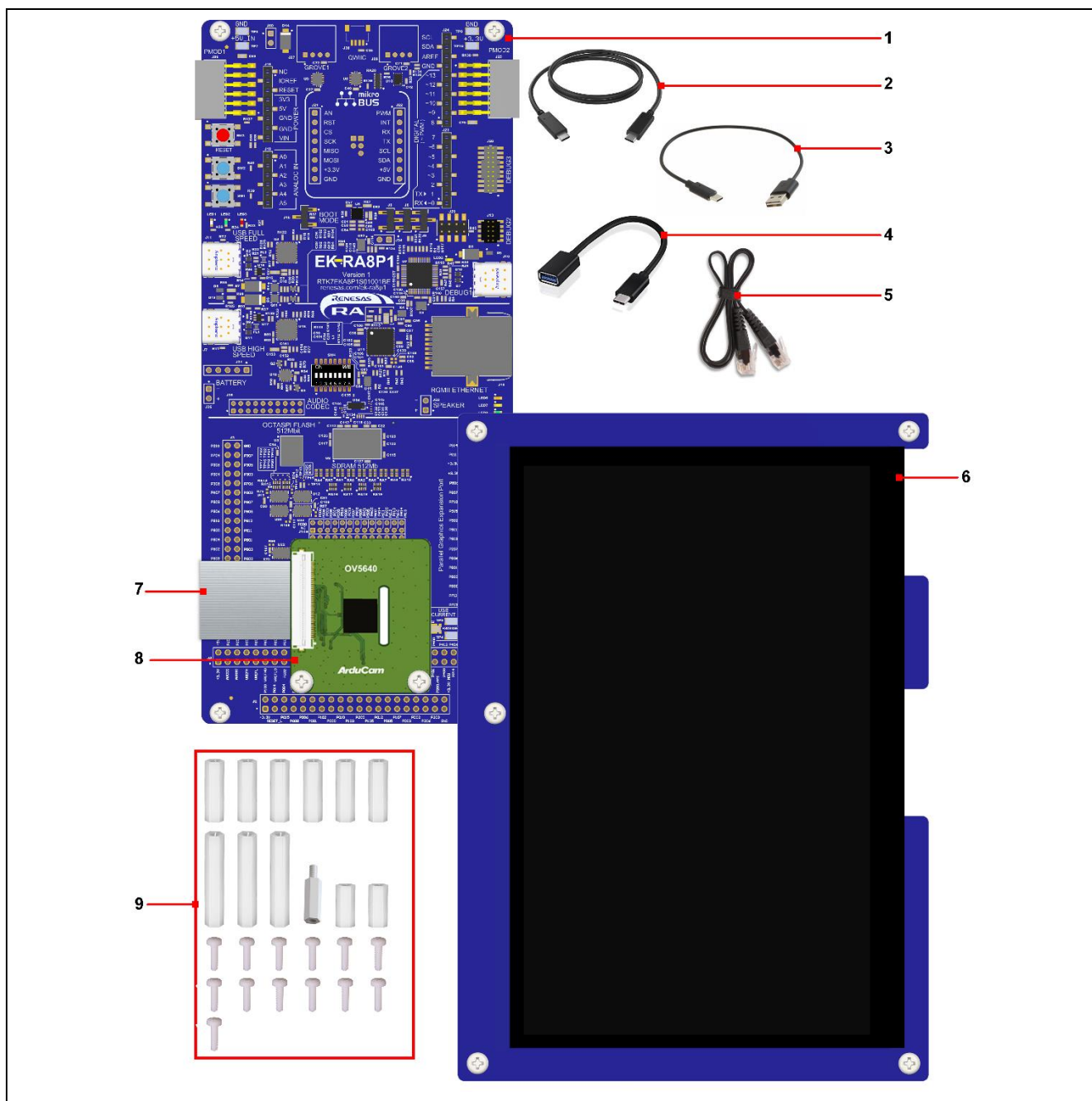
図 1. EK-RA8P1 キットの構成
