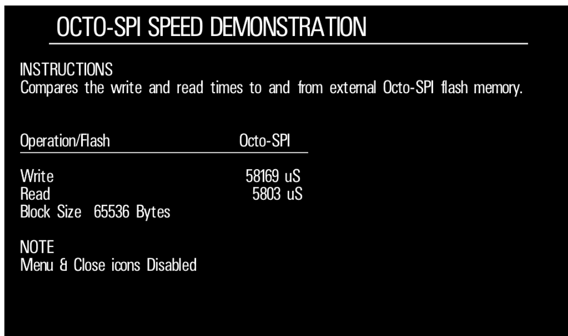
図 18. パラレルディスプレイ：外部メモリのリードライトデモ結果
