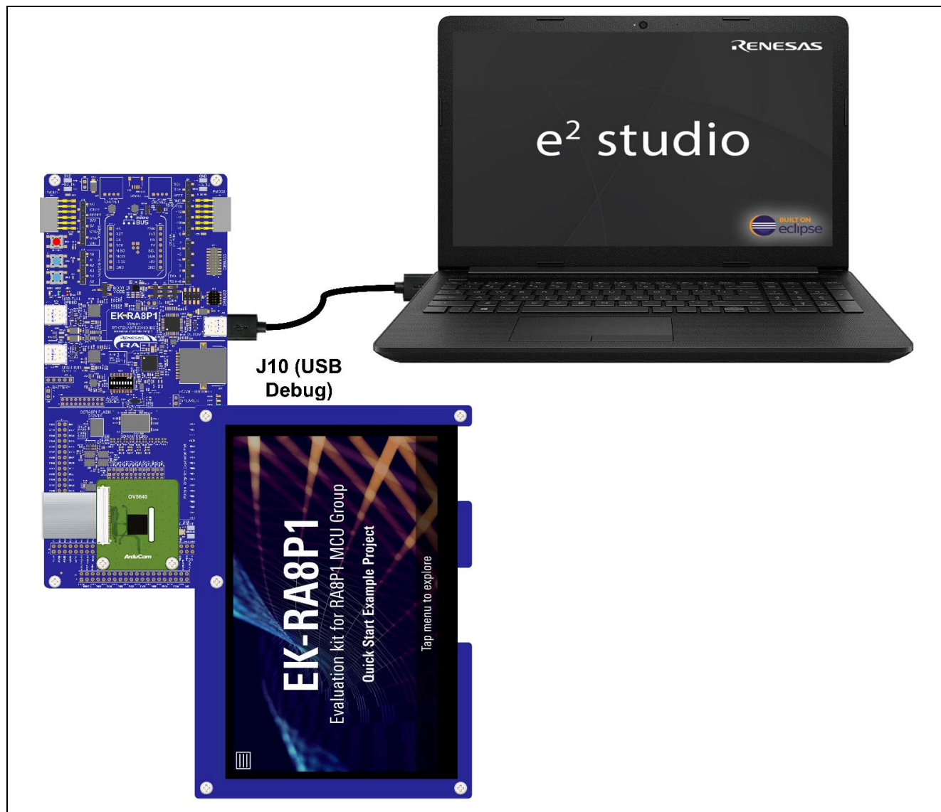
図 36. USB デバッグポート経由で EK-RA8P1 ボードとホスト PC の接続
