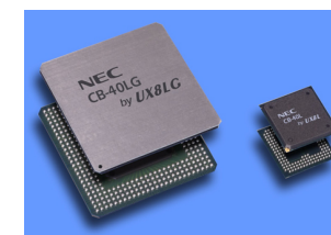
eDRAM対応40nmCBIC
