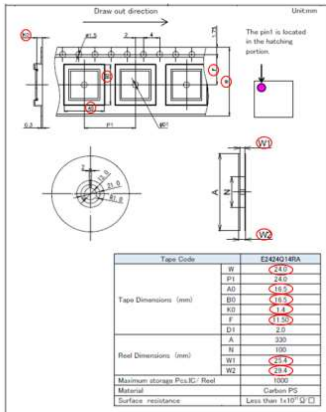
変更後 (W:24mm)
