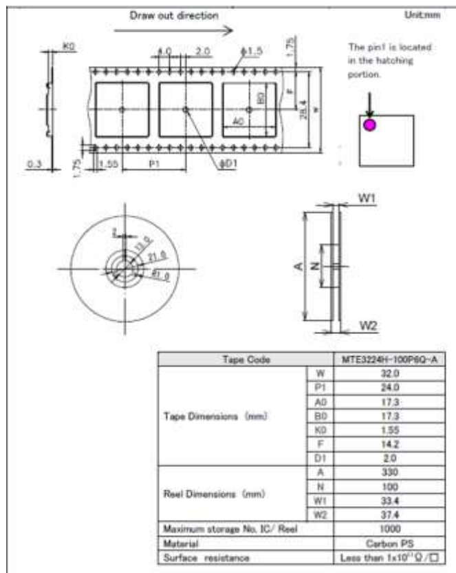
変更前 (W:32mm)
