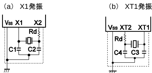
図 外付け発振回路例
