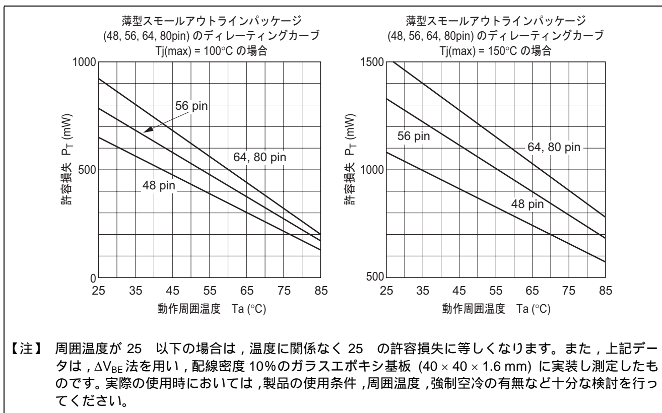
図 1 TSSOP のディレーティングカーブ
