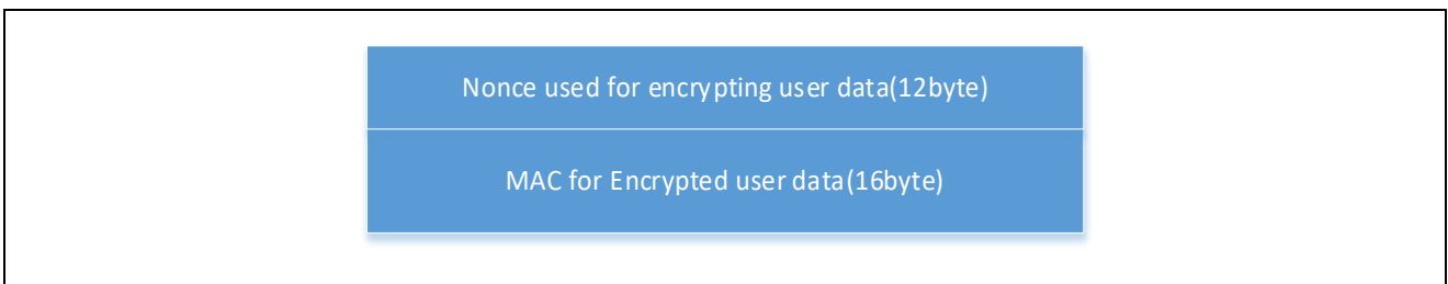
图 8-6 V2 格式 Nonce and MAC for encrypted user data Field
