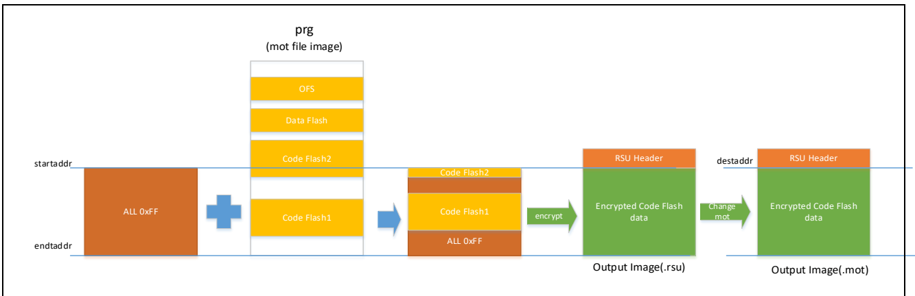
图 4-3 指定 ver 选项 1 时的加密流程
