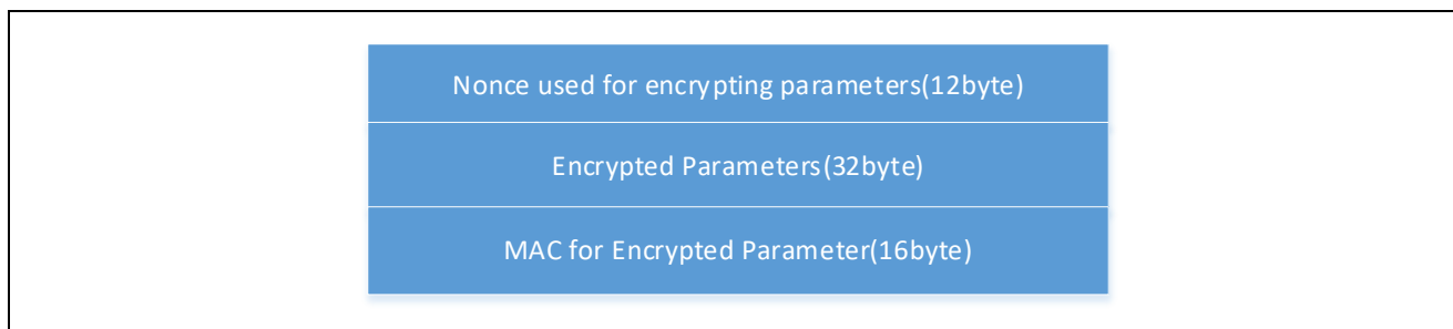
图 8-4 V2 格式 Parameter Field
