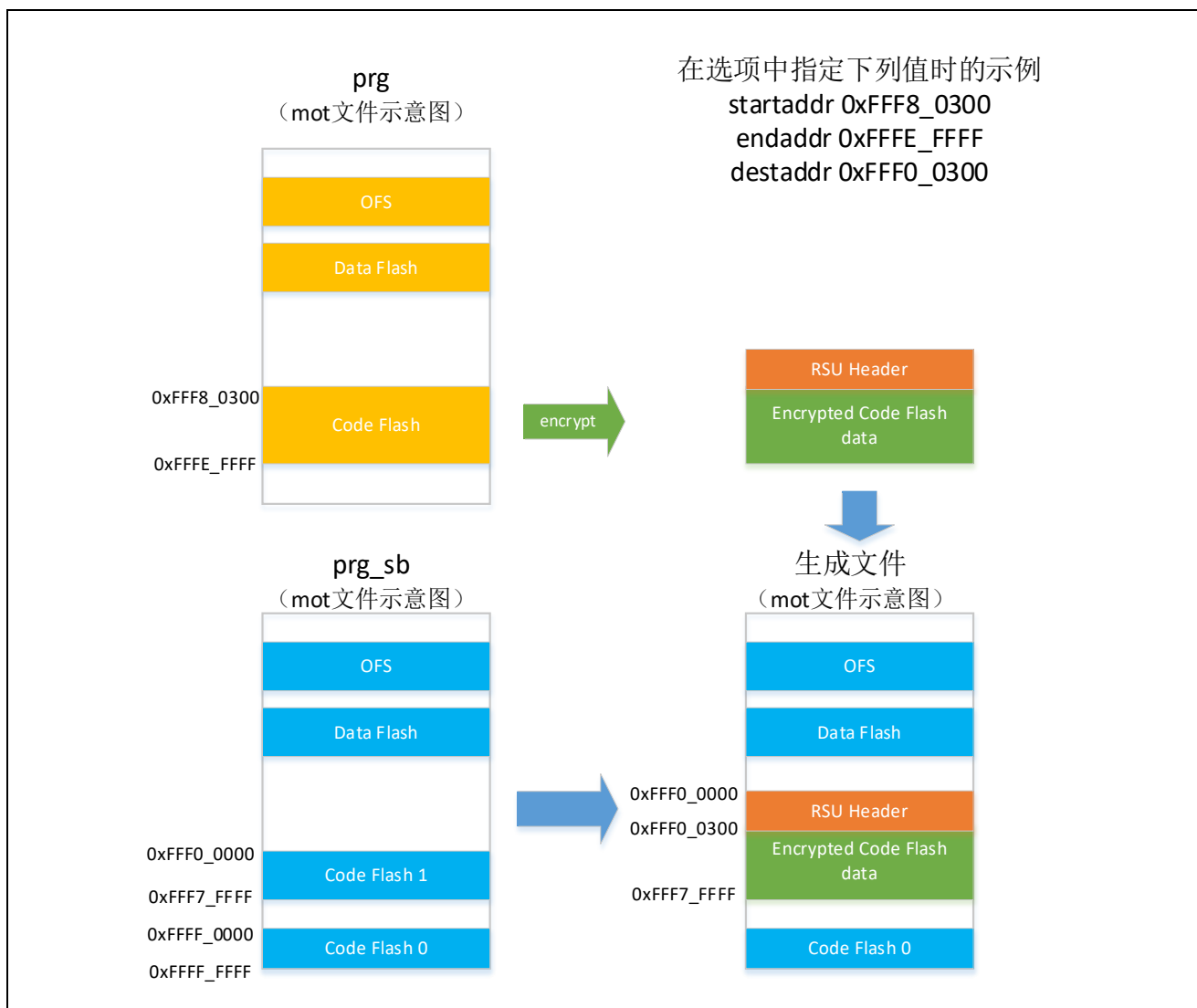
图 4-5 mode选项 指定factory时的文件生成示意图
