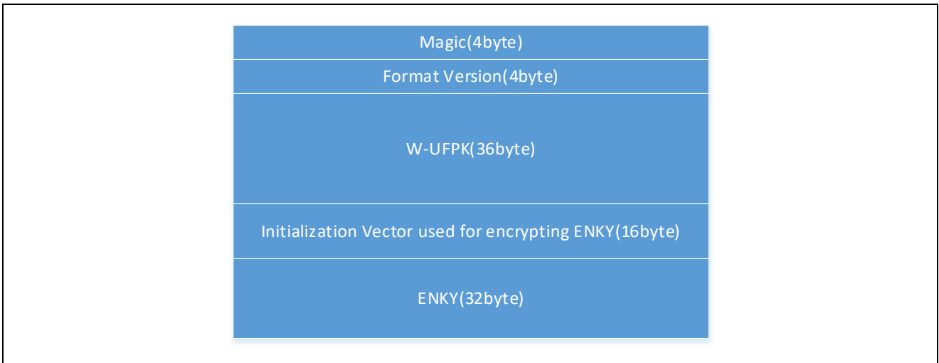
图 8-3 V2 格式 Header Field
