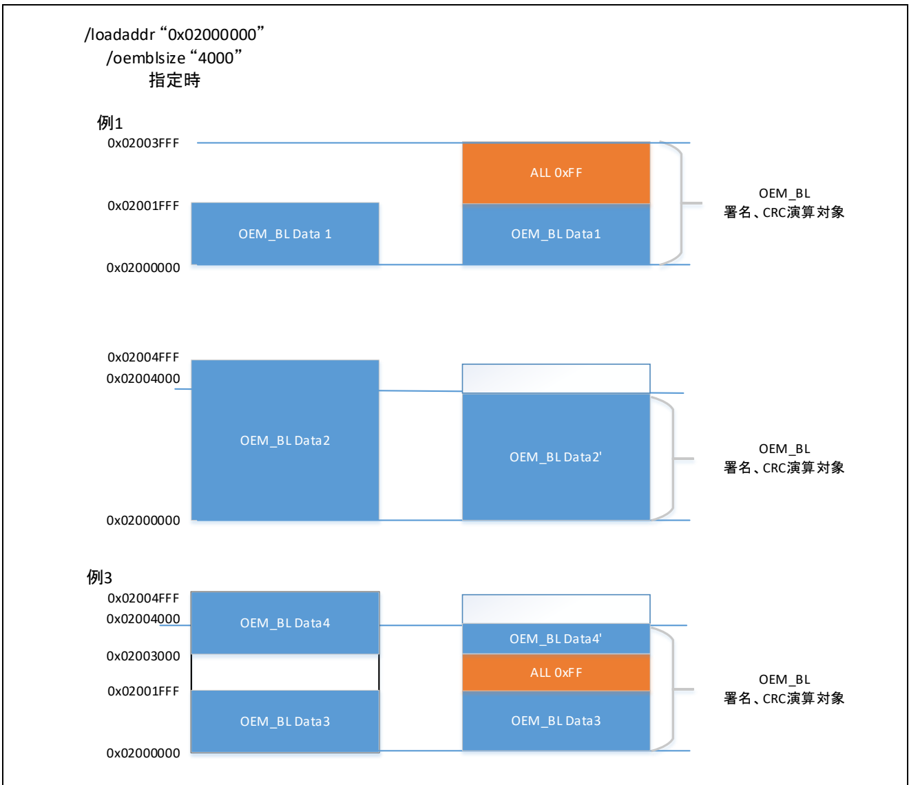
图 4-8 指定oembl_size选项时的签名、CRC运算对象
