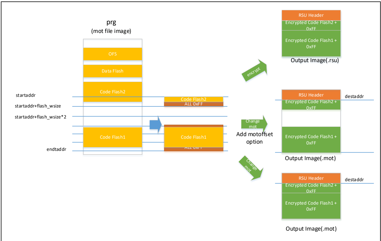
图 4-4 指定 ver 选项 2 时的加密流程
