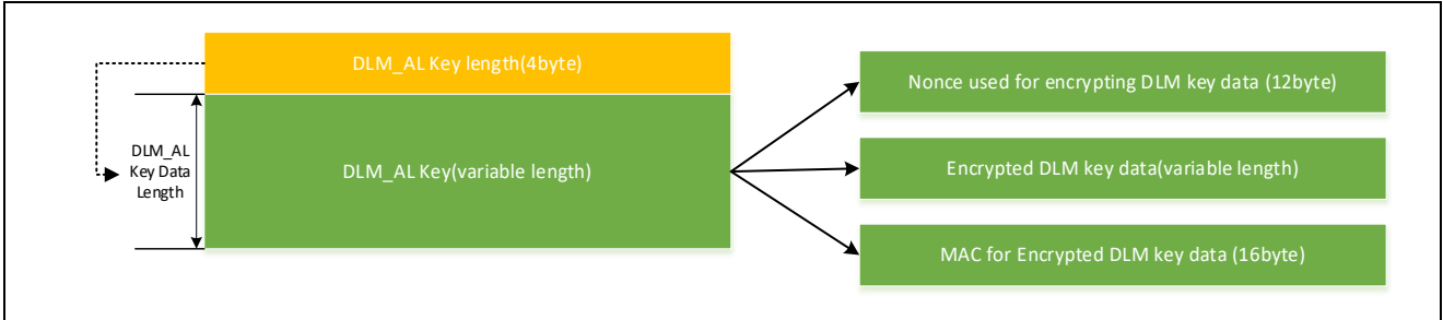
图 8-5 V2 格式 DLM_AL Key Field
