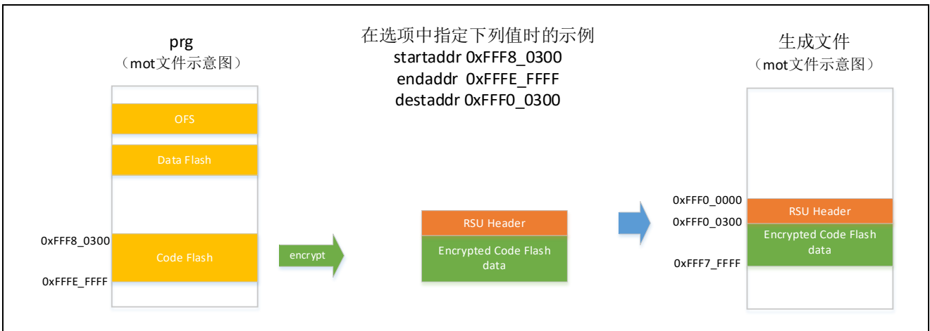
图 4-7 mode选项指定update且 filetype选项指定mot时的文件生成示意图
