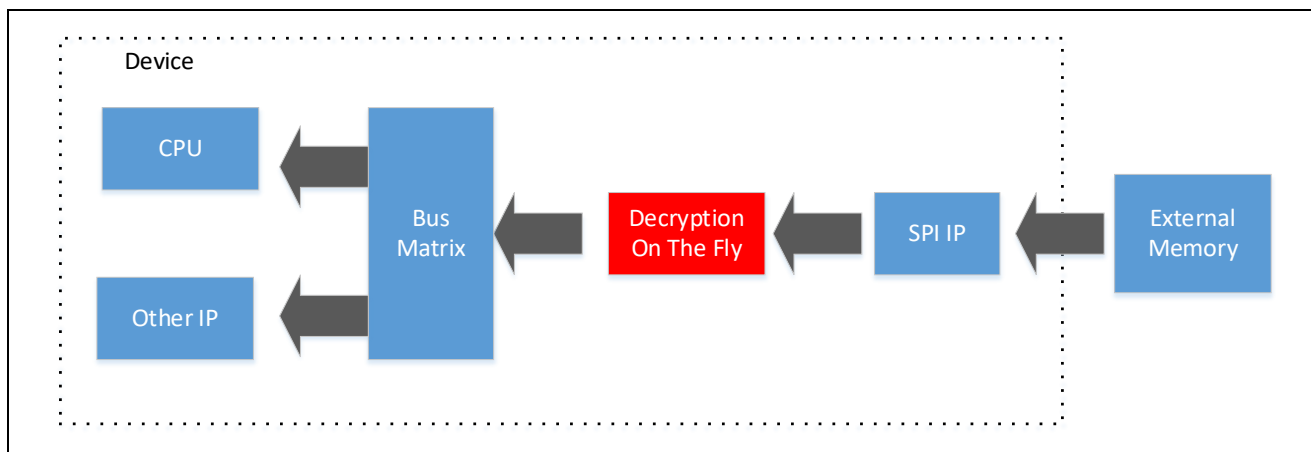
图 1-15 DOTF的MCU/MPU的内部系统总线示例
