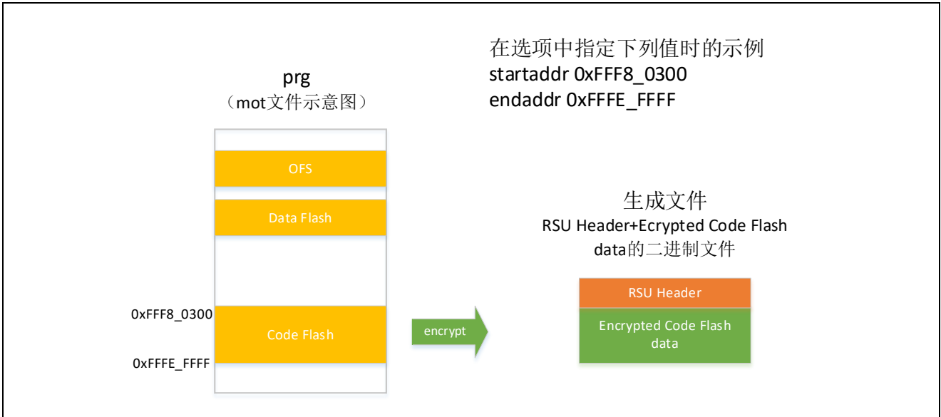
图 4-6 mode选项指定update且 filetype选项指定rsu时的文件生成示意图
