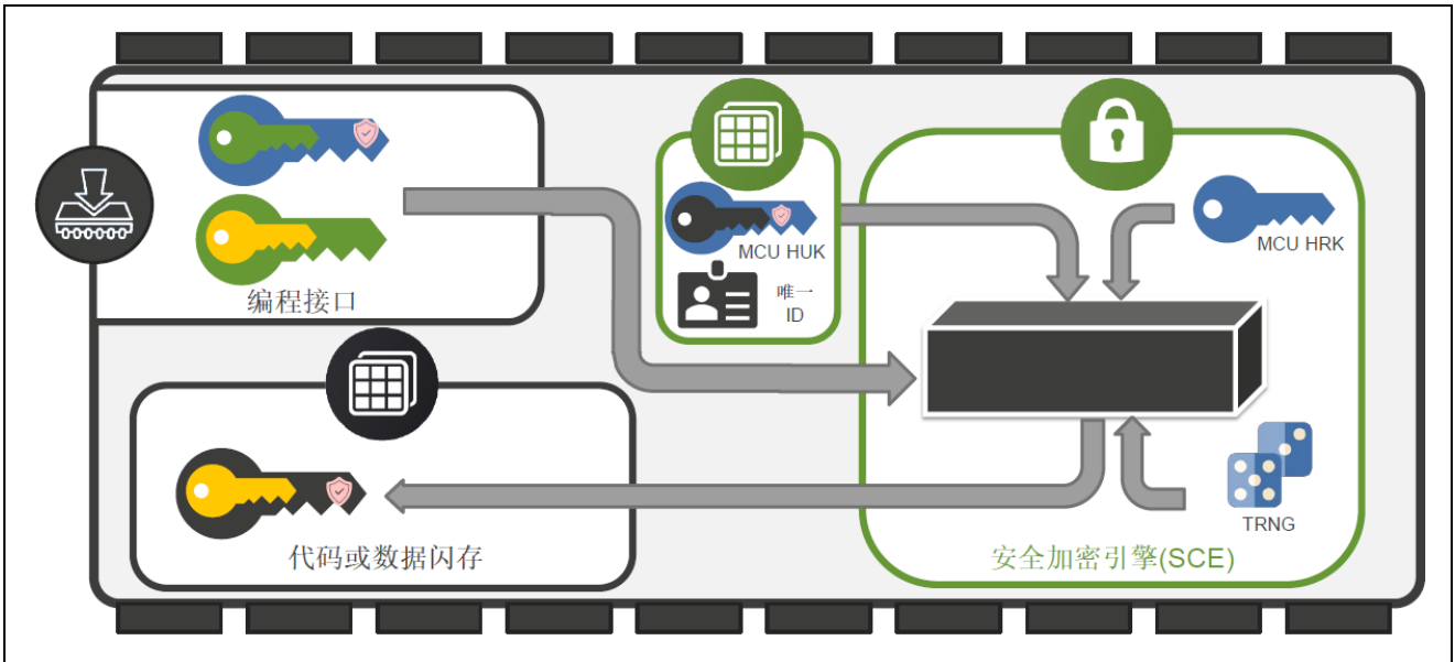
图 1-7 通过串行编程接口注入用户密钥
