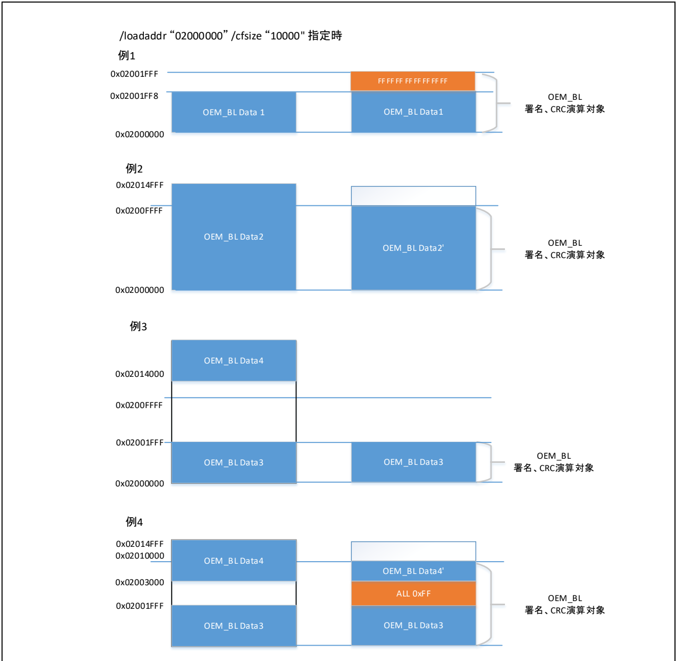
图 4-9 仅指定 cfsize 选项时的签名、 CRC 运算对象
