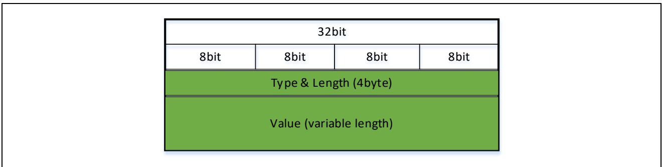
图 8-7 TLV格式
