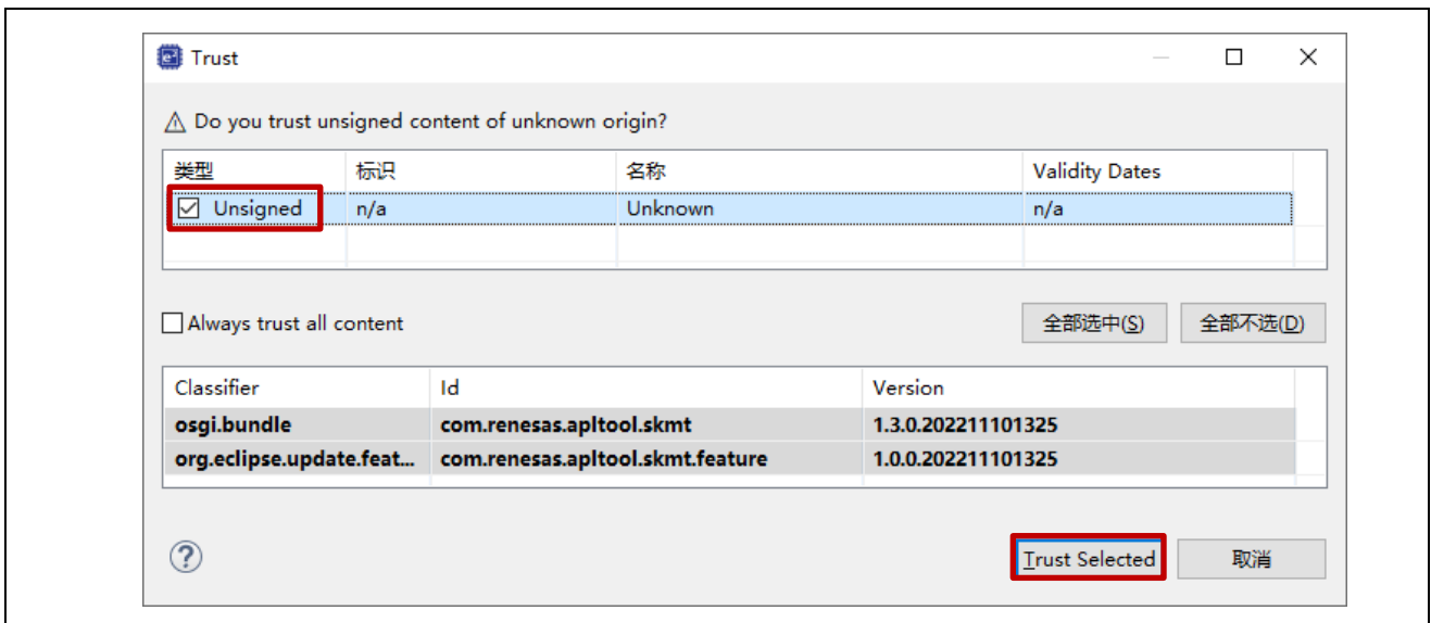
图 5-13 “信任”对话框
