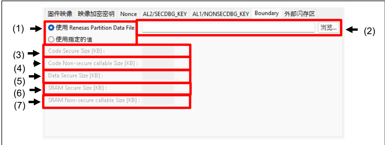
图 3-41 [Boundary]选项卡
