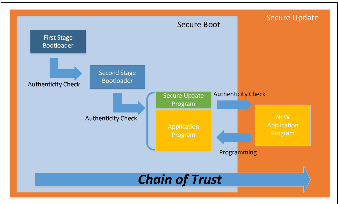
图 1-12 安全系统的Chain of Trust
