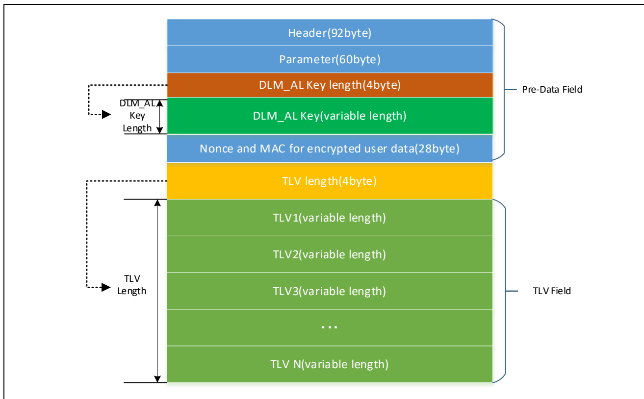
图 8-2 V2格式图像图
