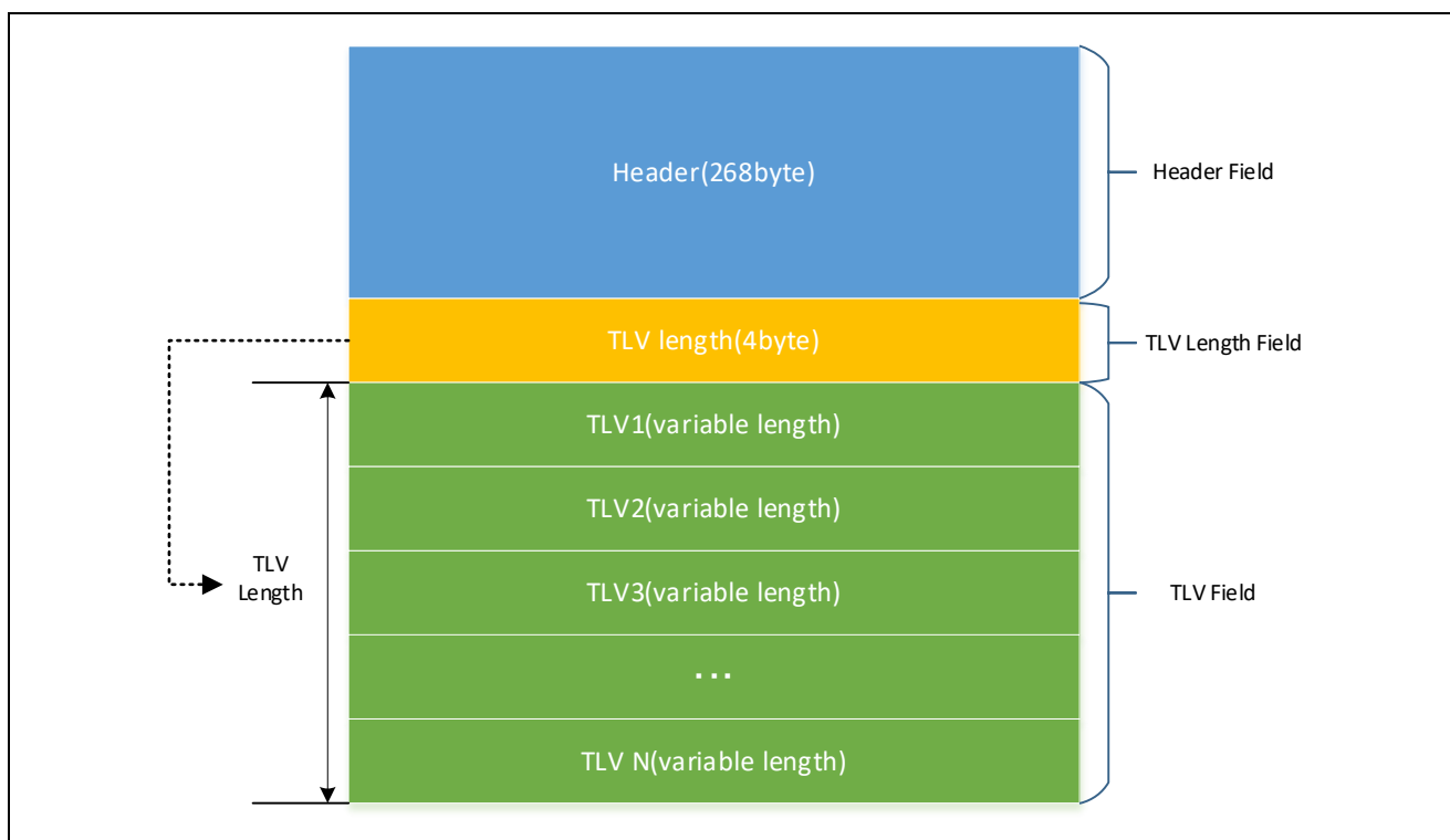
图 8-1 V1格式图像图
