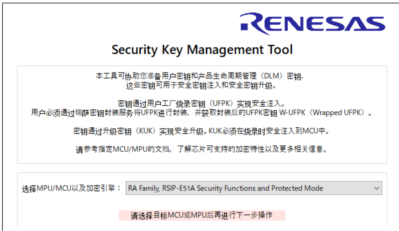
图 6-44 [概要]选项卡
