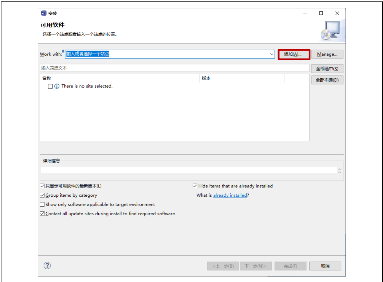
图 5-8 “安装”对话框
