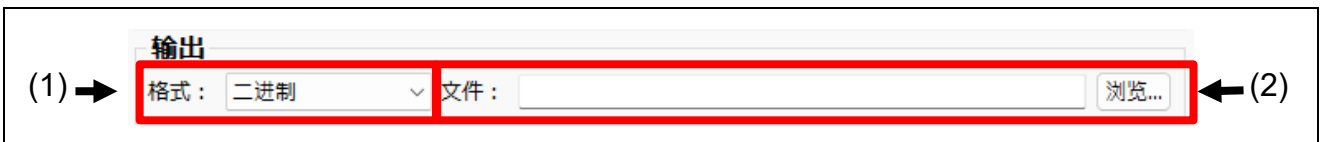
图 3-23 输出
