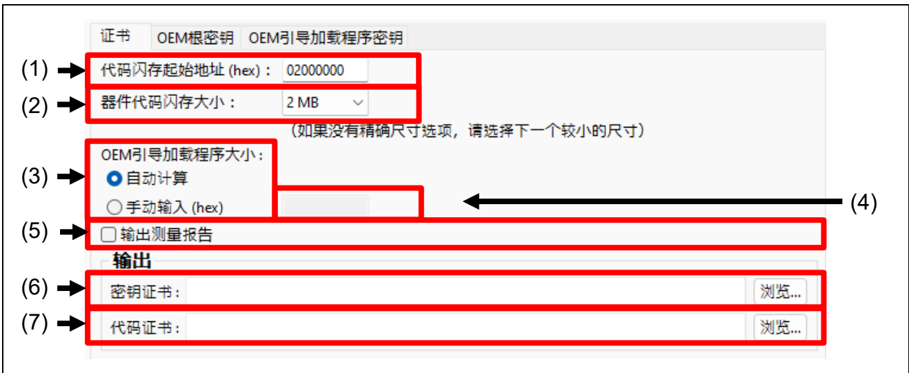
图 3-26 [证书]选项卡
