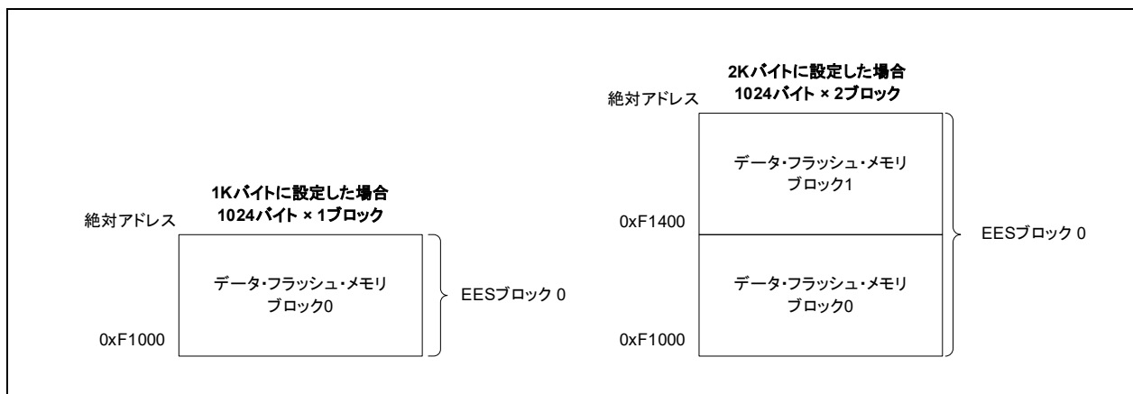
図 2-2 EES ブロック 0 の概念図
