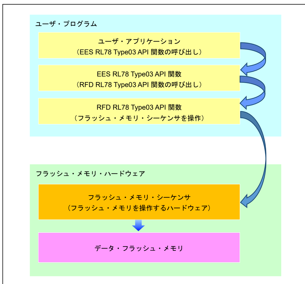
図 1-1 EES RL78 Type03 の API 関数を使ったデータ・フラッシュ・メモリの操作イメージ
