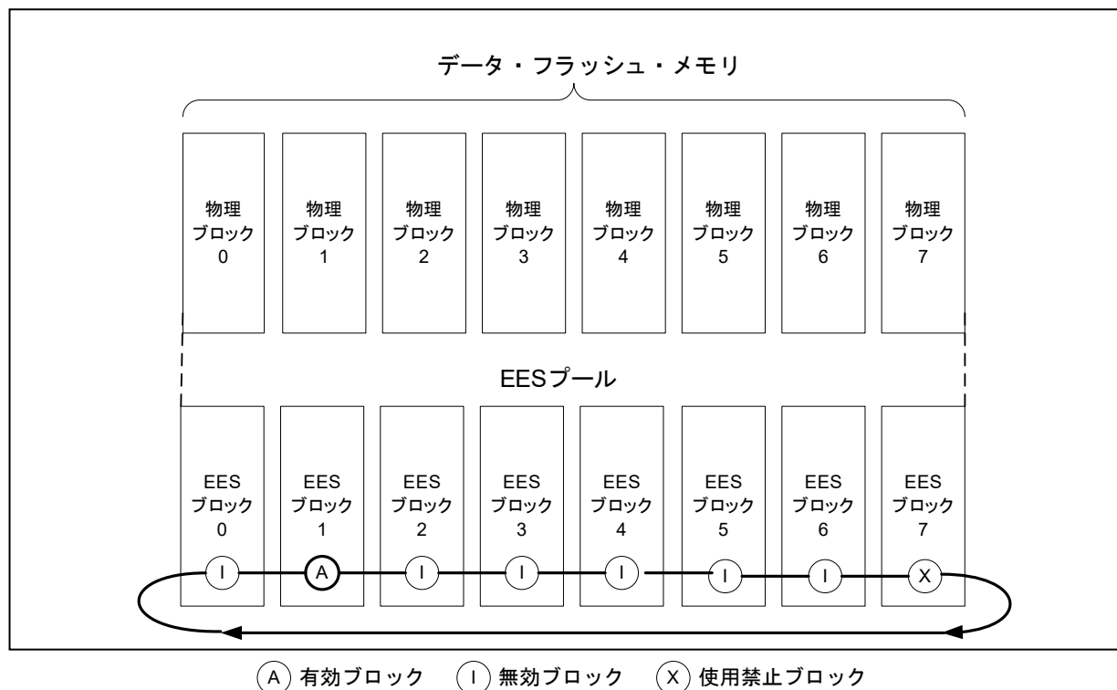
図 3-1 EES プール状態例 (EES ブロックに1K バイト設定時)
