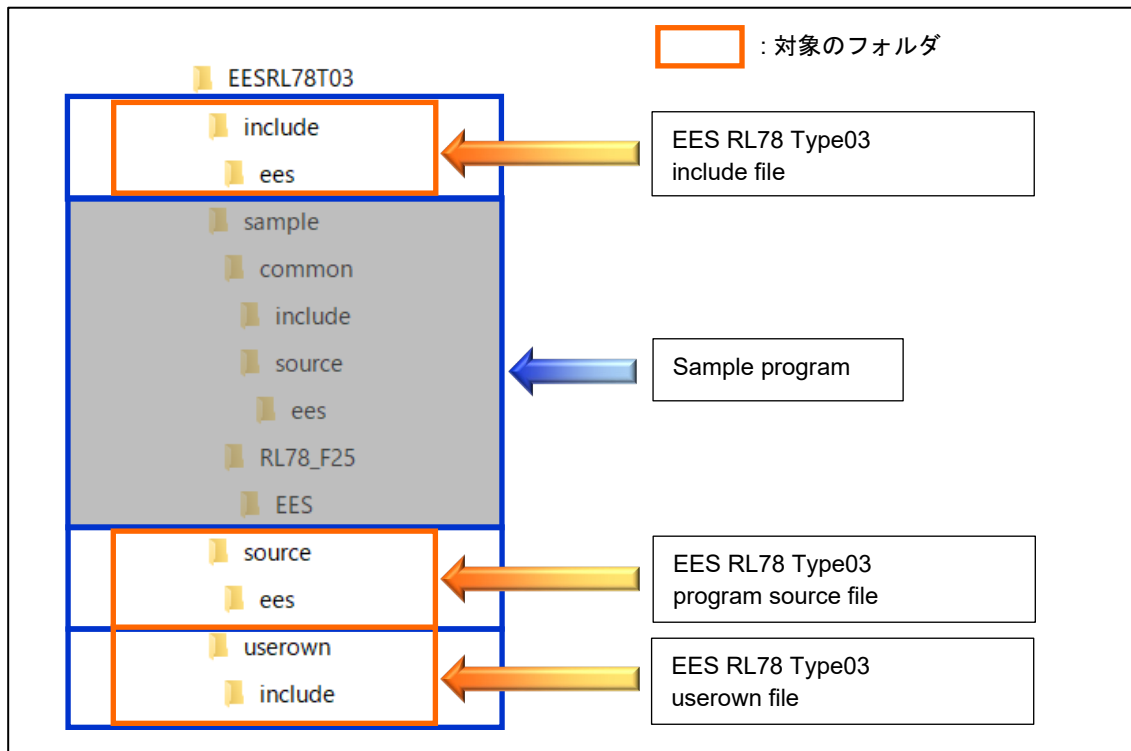
図 2-4 EES RL78 Type03 のフォルダ構成
