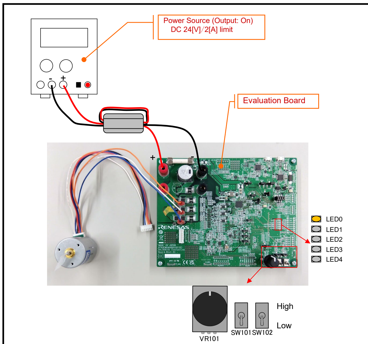
Figure 3-15 モータ駆動停止
