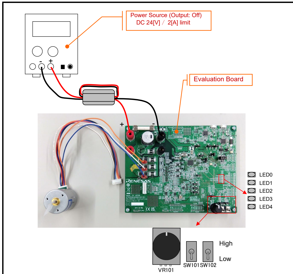
Figure 3-12 初期設定
