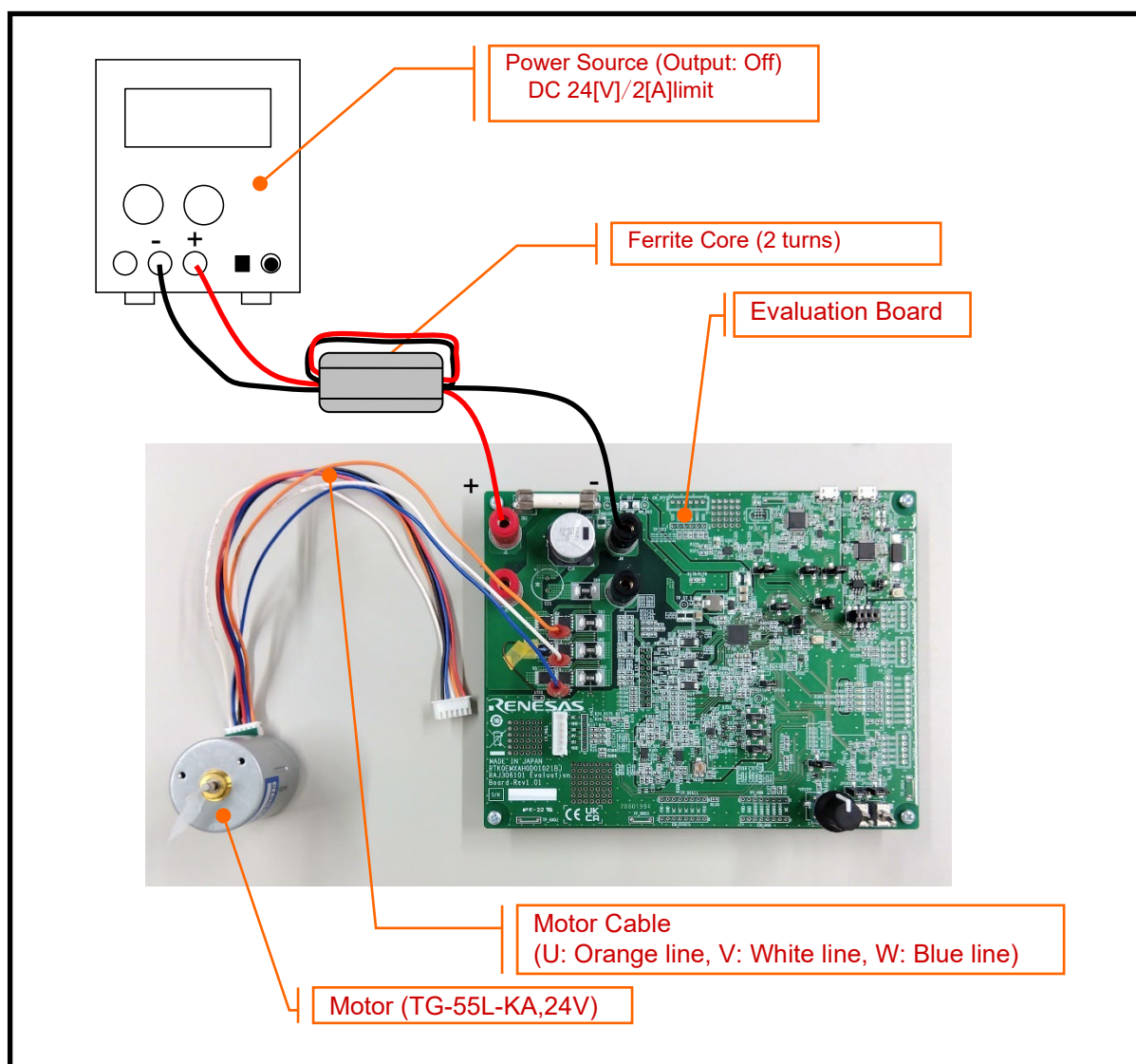
Figure 3-11 接続
