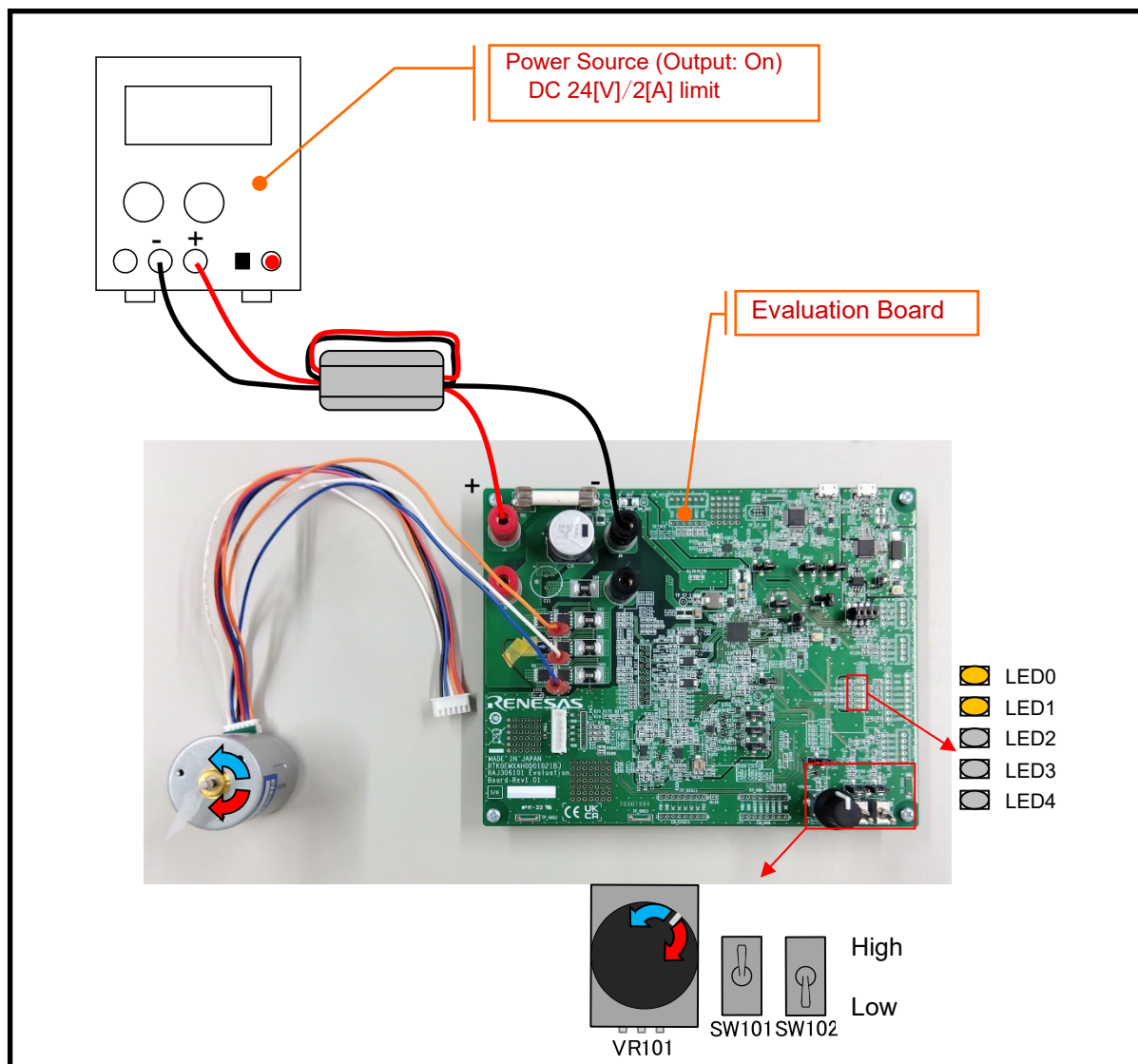
Figure 3-7 モータ駆動
