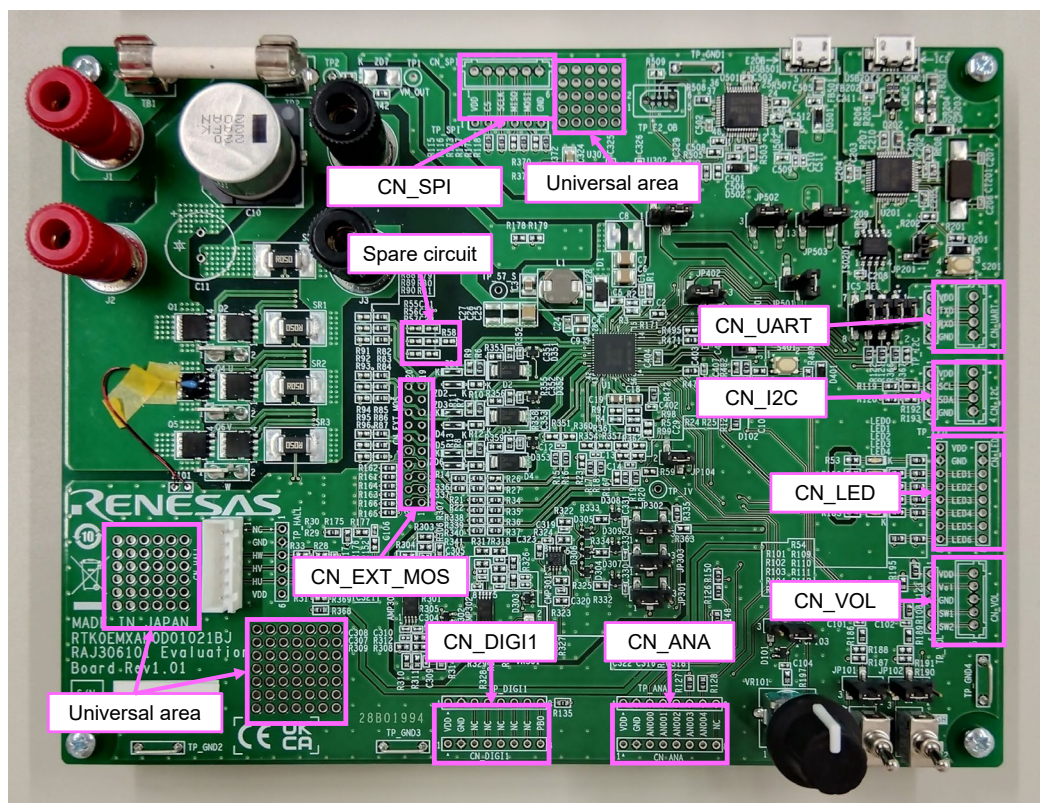
Figure 2-4 未実装のコネクタや回路
