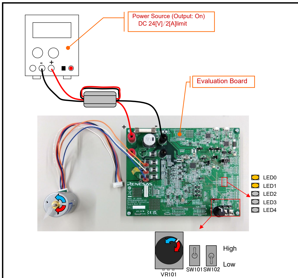
Figure 3-14 モータ駆動
