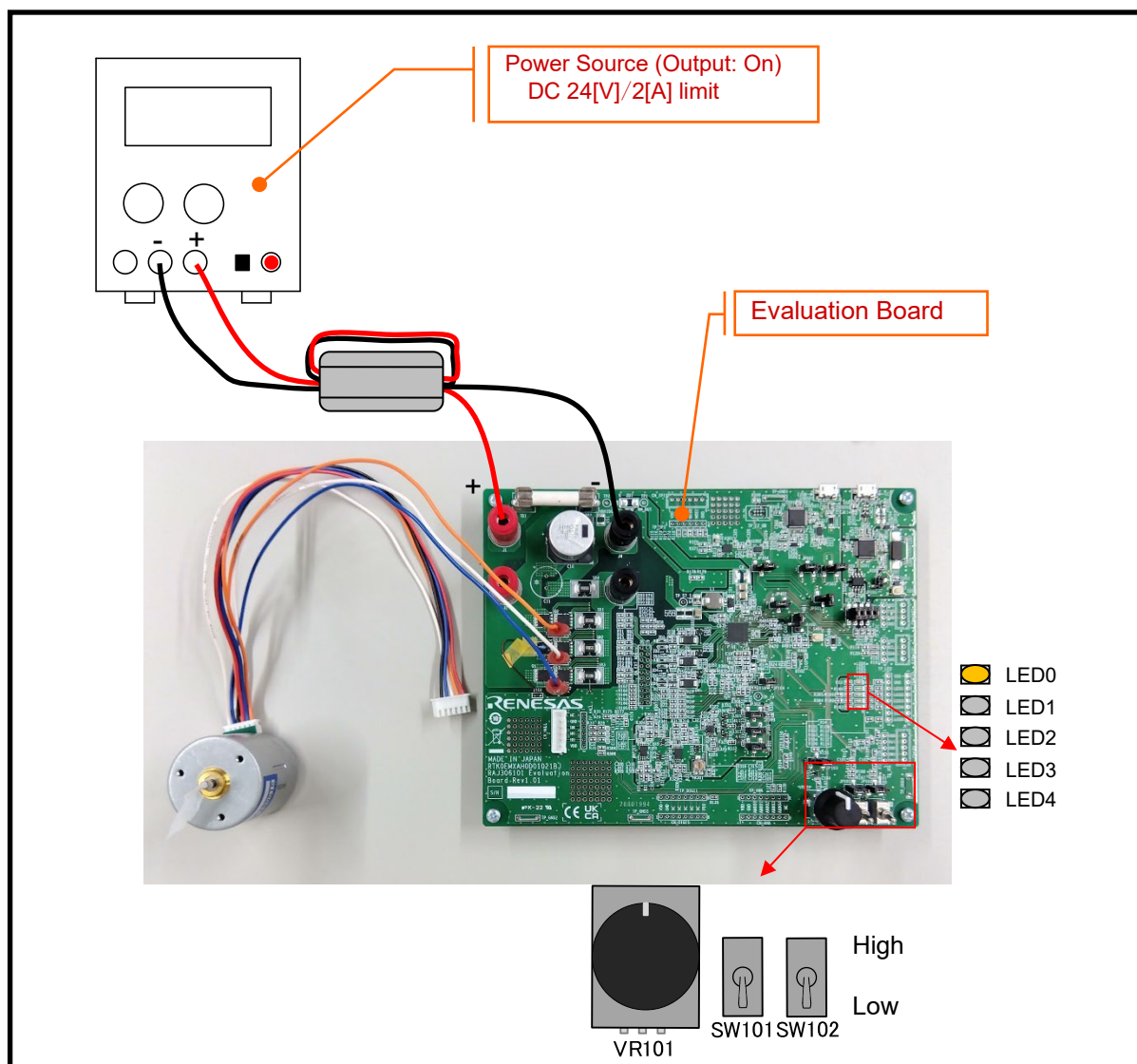
Figure 3-8 モータ駆動停止
