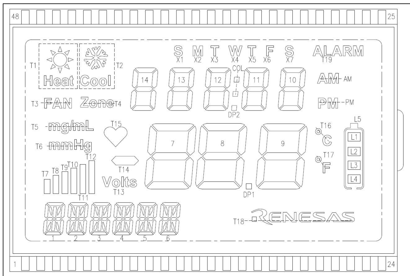
図 5. セグメント LCD ピンエリア割り当て
