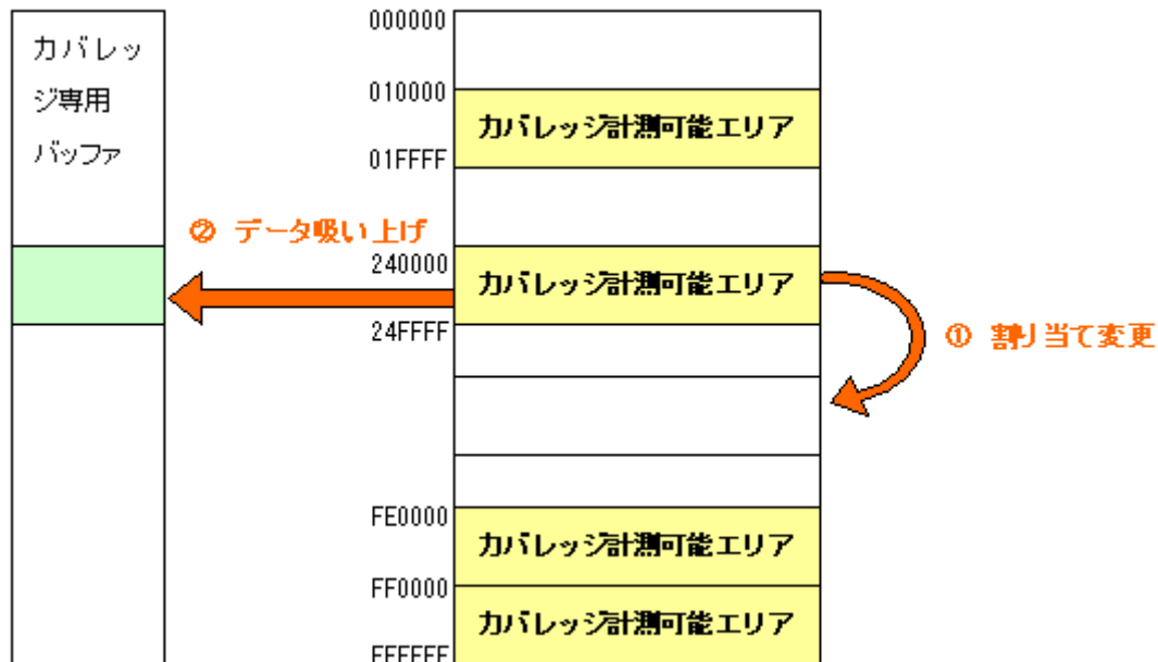
図 5.108 [データカバレッジメモリ] の割り当て変更概略図
