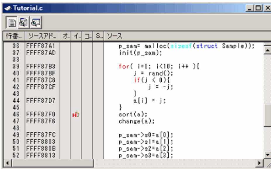
図3.28 [エディタ]ウィンドウ（ハードウェアブ레이크ポイントの設定）
