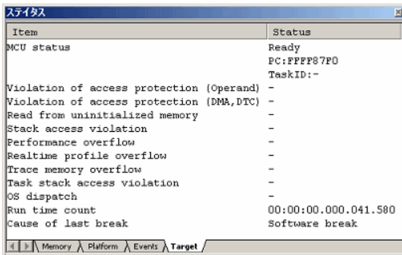
図3.7 [ステイタス]ウィンドウ
