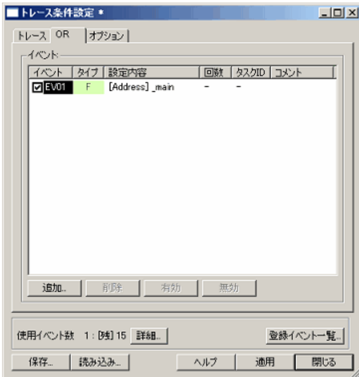
図3.36 [トレース条件設定]ダイアログボックス (ORページ)
