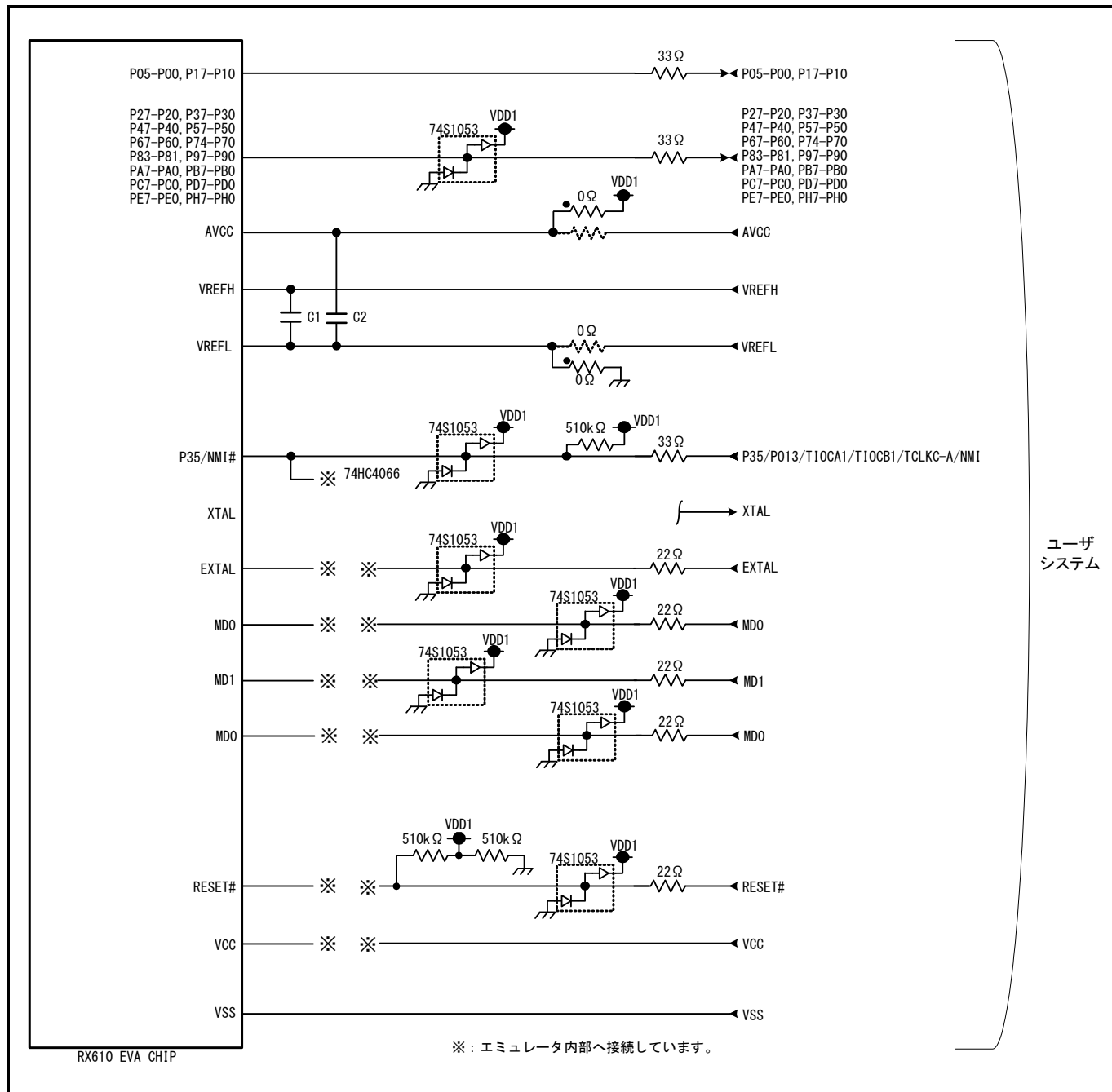
図 7.1 ROE556100MCU00の接続図(一部)
