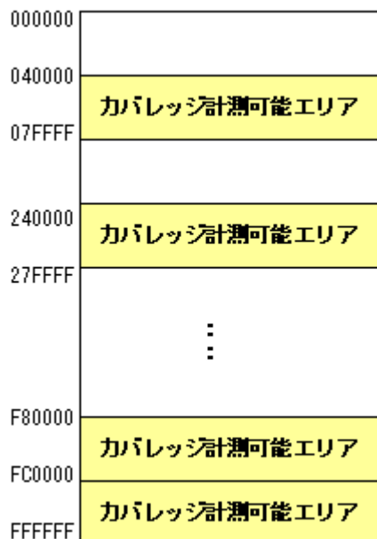
図 5.76 [コードカバレッジメモリ] の割り当て概略図
