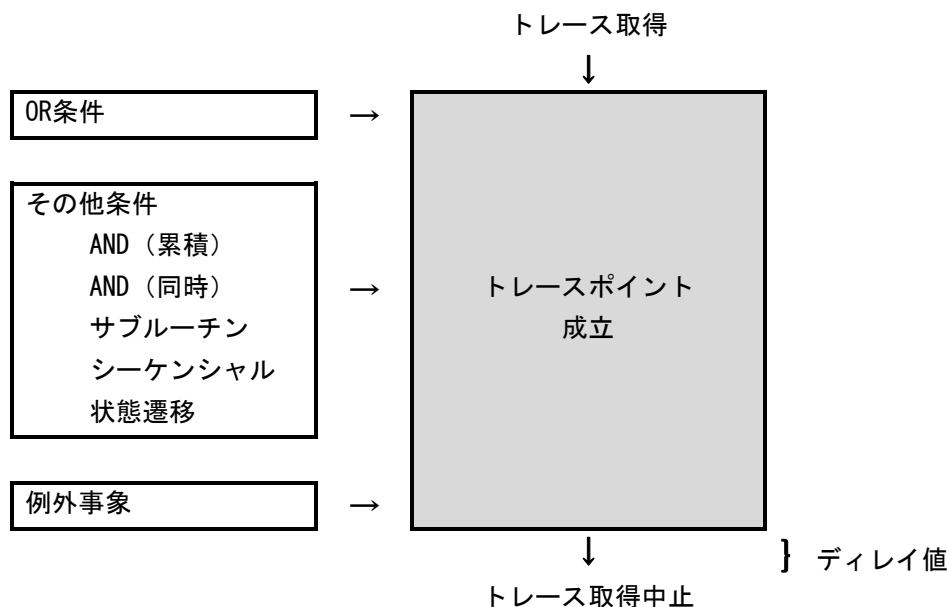
図 5.53 トレースポイント概要
