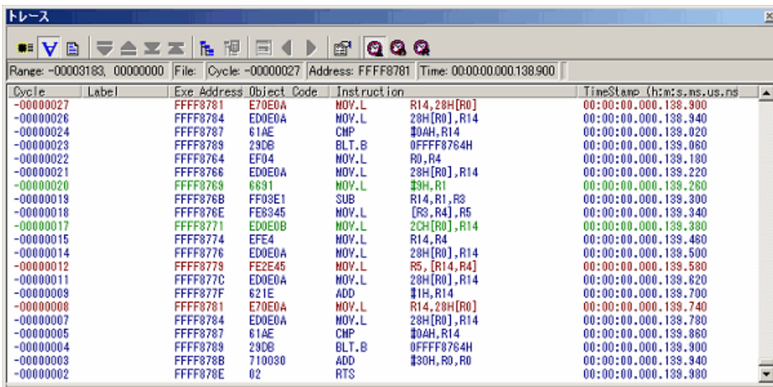
図 5.60 [トレース] ウィンドウ
