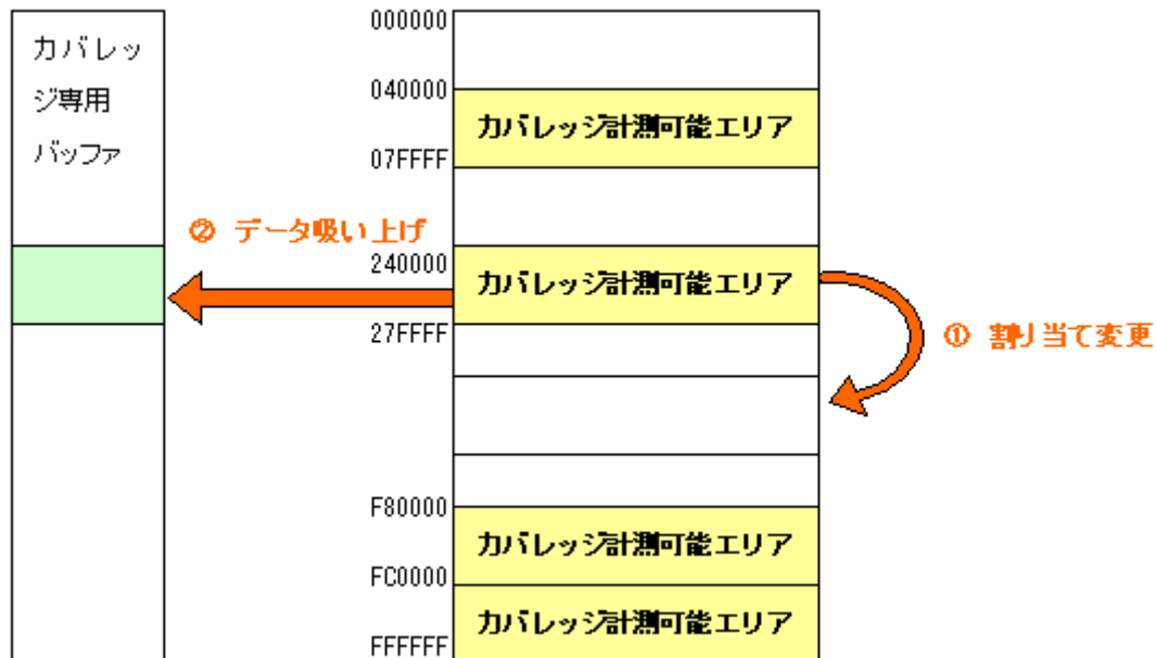
図 5.77 [コードカバレッジメモリ] の割り当て変更概略図
