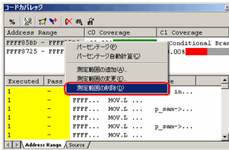
図 5.85 [コードカバレッジ] ウィンドウ
