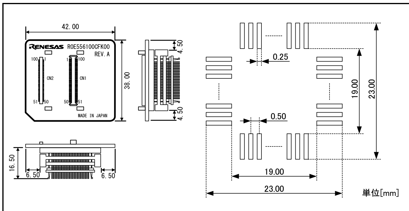
図7.3 R0E556100CFK00ユーザーシステム接続部の寸法図および参考フットパターン
