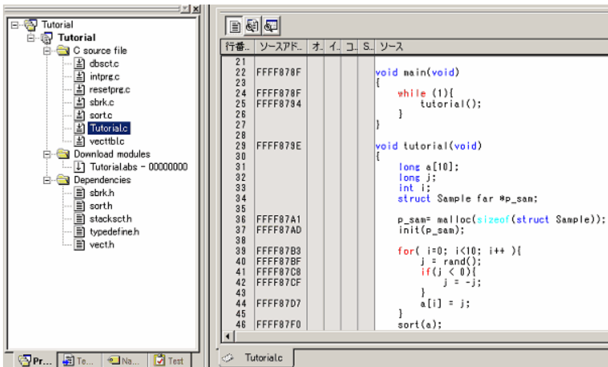
図3.4 [エディタ]ウィンドウ (ソースプログラムの表示)
