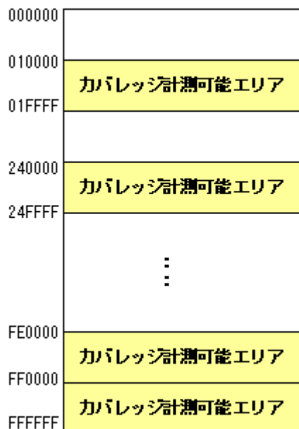
図 5.107 [データカバレッジメモリ] の割り当て概略図
