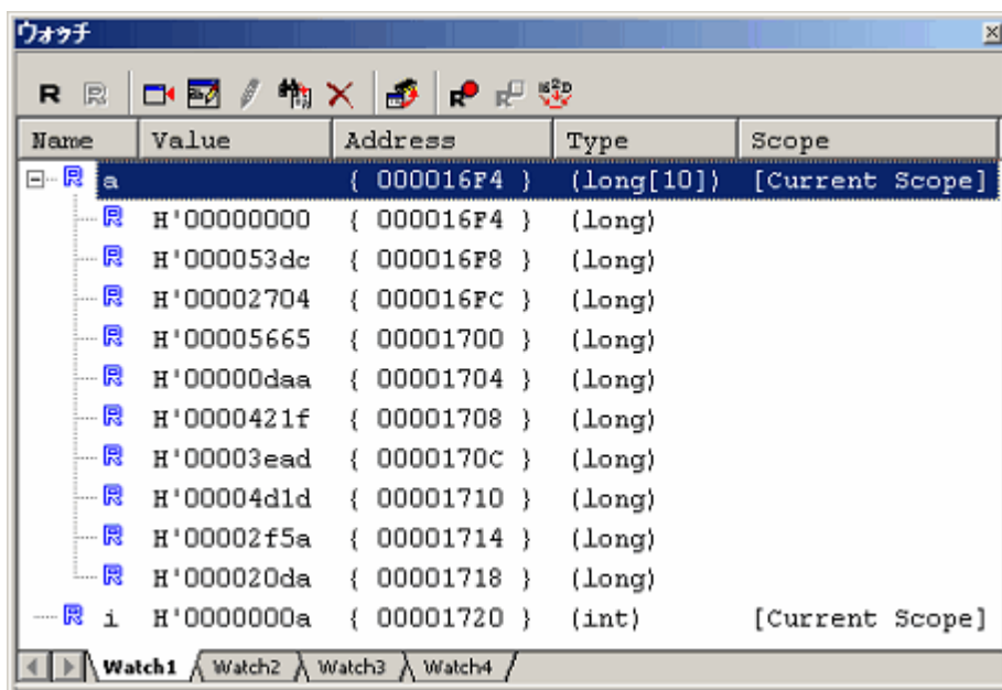
図3.18 [ウォッチ]ウィンドウ (配列要素の表示)
