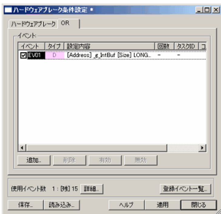
図3.29 [ハードウェアブレイク条件設定]ダイアログボックス
