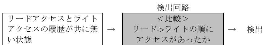
図 5.147 初期化抜け検出方法の概要
