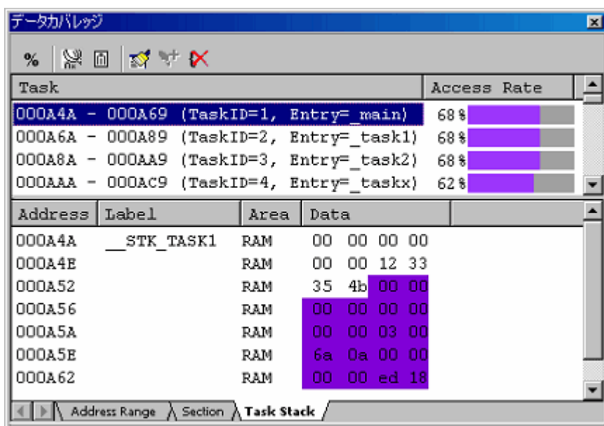
図 5.126 [データカバレッジ] ウィンドウ (タスクスタック指定)
