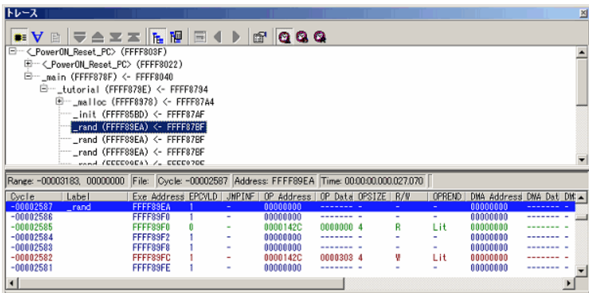
図3.40 [トレース]ウィンドウ (関数実行履歴)
