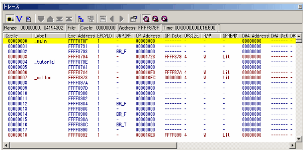
図3.37 [トレース]ウィンドウ (ポイント&ディレイ)
