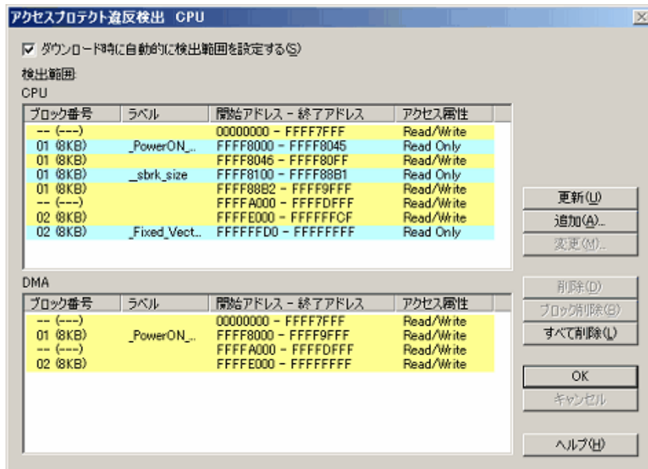
図 5.142 [アクセスプロテクト違反検出] ダイアログボックス
