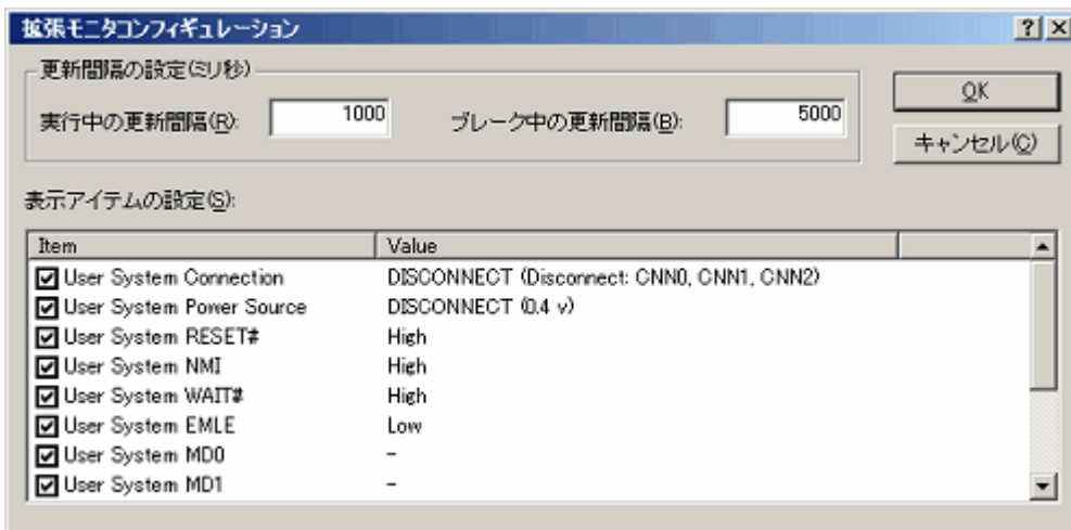
図 5.21 [拡張モニタコンフィギュレーション] ダイアログボックス
