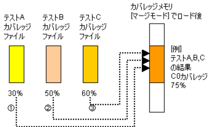
図 5.103 [マージ] モードの応用例時の動作概略
