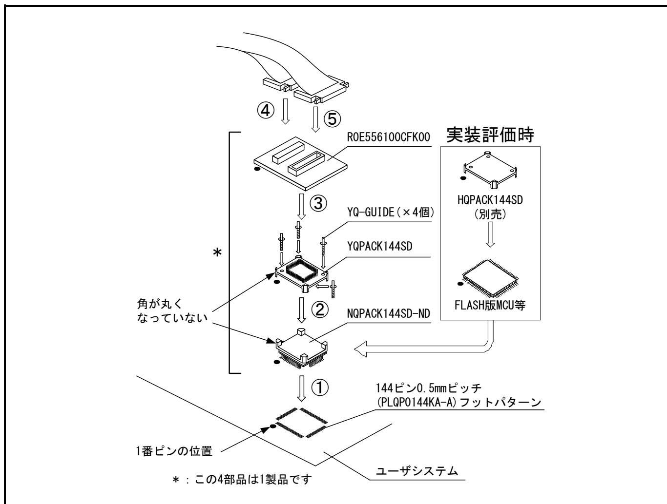
図2.11 144ピン0.5mmピッチフットパターンへの接続
