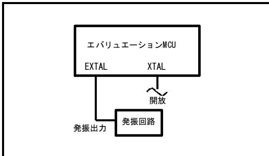
図2.8 ユーザシステム上発振回路の使用
