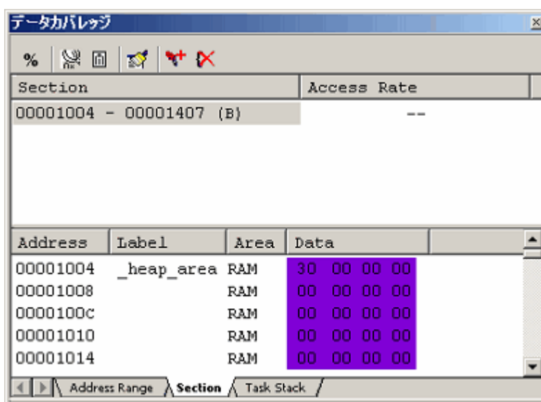
図 5.122 [データカバレッジ] ウィンドウ
