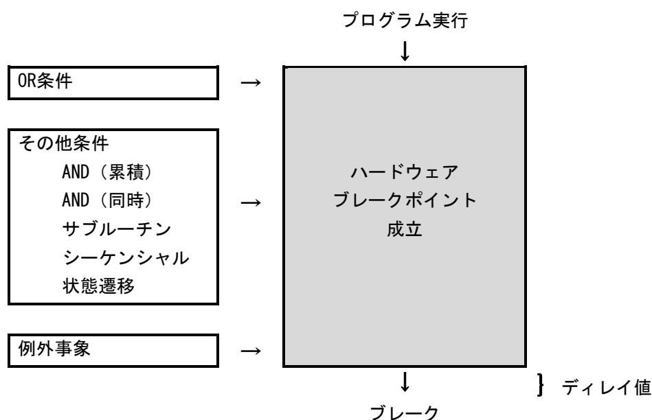
図 5.45 ハードウェアブレイク概要
