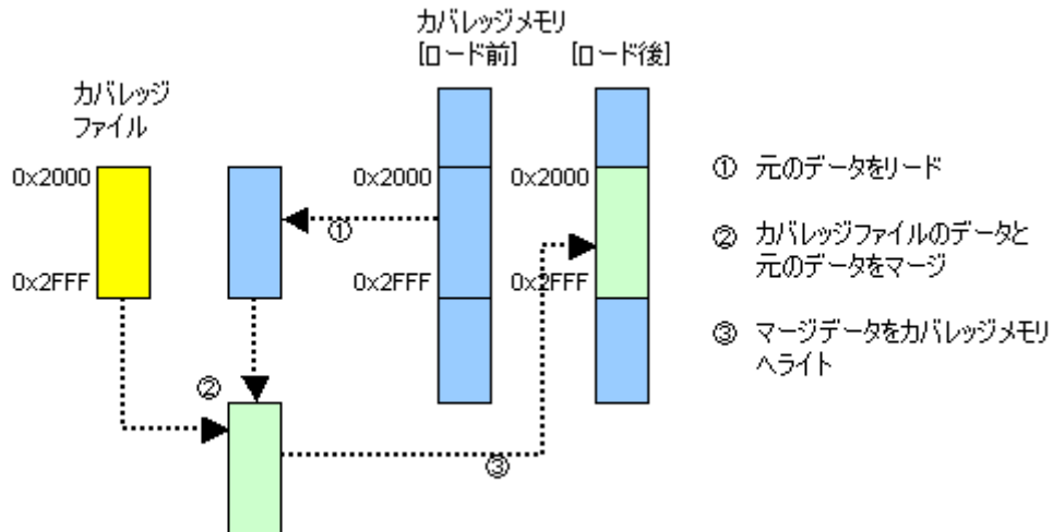
図 5.102 [マージ] 選択時のロードモード動作概略
