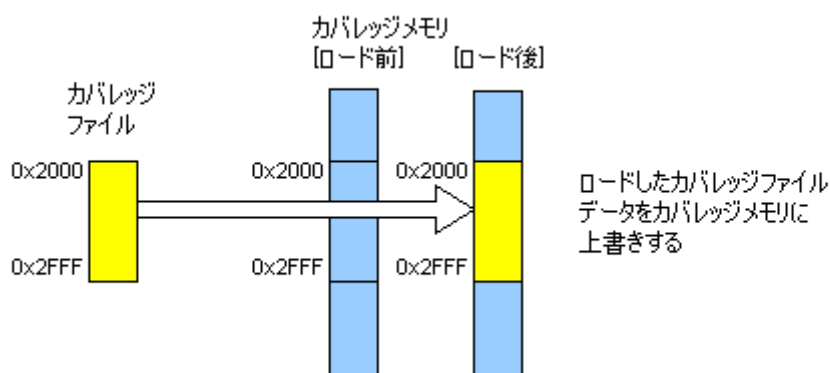
図 5.101 [上書き] 選択時のロードモード動作概略
