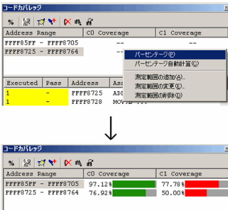
図 5.95 [コードカバレッジ] ウィンドウ
