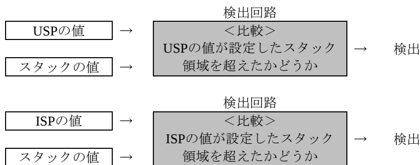
図5.146 スタックアクセス違反検出方法の概要
