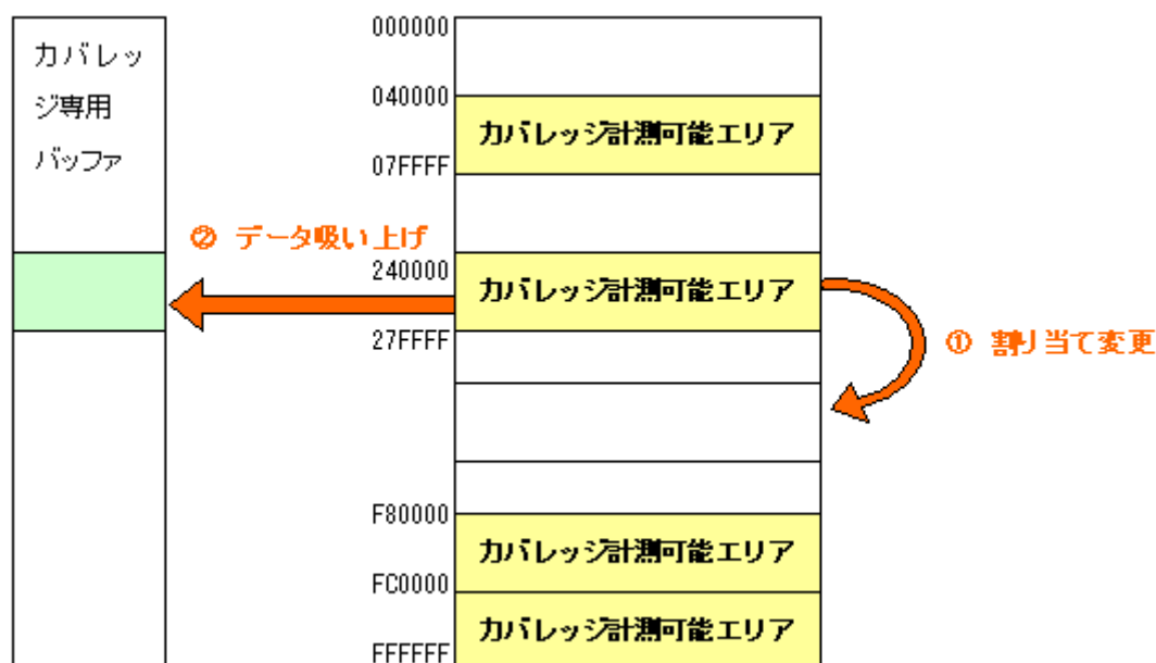
図5.75 「コードカバレッジメモリ」の割り当て変更概略図
