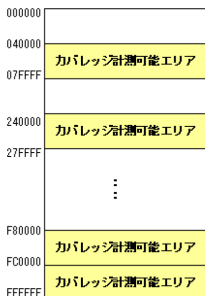
図5.74 「コードカバレッジメモリ」の割り当て概略図
