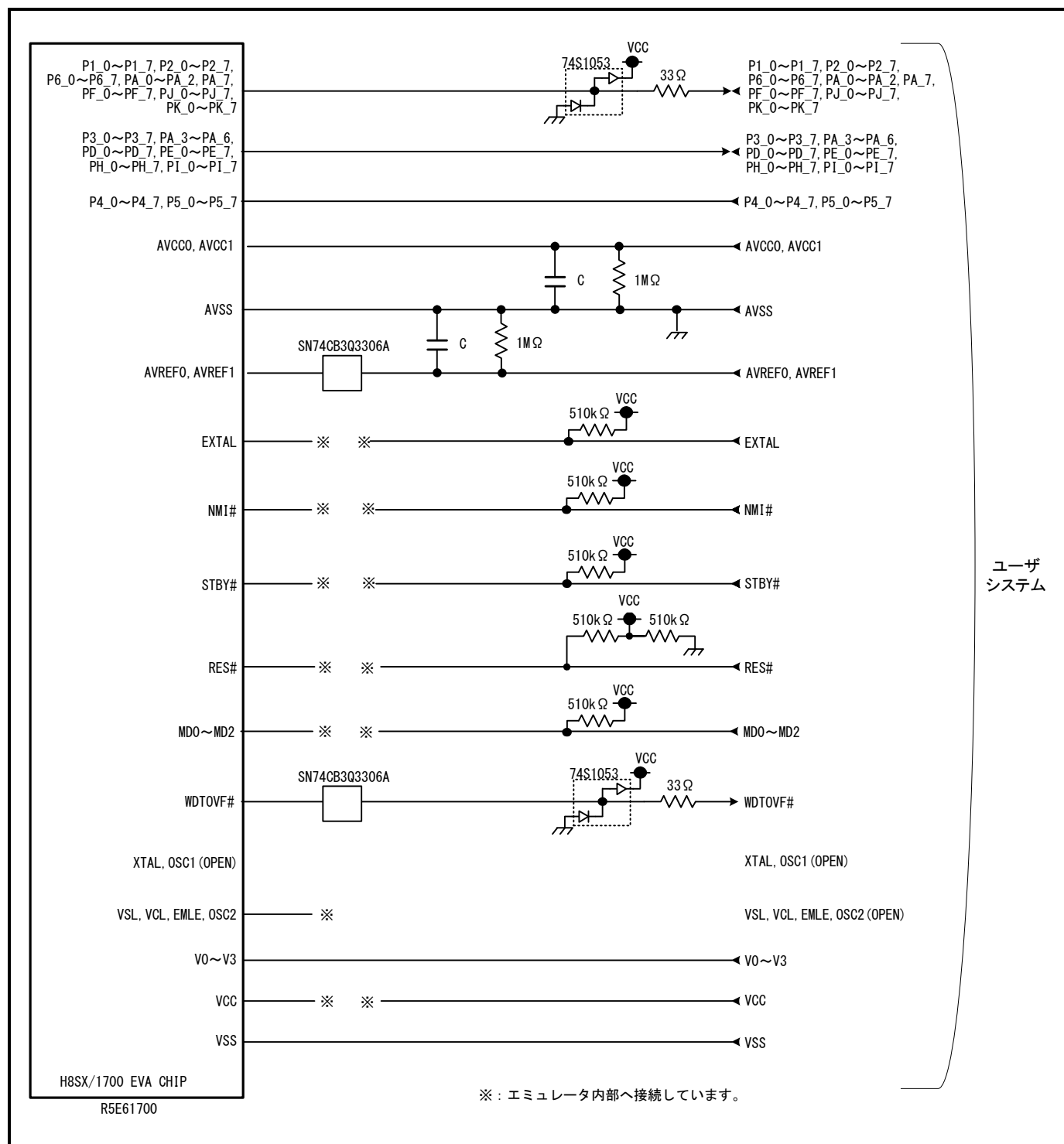
図 7.1 R0E417250MCU00の接続図(一部)
