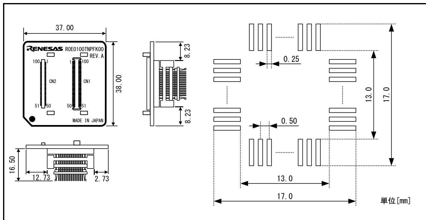
図 7.3 R0E0100TNPFK00ユーザシステム接続部の寸法図および参考フットパターン
