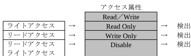
図 5.107 検出方法のNGパターン
