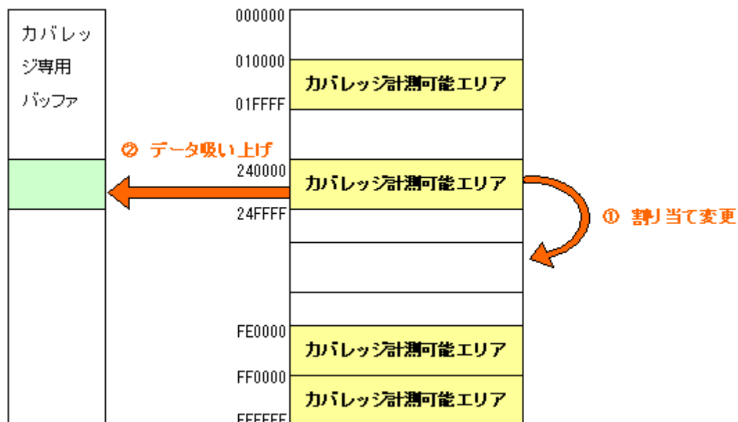
図 5.91 【データカバレッジメモリ】の割り当て変更概略図
