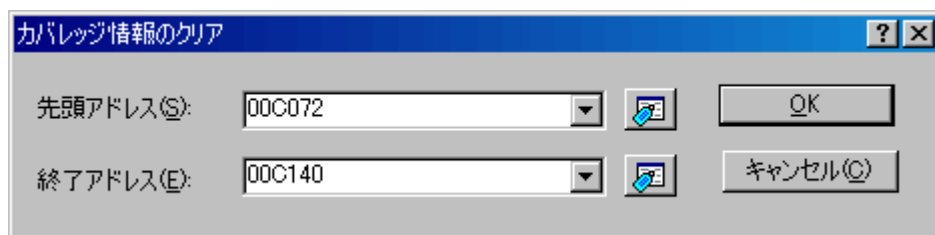
図 5.80 [カバレッジ情報のクリア] ダイアログボックス
