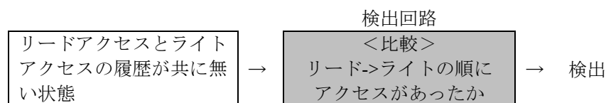
図 5.115 初期化抜け検出方法の概要
