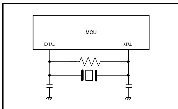
図2.9 エミュレータでは使用できない発振回路
