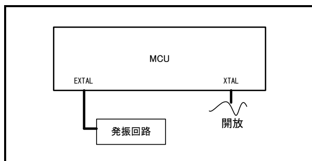
図2.8 ユーザシステム上発振回路の使用
