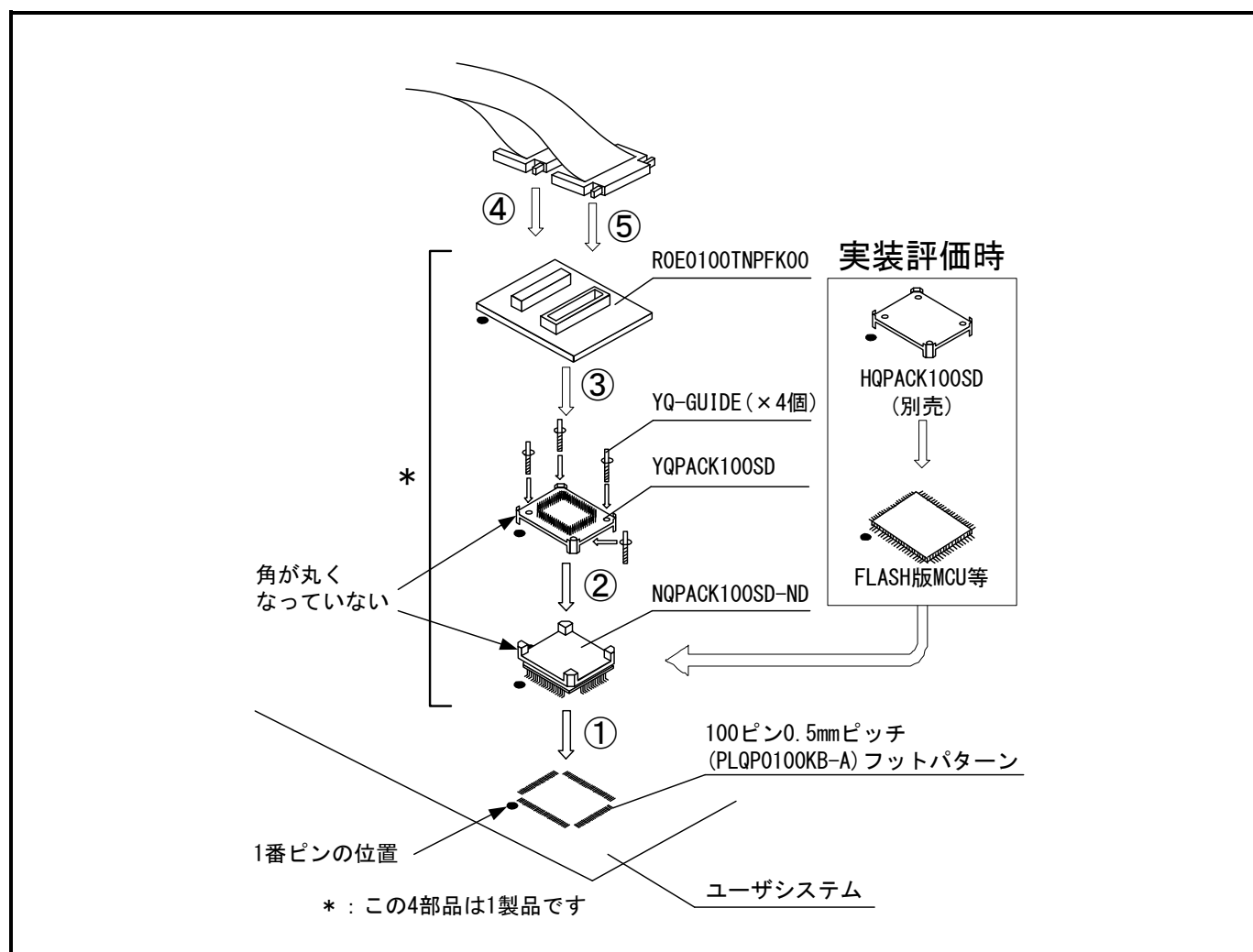
図2.11 100ピン0.5mmピッチフットパターンへの接続
