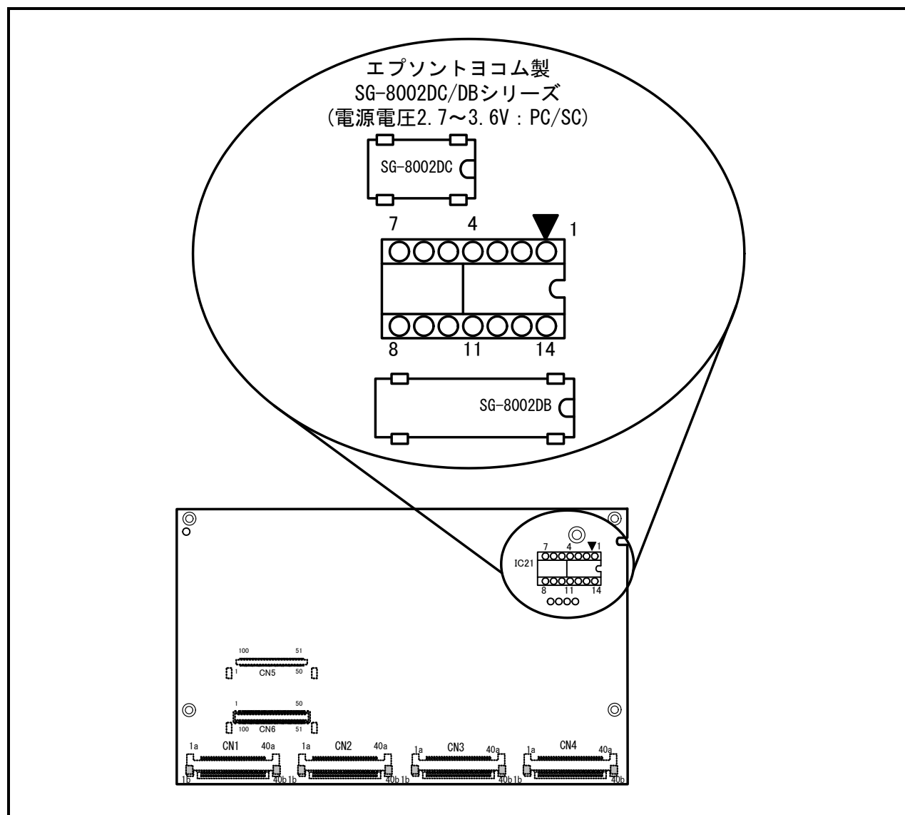
図2.7 発振モジュール交換
