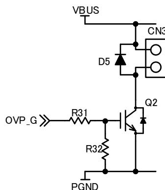
図 4-4 過電圧保護
