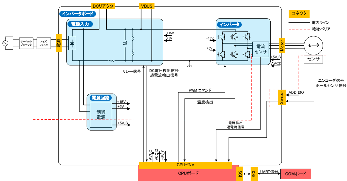
図 2-1 MCI-HV-2-1PH 機能ブロック図
