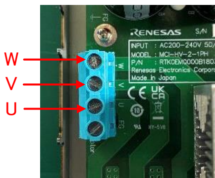
図 3-6 モータの接続
