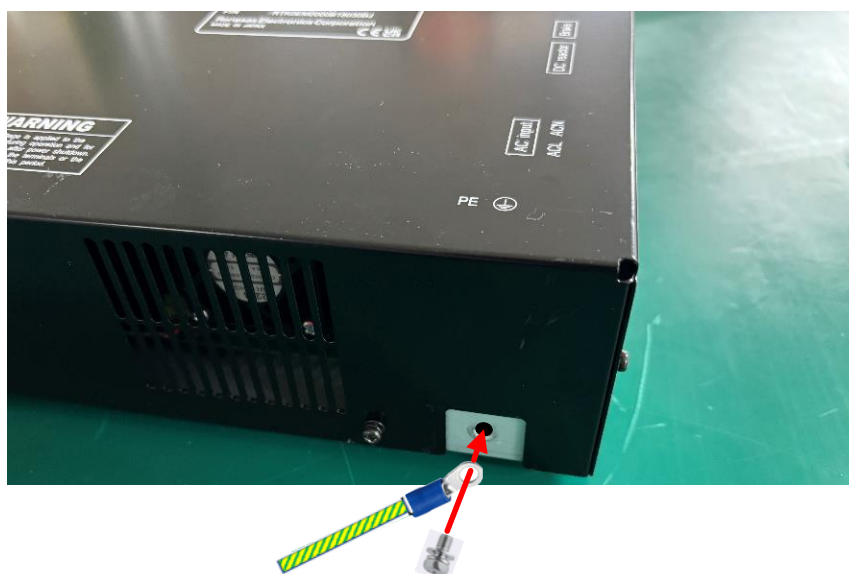
図 3-8 PE の接続
