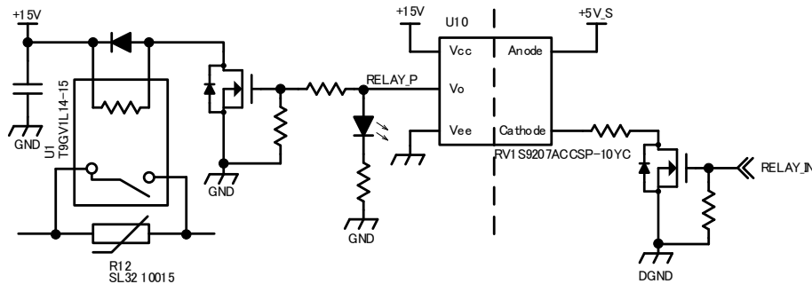
図 4-3 突入電流保護回路
