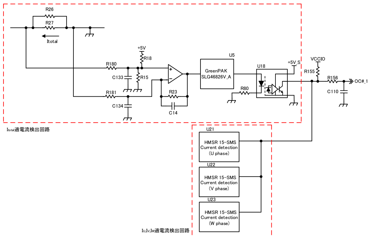
図 4-5 過電流保護
