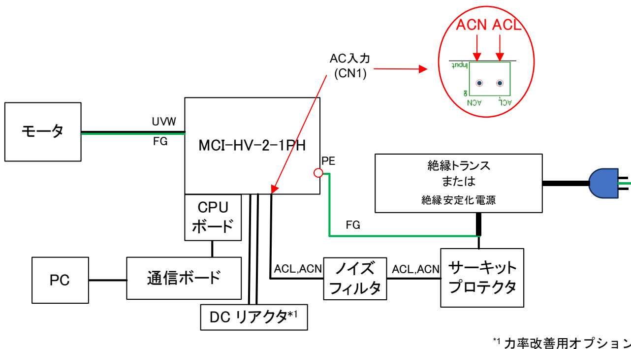
図 3-10 AC 電源接続
