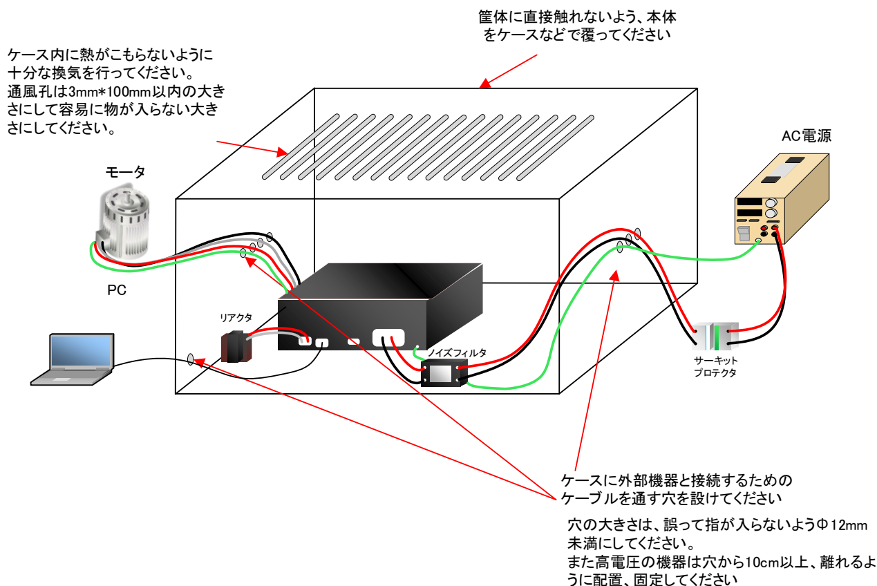
図 3-12 安全操作のためのセットアップ
