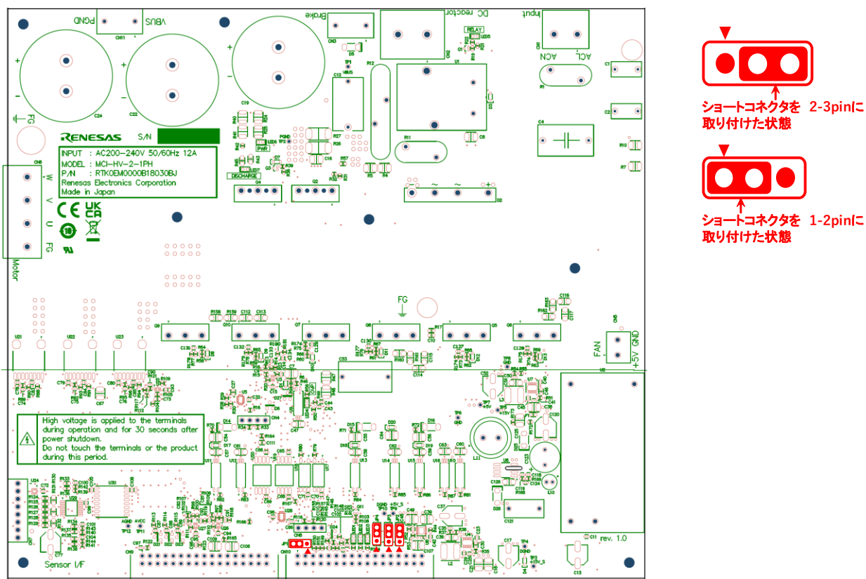
図 2-3 インバータボードジャンパーピンの初期設定
