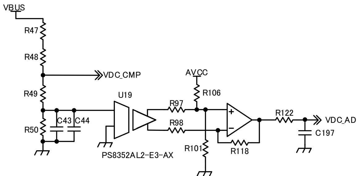
図 4-1 バス電圧検出回路
