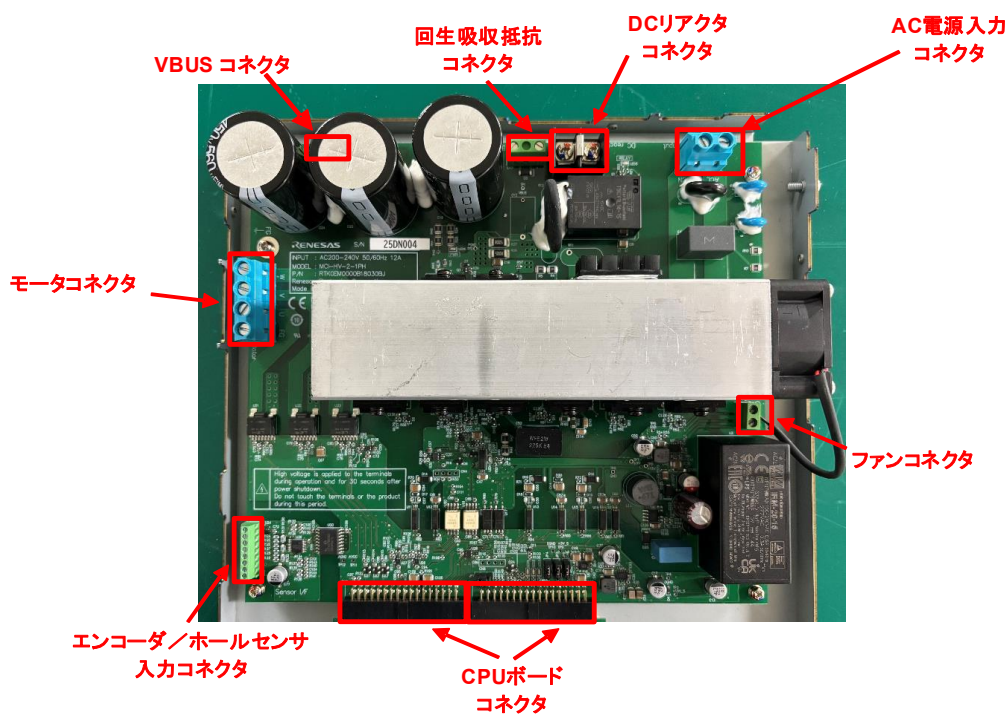
図 2-2 ボードレイアウト
