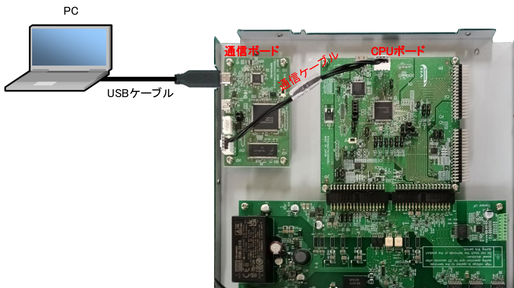
図 3-5 基板の接続 (通信ボード、PC)
