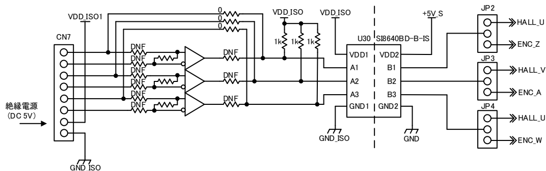
図 4-6 センサ I/F 回路
