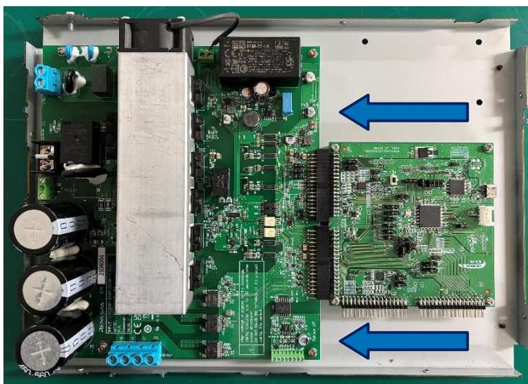
図 3-3 基板の接続 (インバータボード、CPU ボード)
