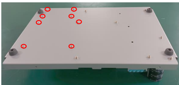
図 3-4 ベースプレートへの取り付け (通信ボード、CPU ボード)
