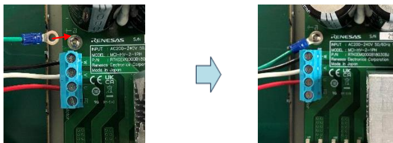
図 3-7 モータ FG の接続
