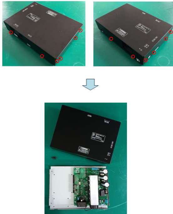
図 3-1 本体カバーの取り外し
