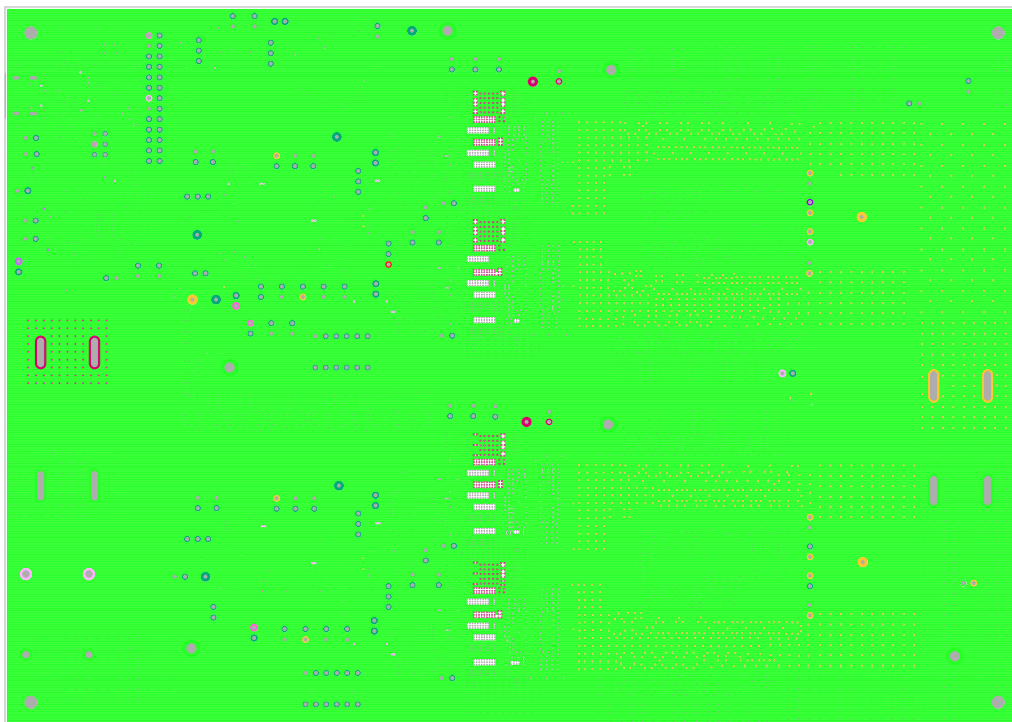
Figure 30. Layer 2
