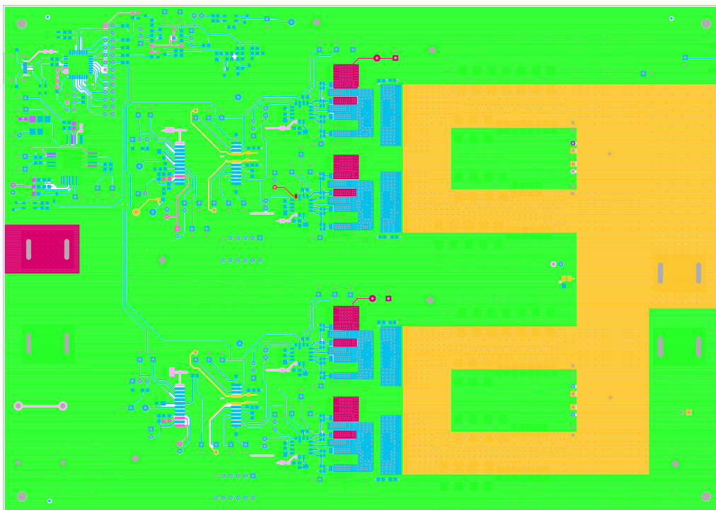
Figure 29. Top Layer
