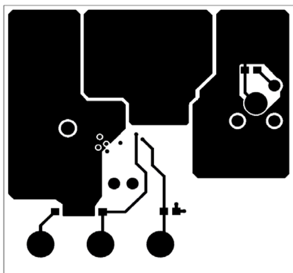
LAYER 4
