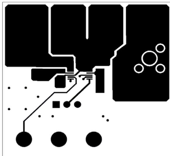
LAYER 1
