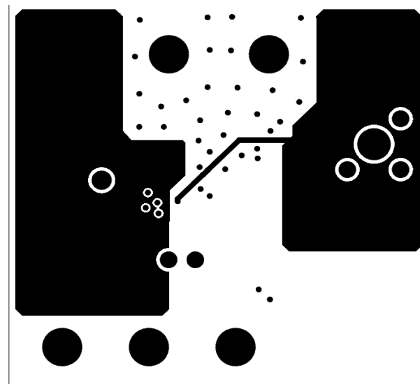
LAYER 3
