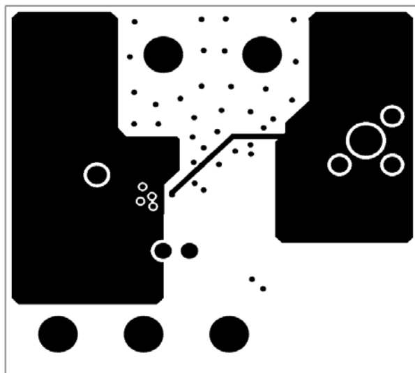
LAYER 3
