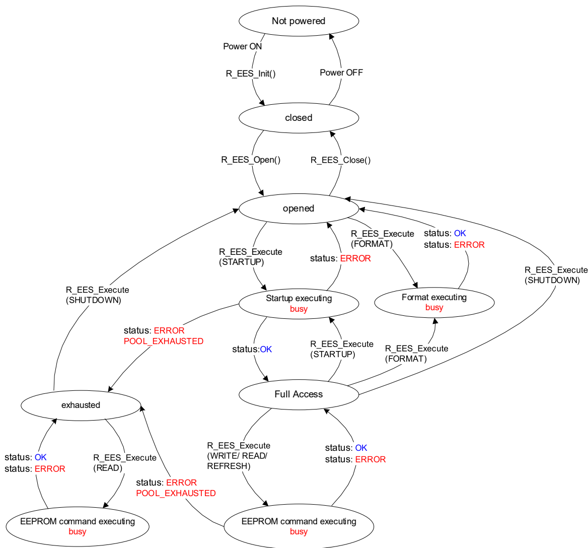
図 5-3 状態遷移図
