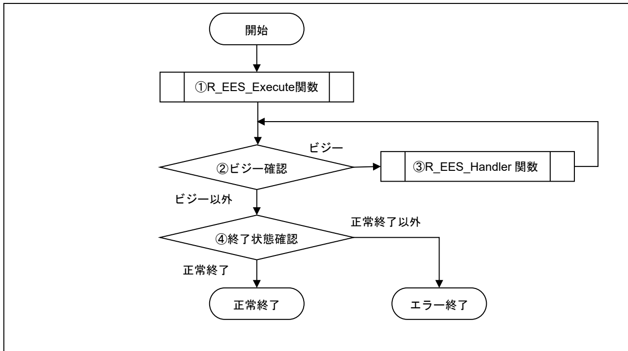
図 5-5 コマンド操作フローチャート
