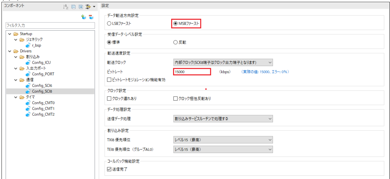
図 4-38 Config_SCI8 設定
