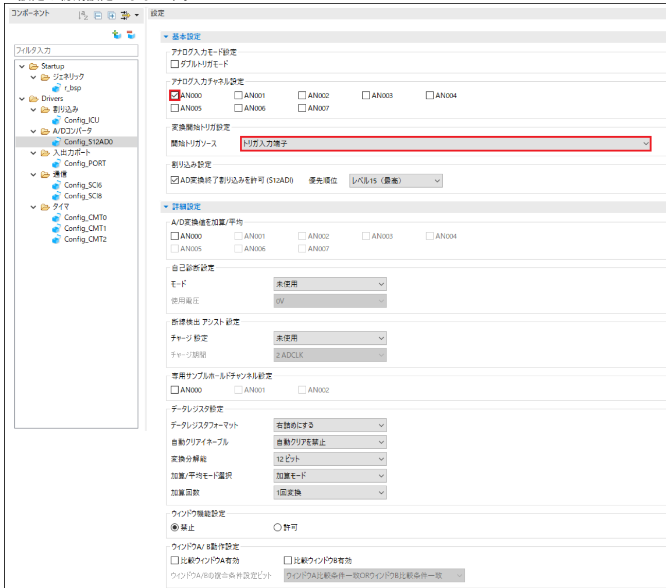
図 4-41 Config_S12AD0 設定(1)
