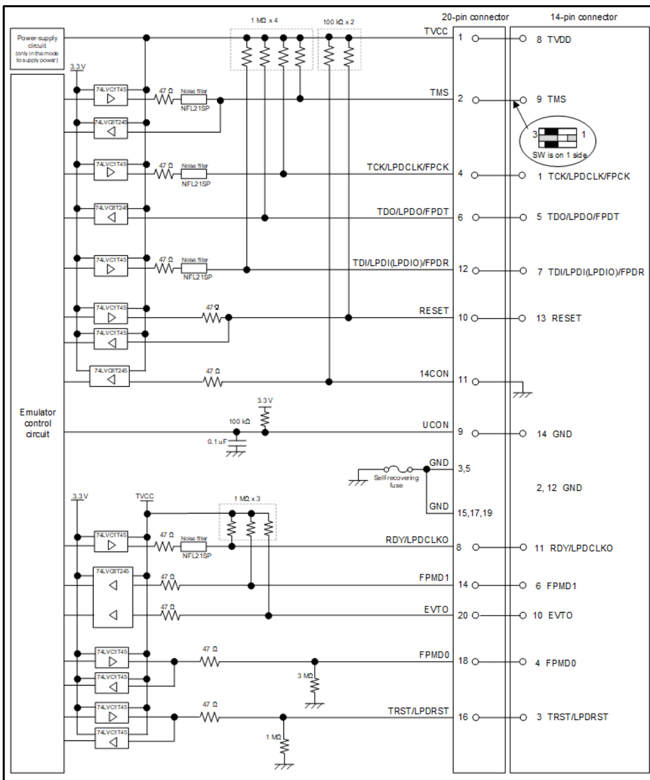
図 6-1 E2 エミュレータ (Rev.C) 内インターフェース回路 (LPD 4pin、JTAG、2wireUART、CSI)
