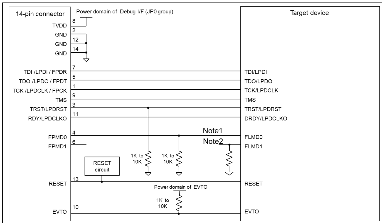
図 2-3 接続例
