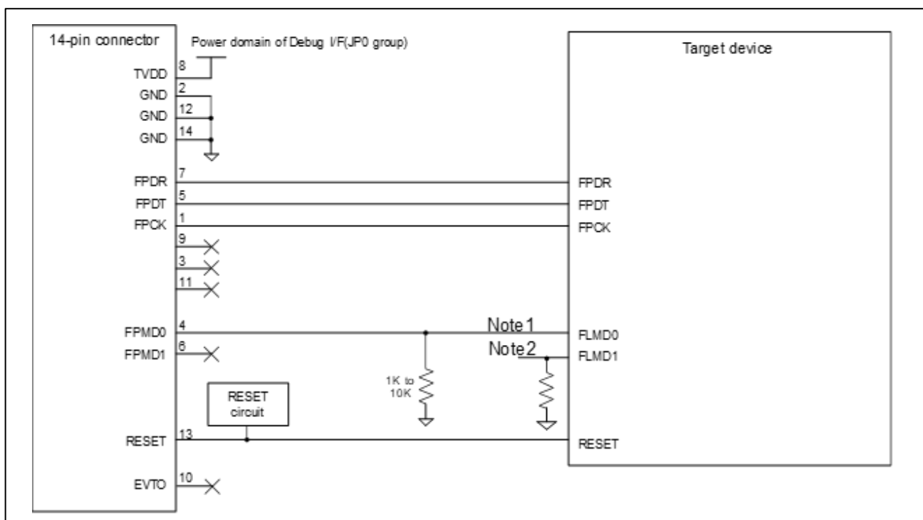
図 2-5 接続例
