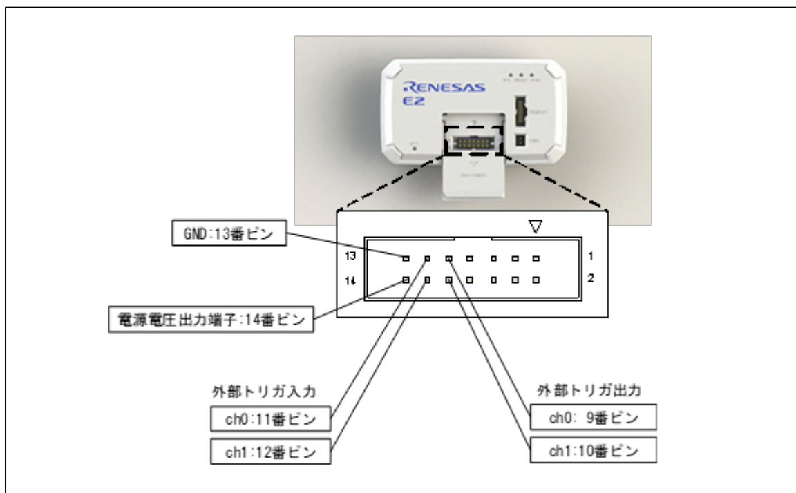
図 2-9 E2 エミュレータ拡張インターフェース
