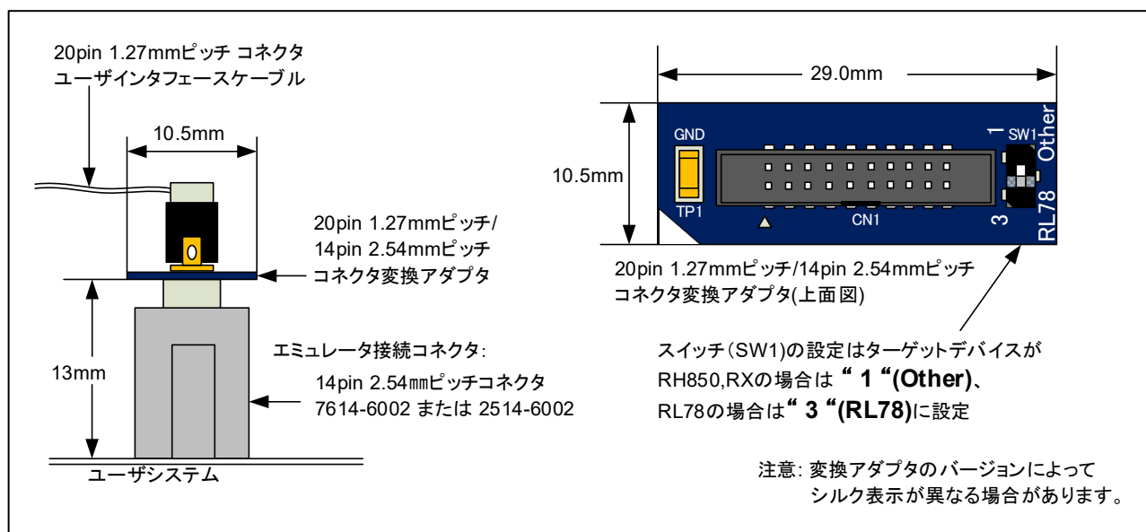
図 2-3 E2 エミュレータでの 14 ピンコネクタへのユーザインタフェースケーブル接続
