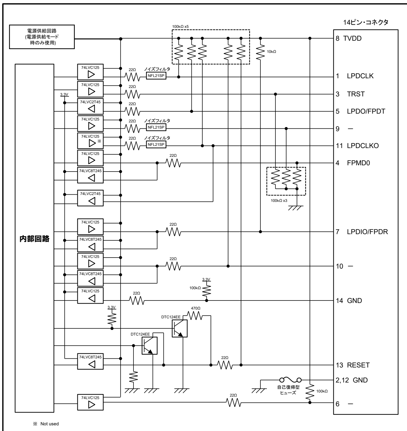
図 5-1 E1/E20 エミュレータ内インタフェース回路(LPД 4pin、2wireUART)
