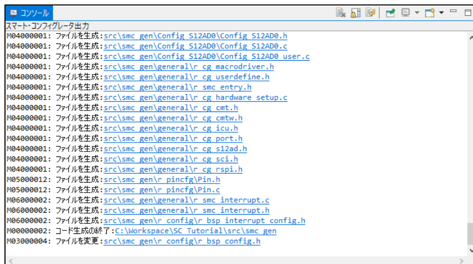
図 4-52 コード生成
